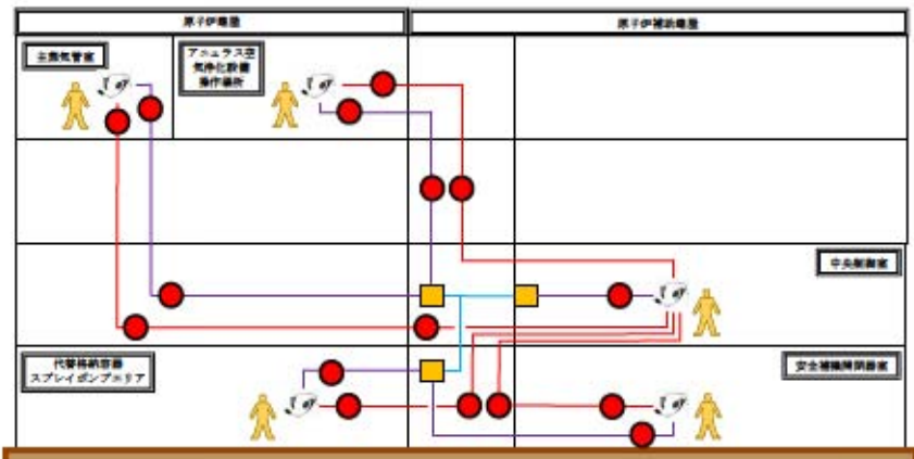
図6 3号炉における中央制御室と現場との通信連絡
