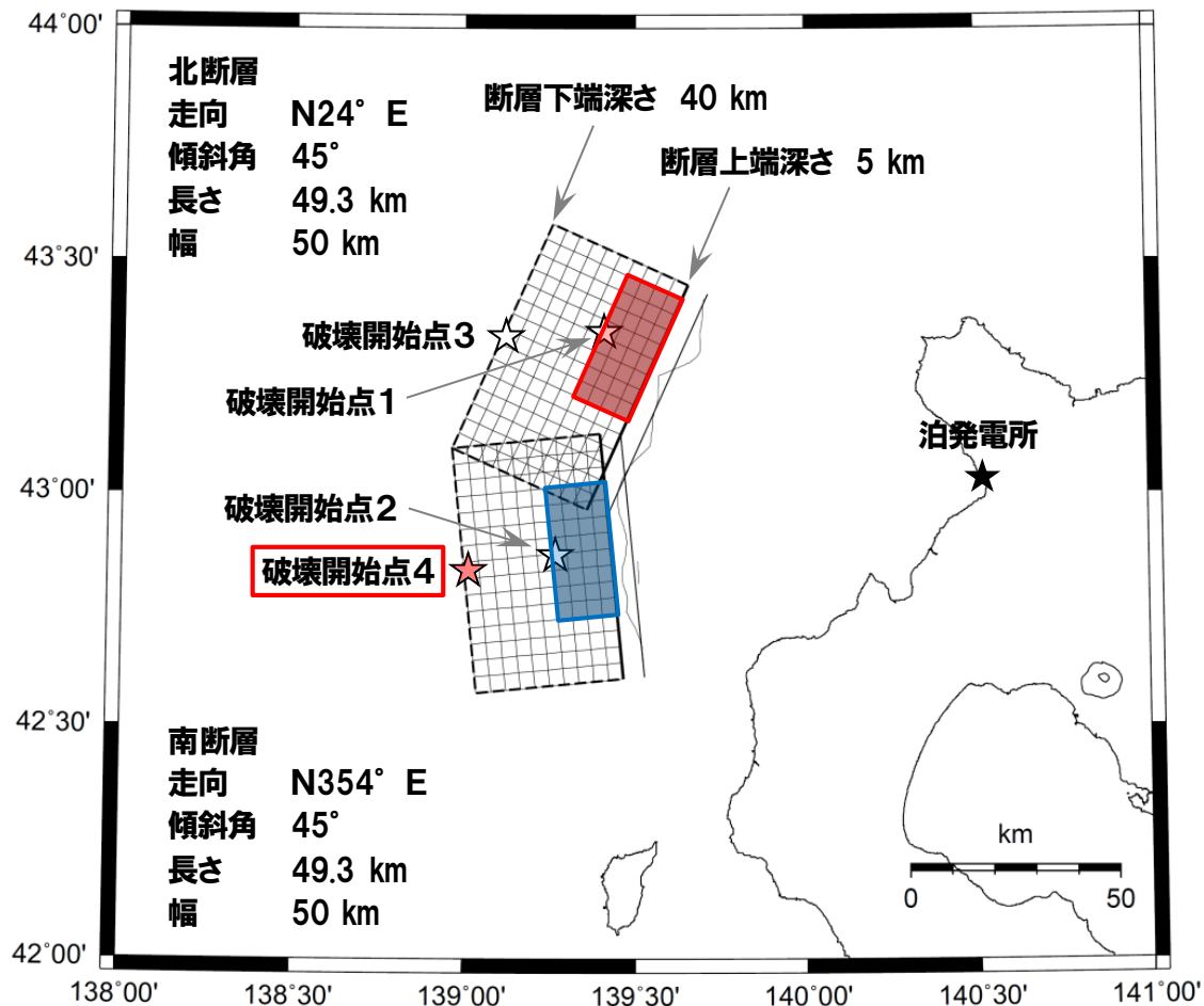
基本震源モデル
