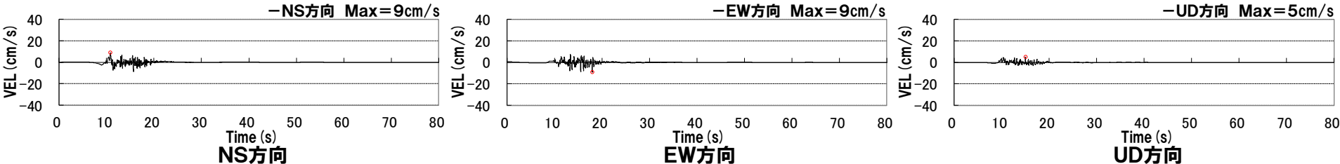
積丹半島北西沖の断層による地震(走向40° ケース, 不確かさ考慮モデル(応力降下量), 破壊開始点4)
