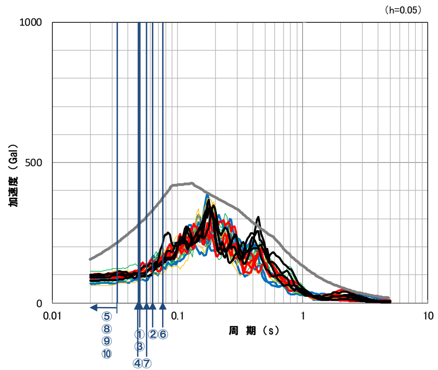
応答スペクトル図(鉛直方向)
