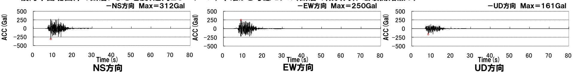
積丹半島北西沖の断層による地震(走向20° ケース, 不確かさ考慮モデル(断層の傾斜角), 破壊開始点2)
