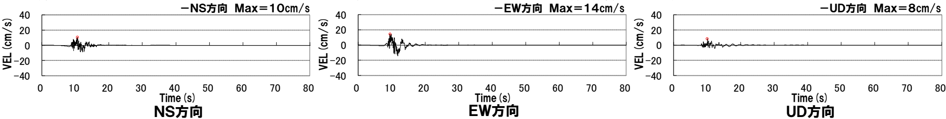
積丹半島北西沖の断層による地震(走向40° ケース, 不確かさ考慮モデル(応力降下量), 破壊開始点2)
