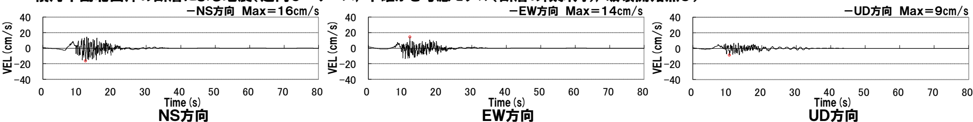
積丹半島北西沖の断層による地震(走向0° ケース, 不確かさ考慮モデル(断層の傾斜角), 破壊開始点4)
