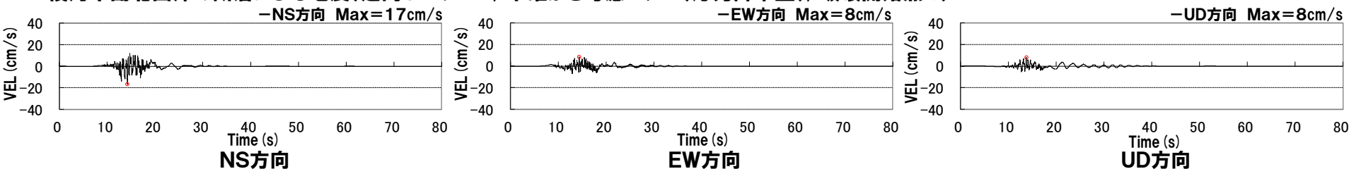
積丹半島北西沖の断層による地震(走向0° ケース, 不確かさ考慮モデル(応力降下量), 破壊開始点4)
