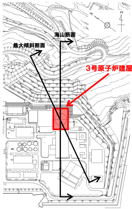
3号炉地盤モデル(断面位置)
