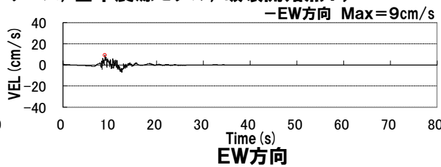
積丹半島北西沖の断層による地震(走向20° ケース, 基本震源モデル, 破壊開始点2)
