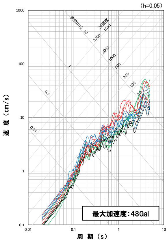
応答スペクトル図(UD方向)
