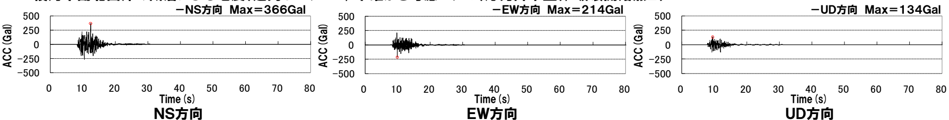
積丹半島北西沖の断層による地震(走向0° ケース, 不確かさ考慮モデル(応力降下量), 破壊開始点3)
