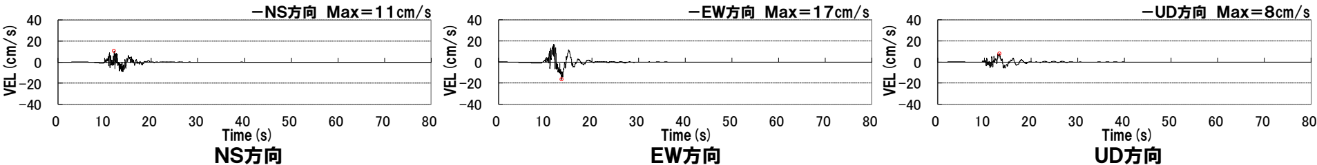
積丹半島北西沖の断層による地震(走向40° ケース, 不確かさ考慮モデル(応力降下量), 破壊開始点3)
