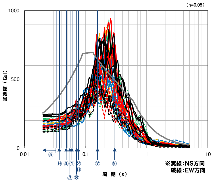
応答スペクトル図(水平方向)
