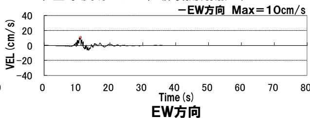
積丹半島北西沖の断層による地震(走向20° ケース, 基本震源モデル, 破壊開始点3)
