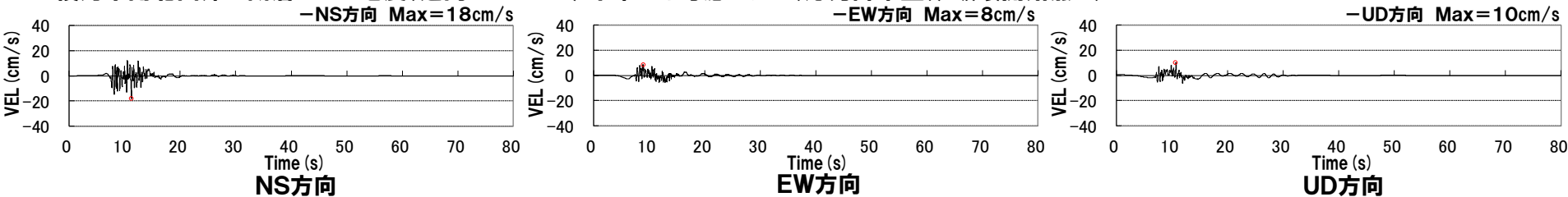
積丹半島北西沖の断層による地震(走向0° ケース, 不確かさ考慮モデル(応力降下量), 破壊開始点2)
