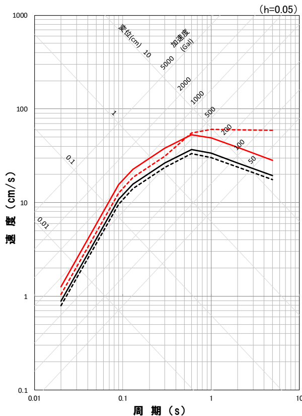
応答スペクトル図(水平方向)
