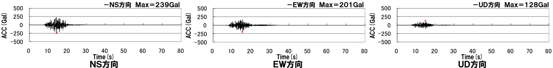
積丹半島北西沖の断層による地震(走向20° ケース, 不確かさ考慮モデル(応力降下量), 破壊開始点4)
