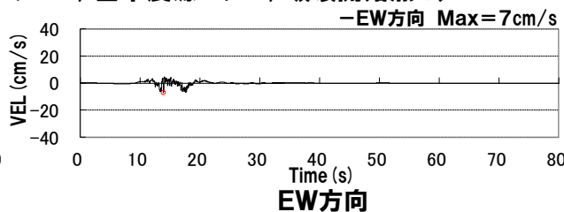
積丹半島北西沖の断層による地震(走向20° ケース, 基本震源モデル, 破壊開始点4)
