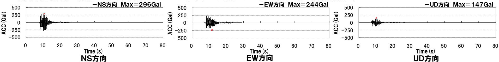
積丹半島北西沖の断層による地震(走向20° ケース, 不確かさ考慮モデル(応力降下量), 破壊開始点2)
