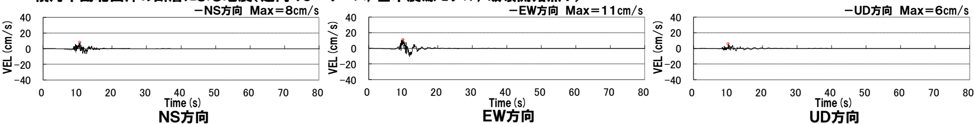
積丹半島北西沖の断層による地震(走向40° ケース, 基本震源モデル, 破壊開始点2)
