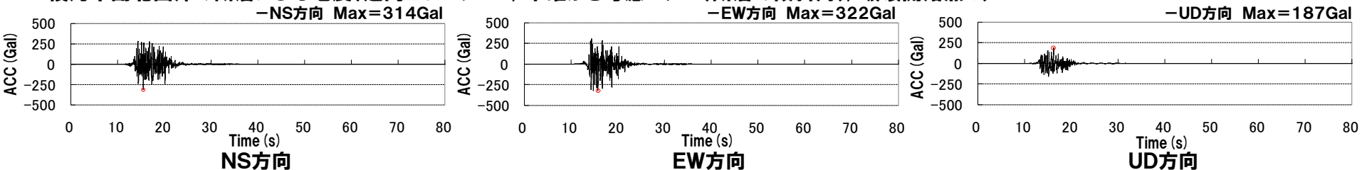
積丹半島北西沖の断層による地震(走向20° ケース, 不確かさ考慮モデル(断層の傾斜角), 破壊開始点4)
