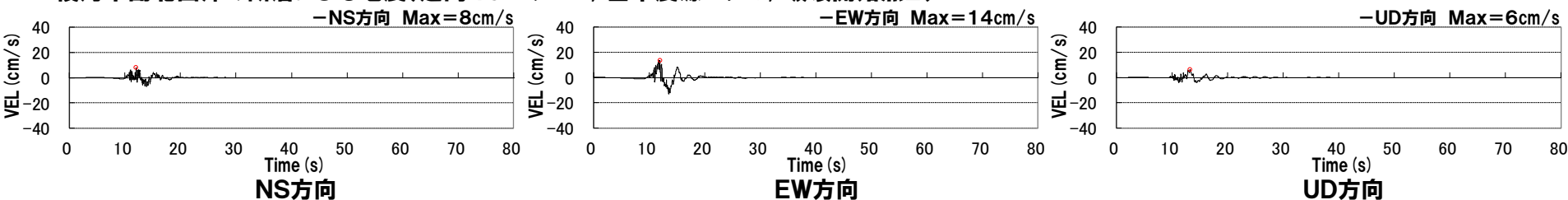
積丹半島北西沖の断層による地震(走向40° ケース, 基本震源モデル, 破壊開始点3)
