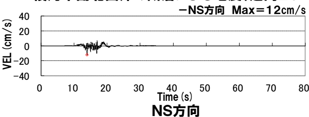
積丹半島北西沖の断層による地震(走向20° ケース, 基本震源モデル, 破壊開始点4)
