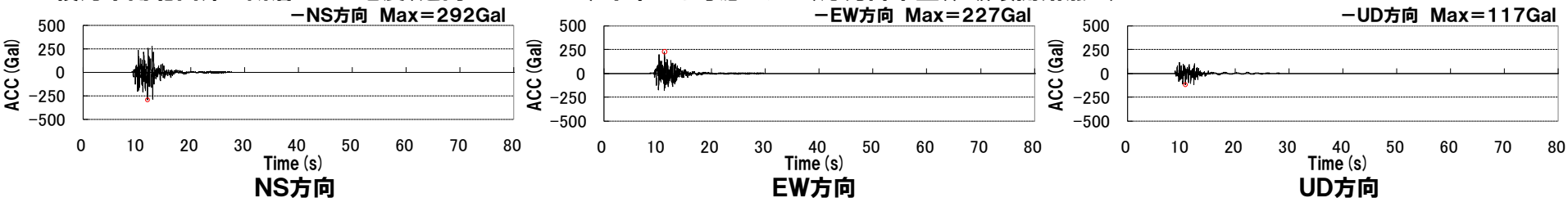
積丹半島北西沖の断層による地震(走向20° ケース, 不確かさ考慮モデル(応力降下量), 破壊開始点3)
