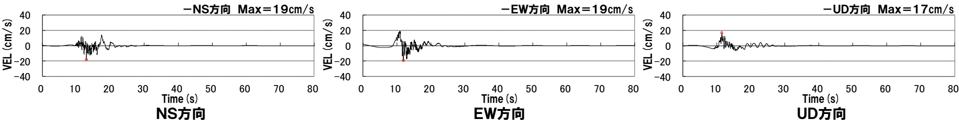
積丹半島北西沖の断層による地震(走向20° ケース, 不確かさ考慮モデル(断層の傾斜角), 破壊開始点3)
