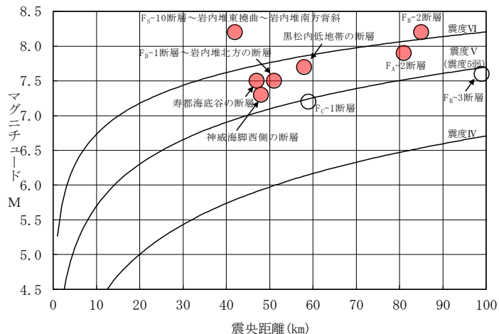
敷地周辺の活断層から想定される地震のマグニチュード-震央距離図
