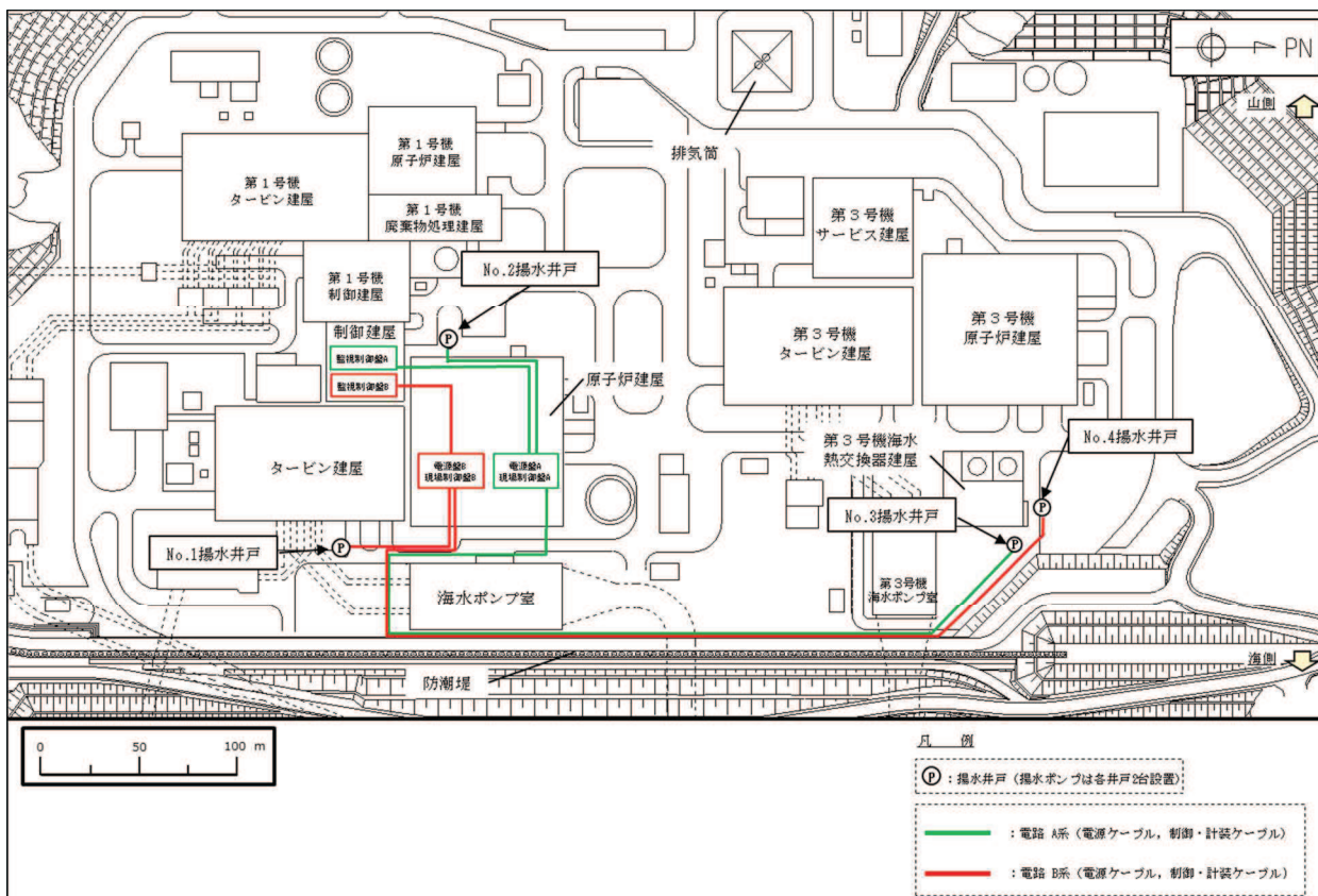
図 6-1 電路の配置
