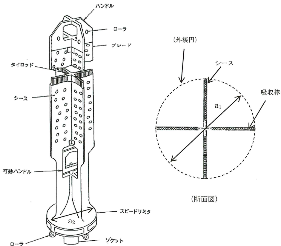
添付 9-5 図 制御棒構造図
