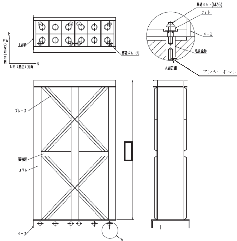
添付 9-6 図 制御棒貯蔵ラック構造図
