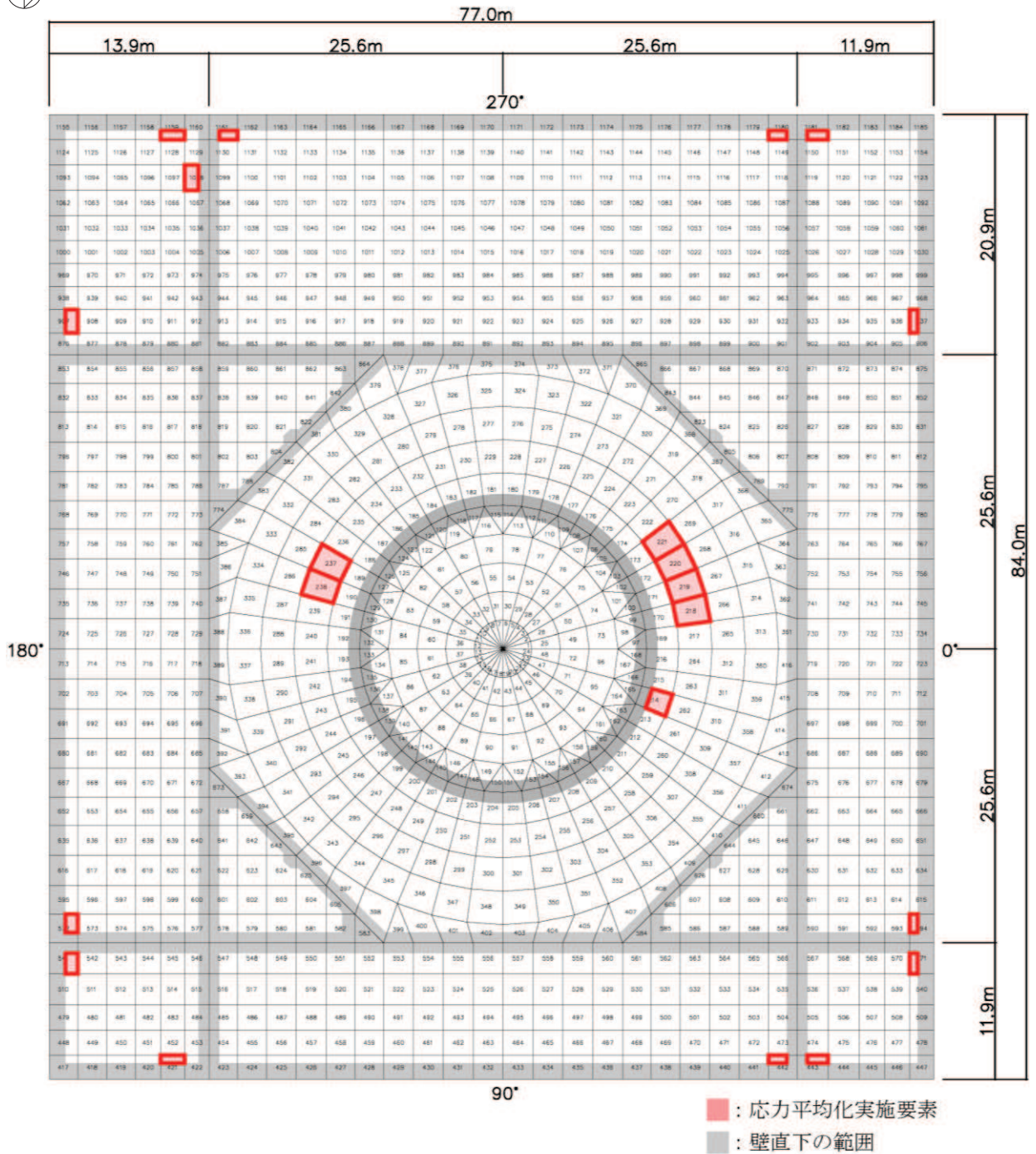
図 2-1 要素位置図
