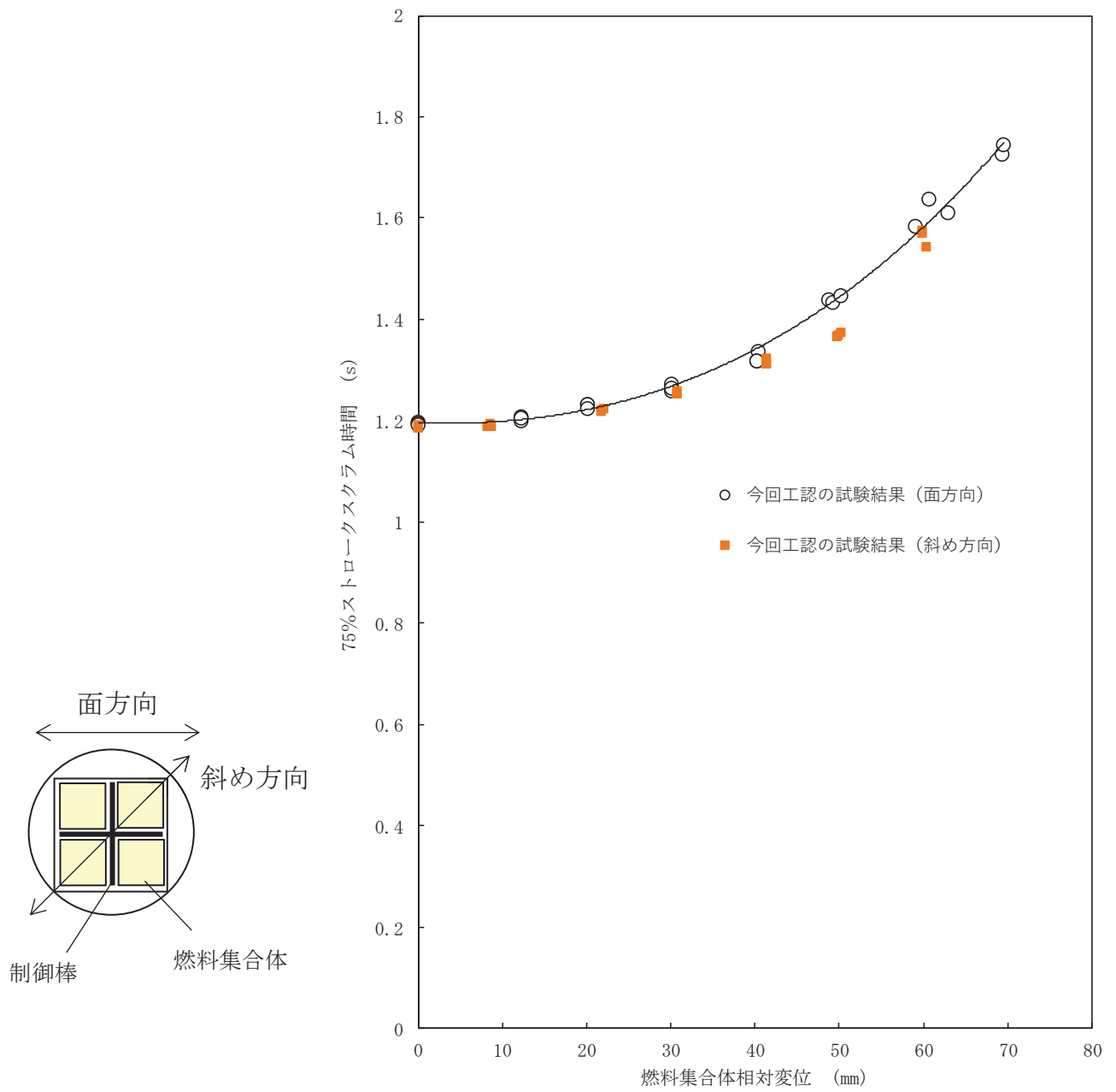
図8 制御棒挿入性試験結果（面方向加振－斜め方向加振の比較）
