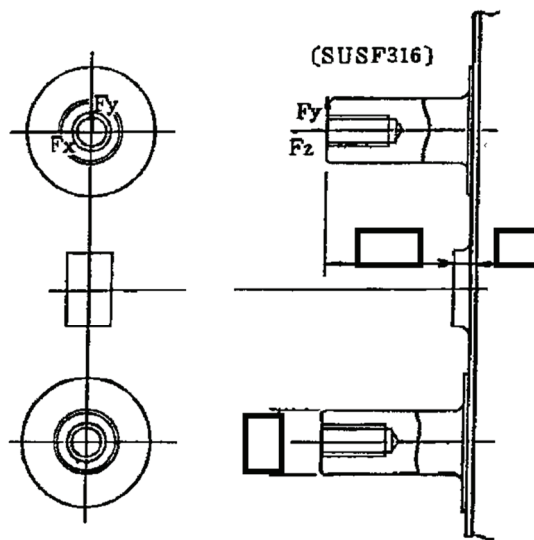
炉心スプレイブラケット (高圧, 低圧)
