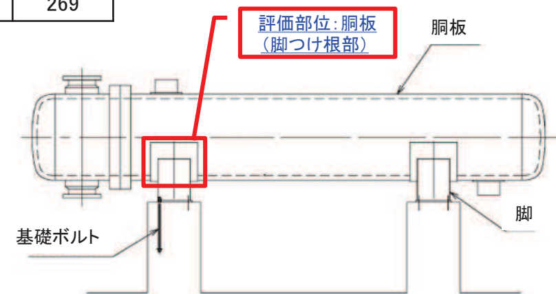
残留熱除去系熱交換器 概略構造図
