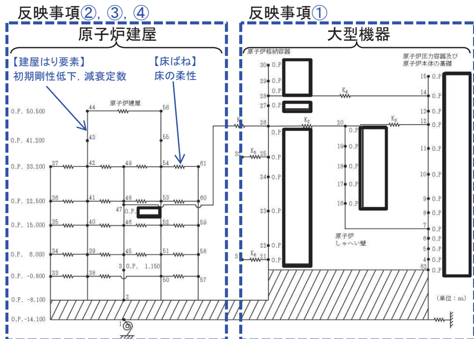
大型機器系(NS方向。その他のモデルは別紙4参照)
