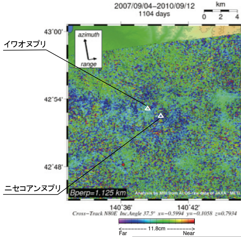
ニセコ・雷電火山群周辺における干渉SAR解析結果 (安藤(2013)に加筆)
