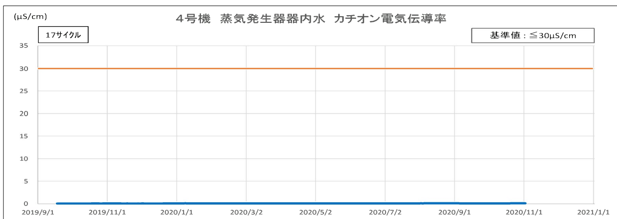
第 2.2.1.2.13 図 水質データの推移 ( 2 / 2 )
