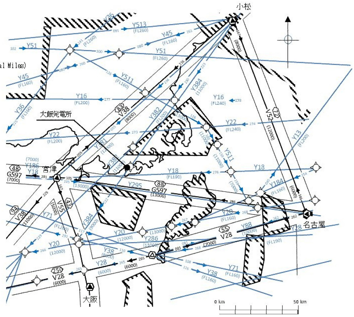
第 1.2.6.4.2 図 発電所周辺の航空路
