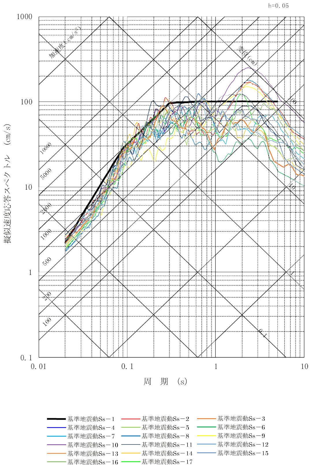
第 1.2.5.6.5 図(2) 基準地震動 Ss-1 と Ss-2~Ss-17 の応答スペクトル (EW 方向)
