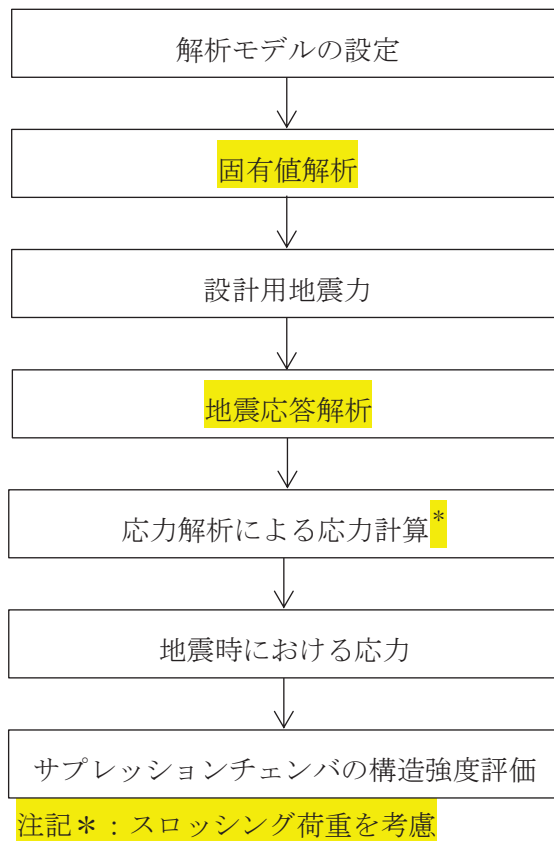
図 2-1 サプレッションチェンバの耐震評価フロー
