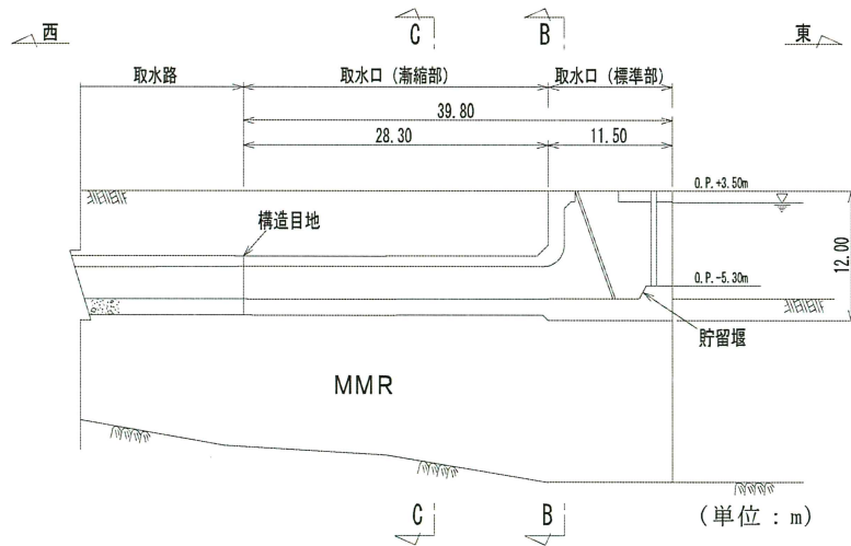
図 3-3-31 取水口，貯留堰縦断面図 (A-A)
