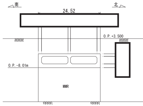
図 3-3-33 取水口断面図 (漸縮部, C-C)
