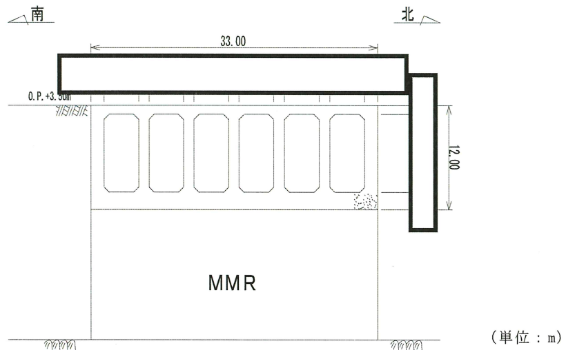
図 3-3-32 取水口断面図 (標準部，B-B)
