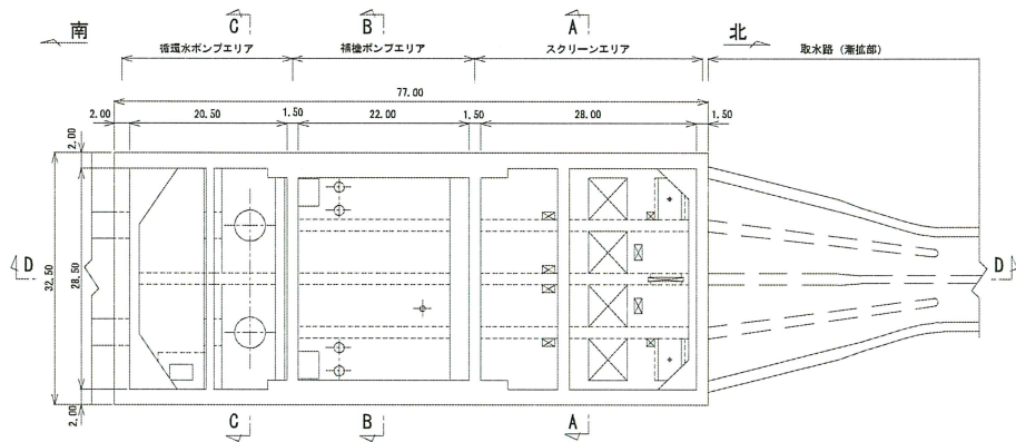
図 3-3-25 海水ポンプ室平面図
