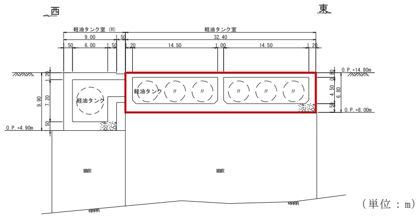
図 3-3-20 軽油タンク室断面図 (B-B, タンク室)
