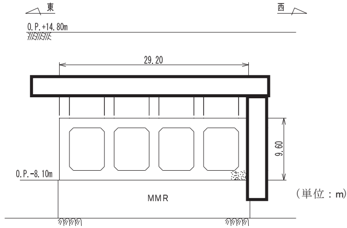
図 3-3-14 取水路（漸拡部）断面図（A-A）
