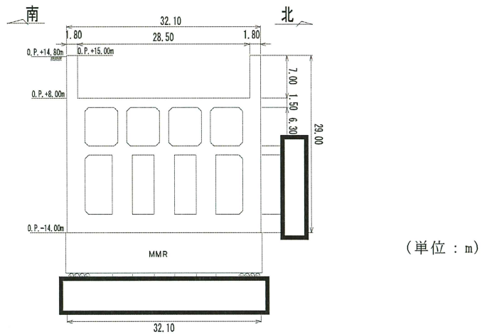
図 3-3-41 第 3 号機海水ポンプ室縦断面図 (A-A)
