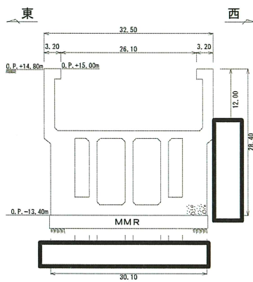
図 3-3-27 海水ポンプ室断面図 (B-B)
