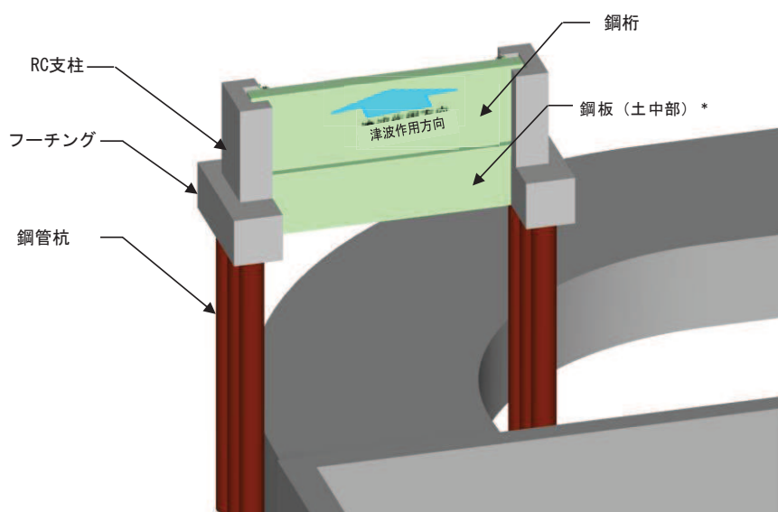
図 3-4-9 鋼製遮水壁（鋼桁） 構造概要図
