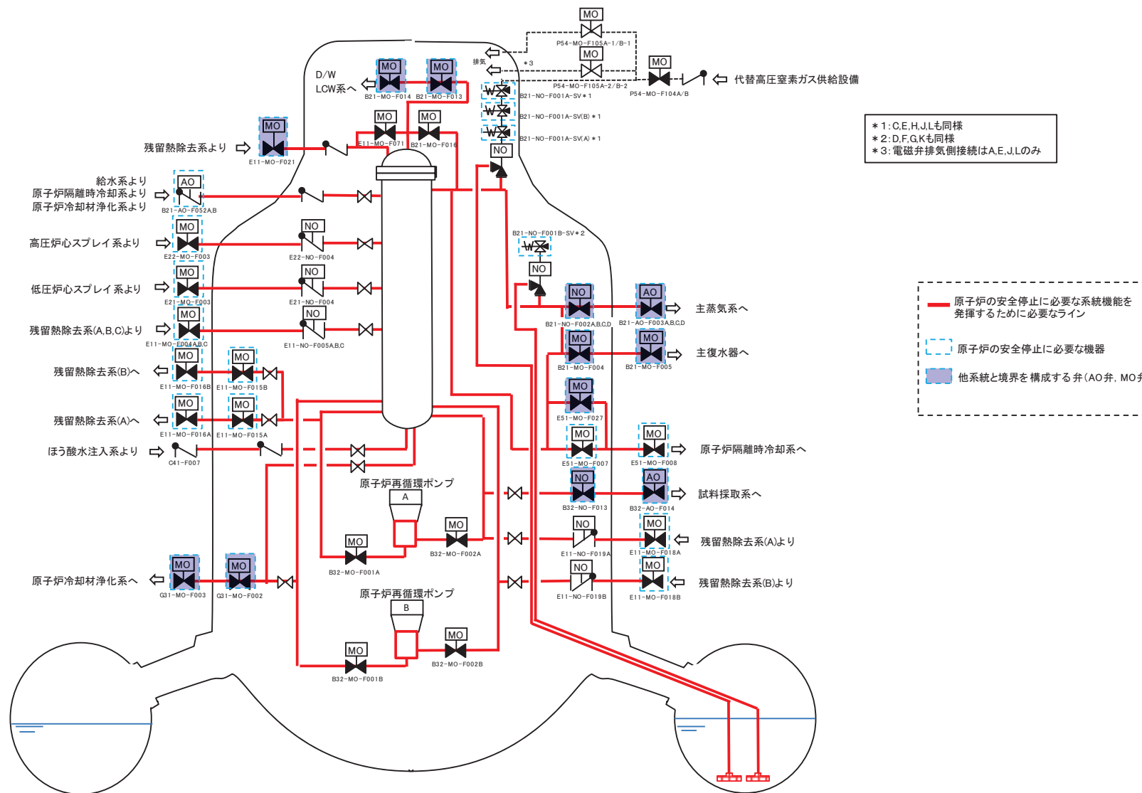
図1 原子炉冷却材圧カバウンダリ／自動減圧系／逃がし安全弁
