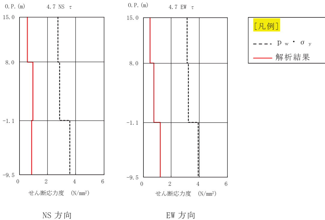
図 2-27 耐震壁のせん断応力度 (4.7 地震)
