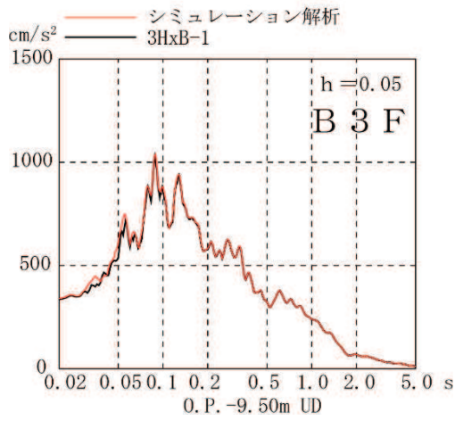
図 2-17 加速度応答スペクトルの比較 (3.11 地震)
