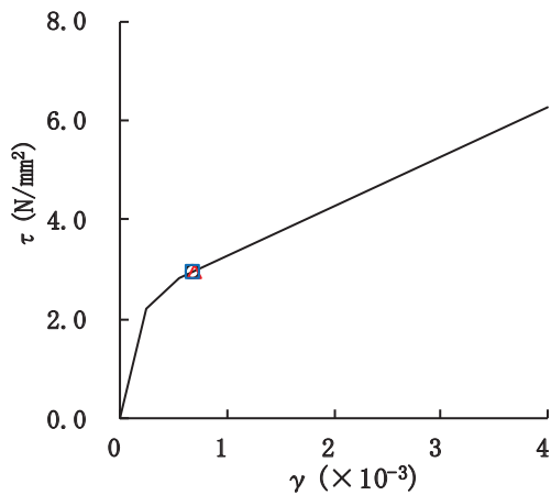
図 2-34 せん断スケルトンカーブ上の最大応答値 (S s - D 3, EW 方向)
