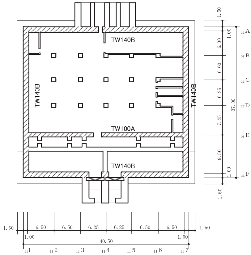
図 2-4 耐震壁配置図 (O.P. -9.5m~O.P. -1.1m)
