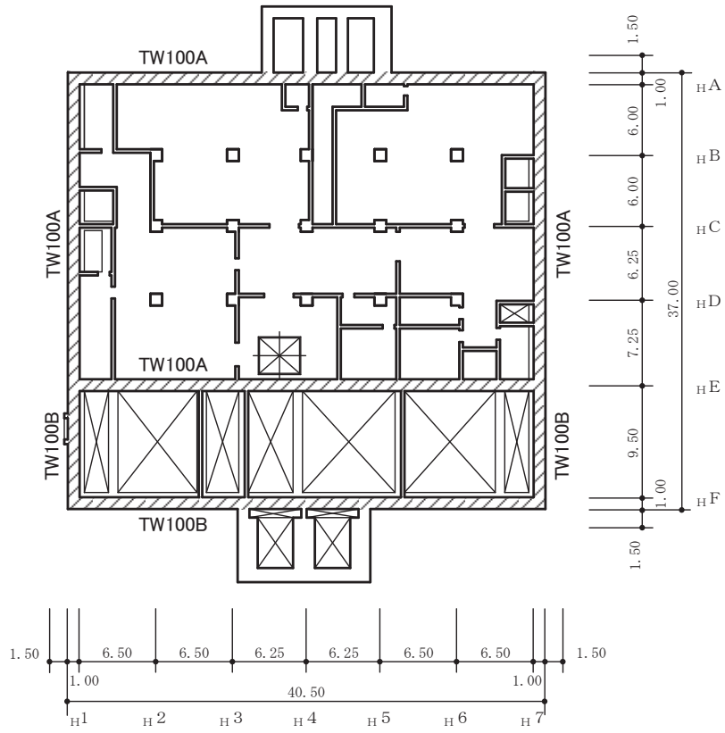
図 2-6 耐震壁配置図 (0. P. 8. 0m~0. P. 15. 0m)
