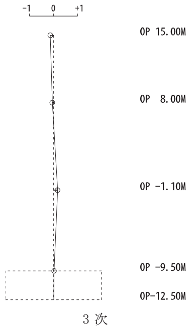
図 4-10 刺激関数図 (ケース 5) (NS 方向 1 次~4 次)
