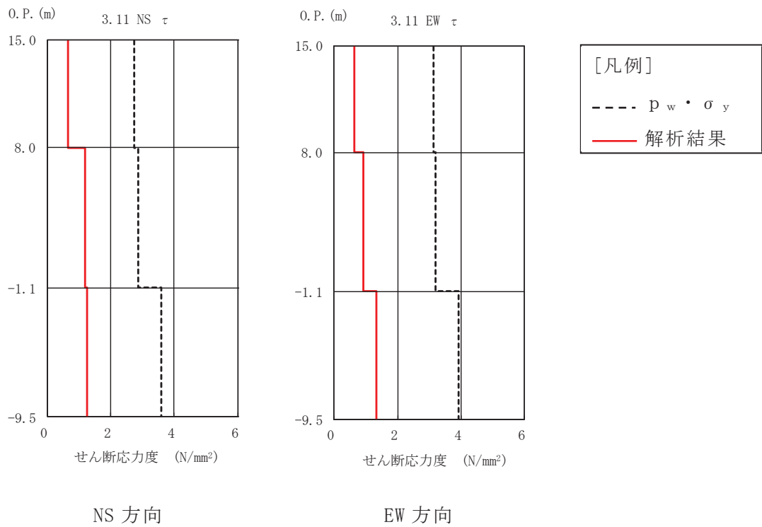
図 2-26 耐震壁のせん断応力度 (3.11 地震)
