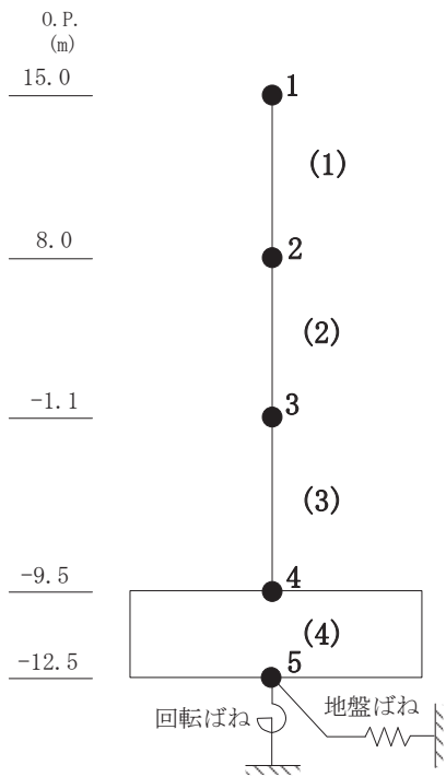
① 誘発上下動を考慮しないモデル
