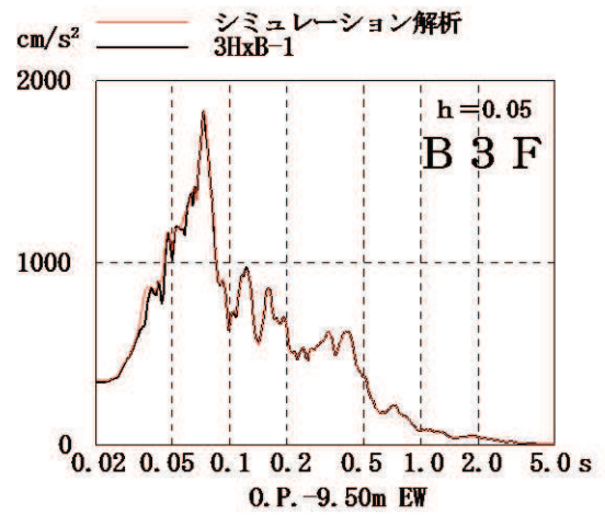
図 2-20 加速度応答スペクトルの比較 (4.7 地震)
