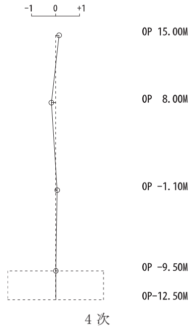
図 4-10 刺激関数図 (ケース 5) (NS 方向 1 次~4 次)
