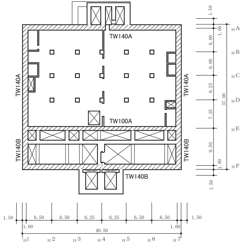
図 2-5 耐震壁配置図 (O.P. -1.1m ~ O.P. 8.0m)
