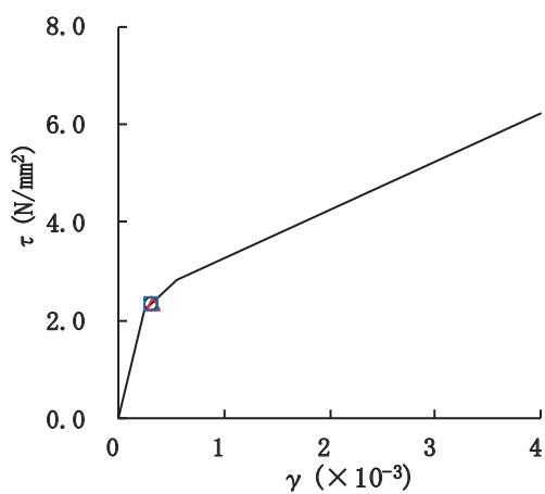
図 2-31 せん断スケルトンカーブ上の最大応答値 (S s - F 3, NS 方向)
