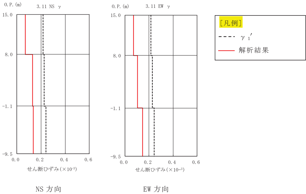
図 2-28 耐震壁のせん断ひずみ (3.11 地震)
