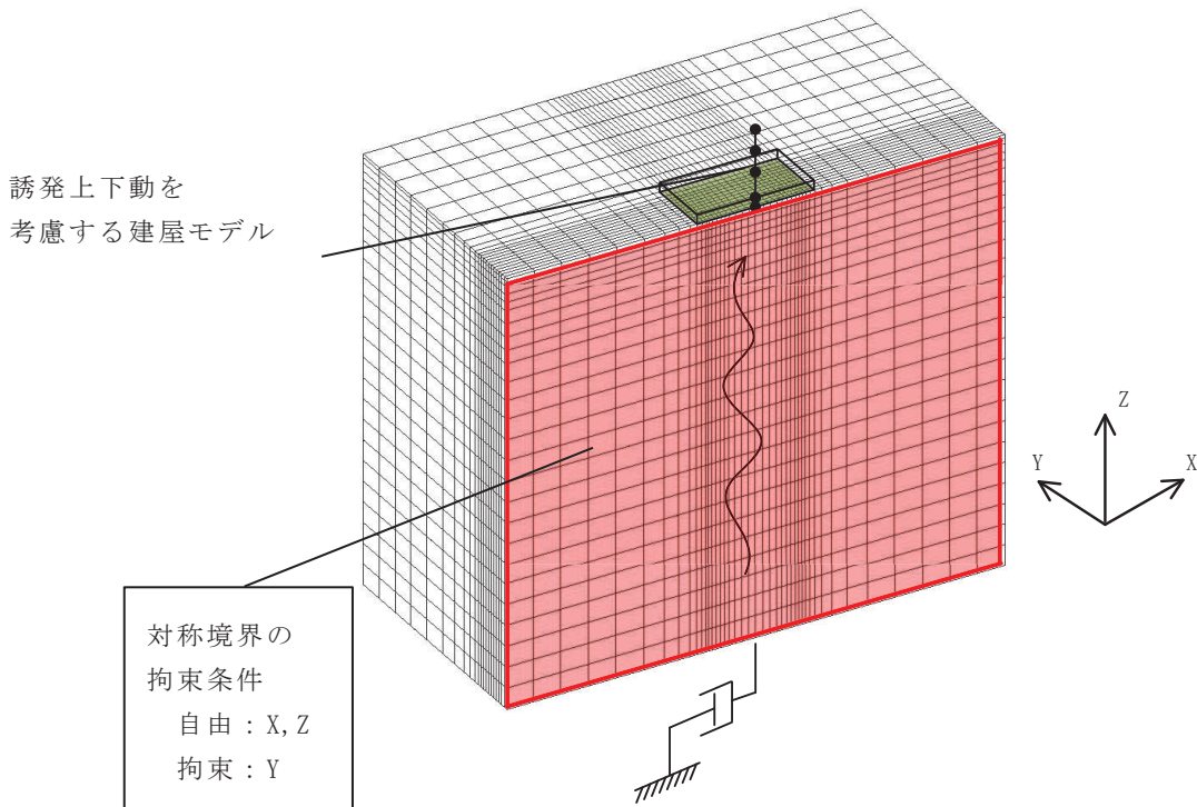
③ 地盤 3 次元 FEM モデル
