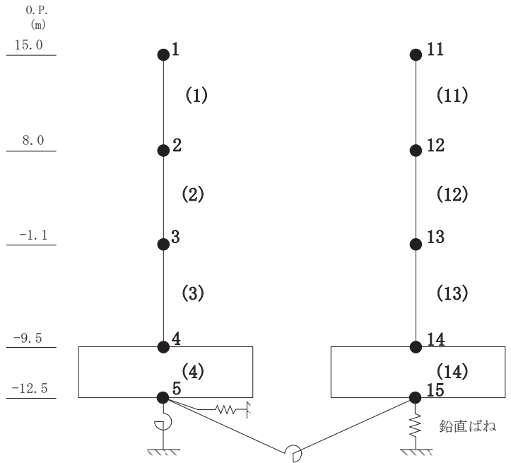
② 誘発上下動を考慮するモデル
