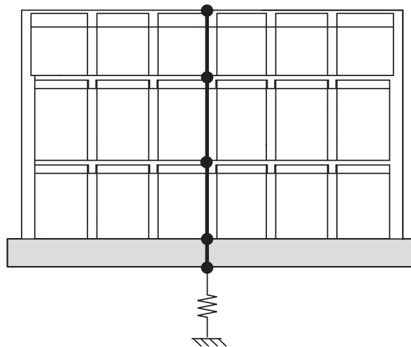
図 2-12 地震応答解析モデル（鉛直方向）
