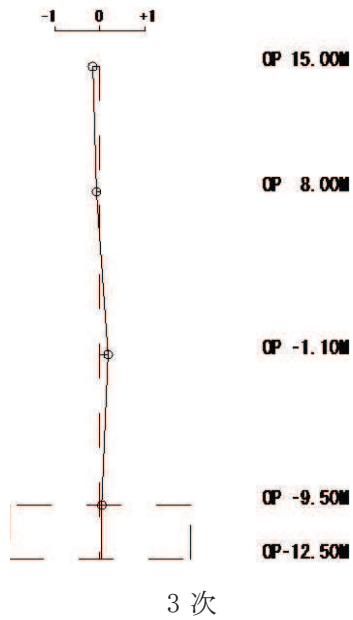
図 2-23 固有振動モード (NS 方向)
