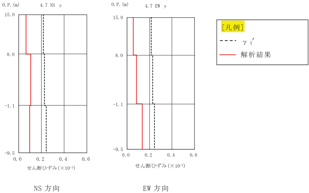
図 2-29 耐震壁のせん断ひずみ (4.7 地震)
