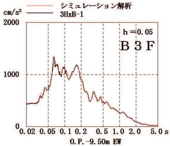
図 2-15 加速度応答スペクトルの比較 (3.11 地震)
