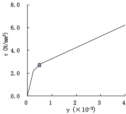
図 2-29 せん断スケルトンカーブ上の最大応答値 (S s - D 2, NS 方向)
