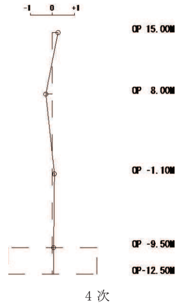
図 2-23 固有振動モード (NS 方向)
