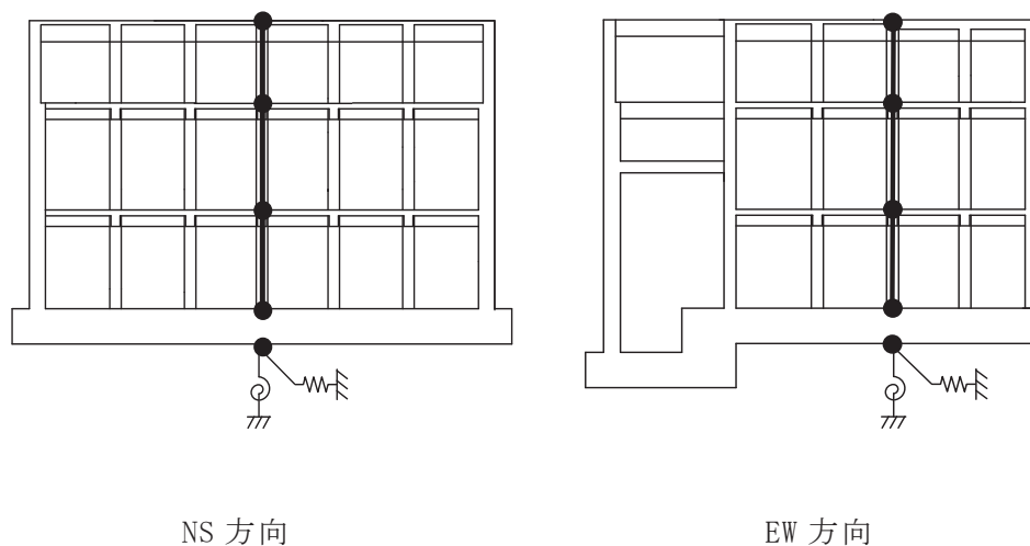
図 2-7 地震応答解析モデル（水平方向）
