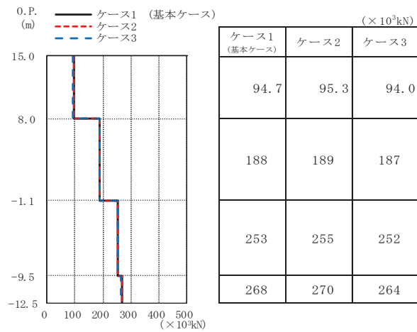
図 2-42 最大応答せん断力 (S d - D 2, EW 方向)
