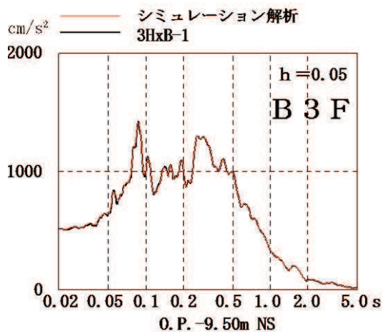
図 2-15 加速度応答スペクトルの比較 (3.11 地震)
