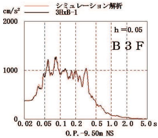
図 2-20 加速度応答スペクトルの比較 (4.7 地震)
