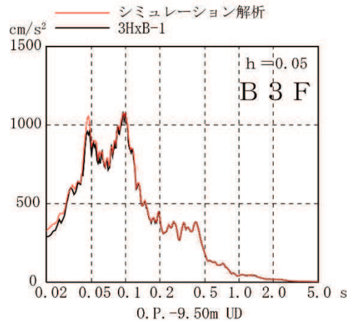
図 2-22 加速度応答スペクトルの比較 (4.7 地震)
