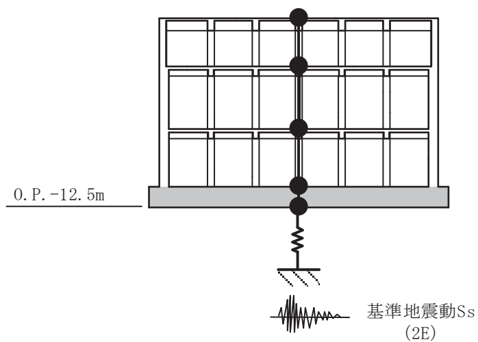
図 3-12 地震応答解析モデルに入力する地震動の概念図（鉛直方向）
