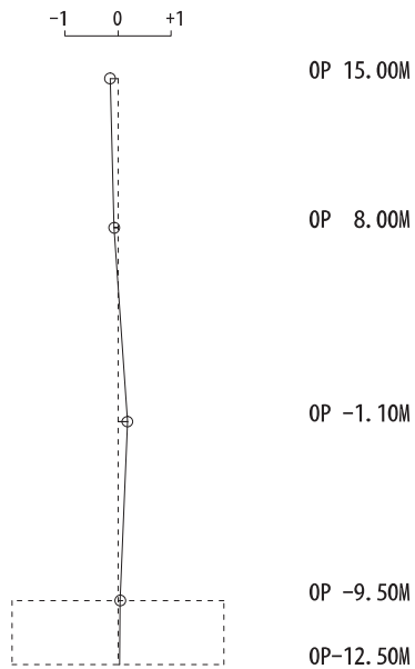
図 4-1(1) 刺激関数図 (NS 方向)
