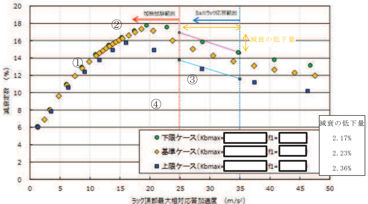
補足図 2-8 締結ボルト剛性 K_{b_{max}} の影響
