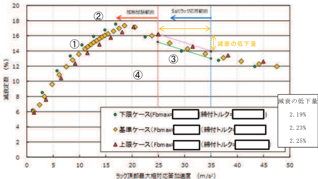
補足図 2-6 ボルト締結面摩擦力 F_{b_{max}} の影響
