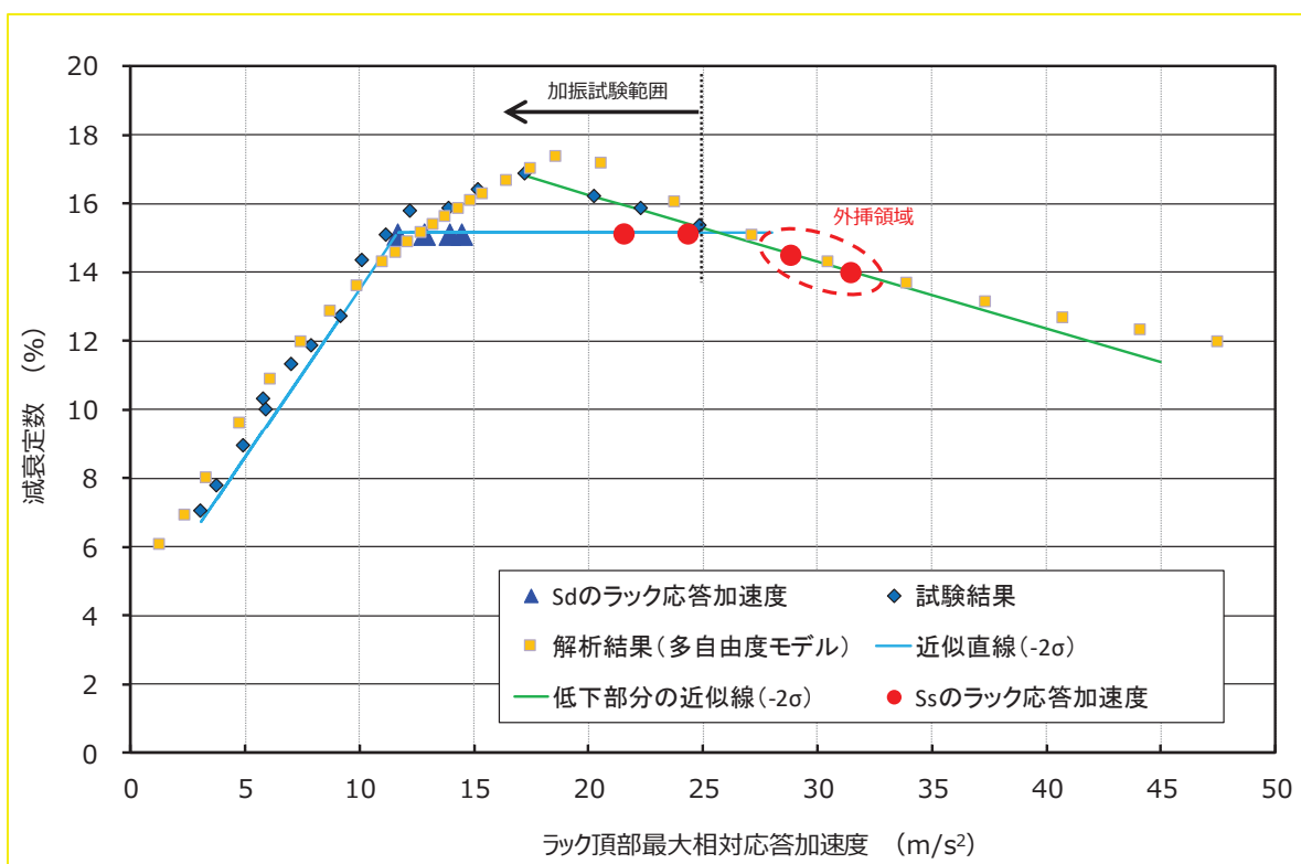
図 12 燃料ラックの減衰挙動に係る解析結果と試験結果 (解析結果の横軸を -3\text{m/s}^2 シフト)
