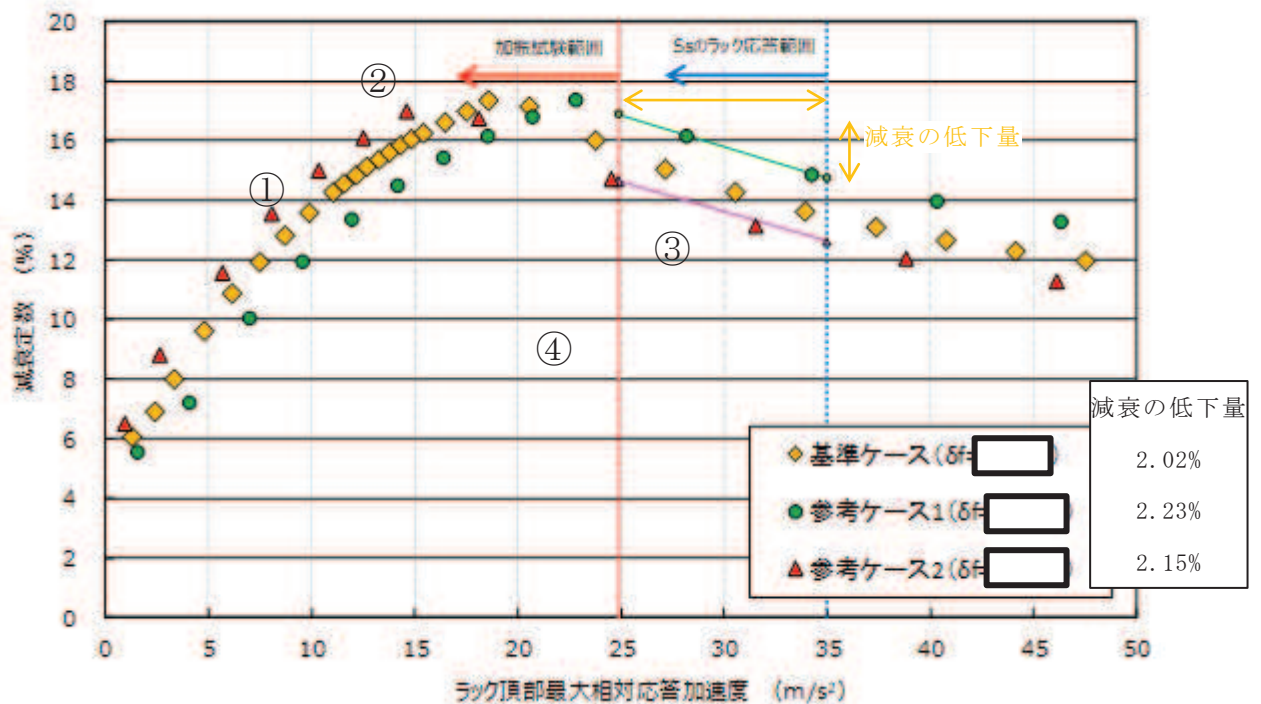
補足図 2-7 摩擦力の振幅依存性を定義する最大変位 \delta f の影響
