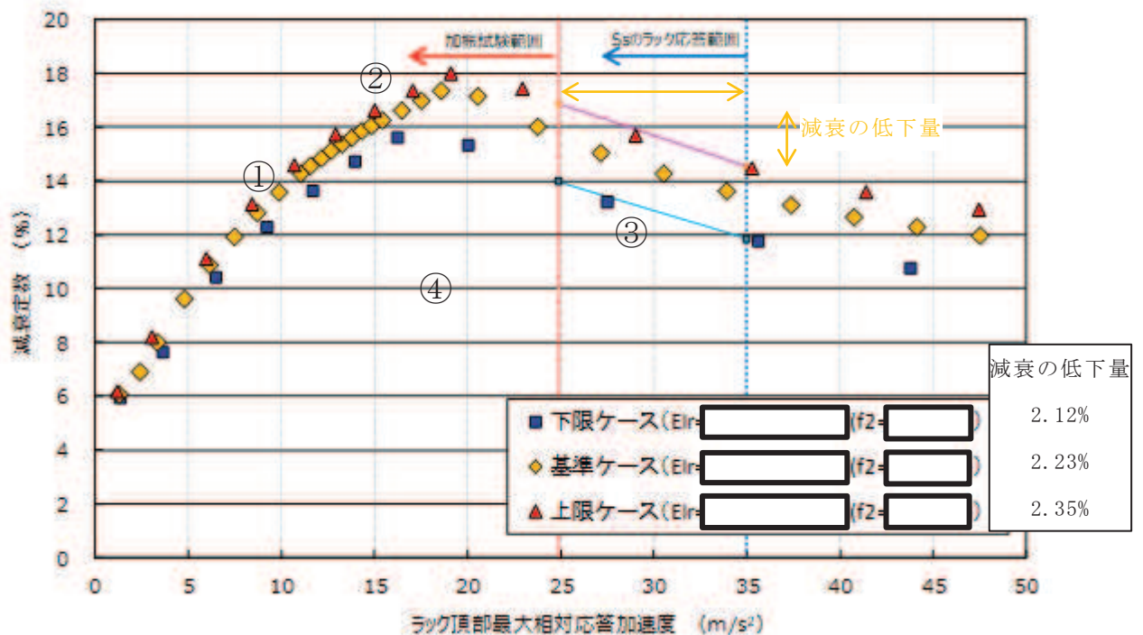
補足図 2-10 燃料ラックの剛性（胴部中央の曲げ剛性） EI_r の影響
