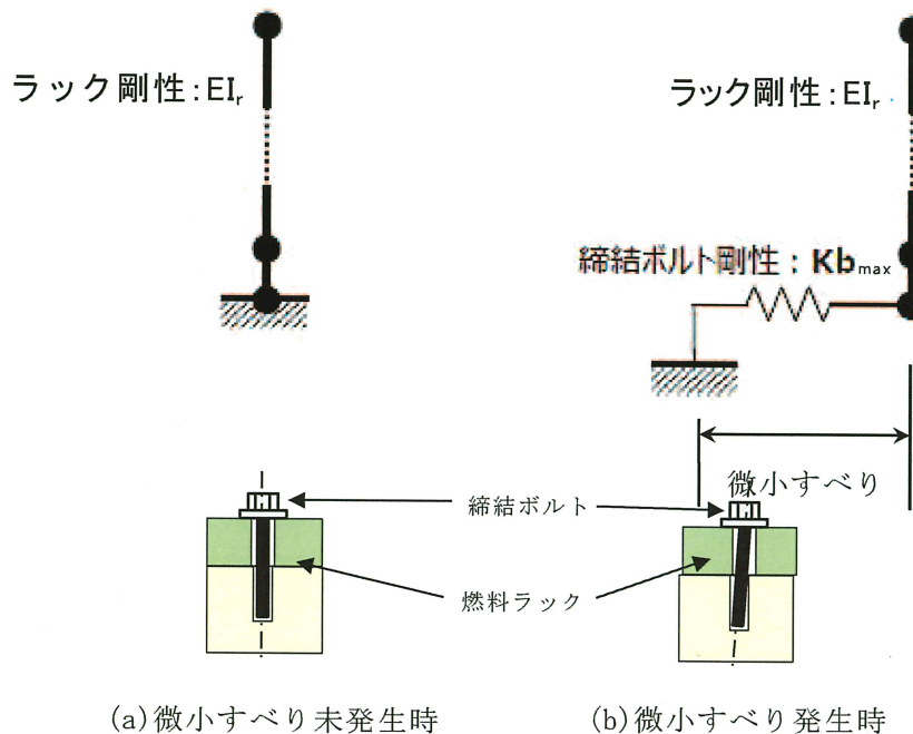
補足図 2-3 締結ボルト及び燃料ラック剛性のモデル化
