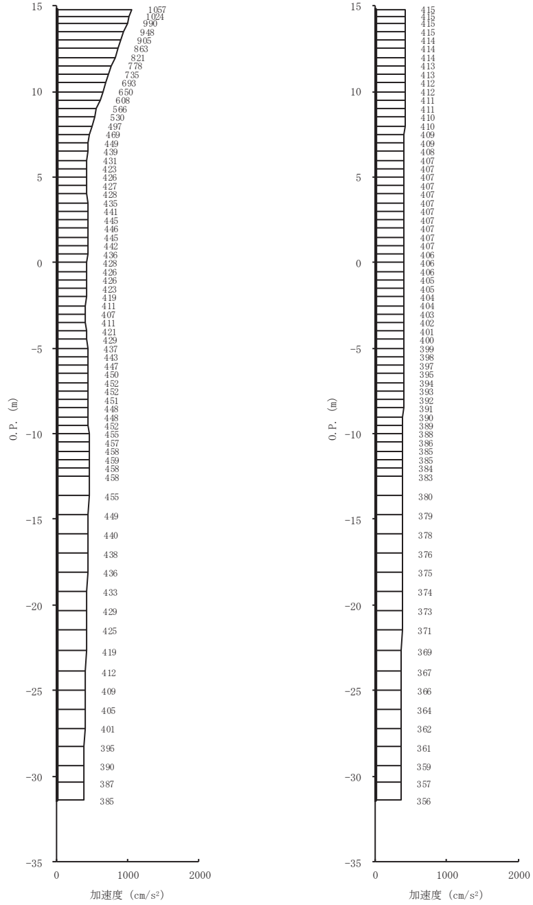
(a) S s - D 1 (-+) 水平 (b) S s - D 1 (-+) 鉛直 図 4-9(8) 最大加速度分布図 (8/14) (No. 3 揚水井戸, 解析ケース⑥)
