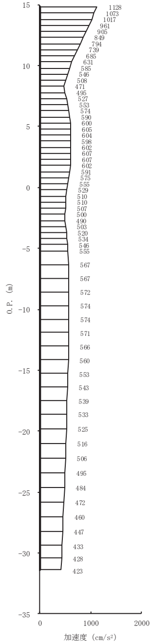
(a) S s - F 1 (++) 水平 (b) S s - F 1 (++) 鉛直 図 4-1(11) 最大加速度分布図 (11/28) (No. 1 揚水井戸, 解析ケース②)
