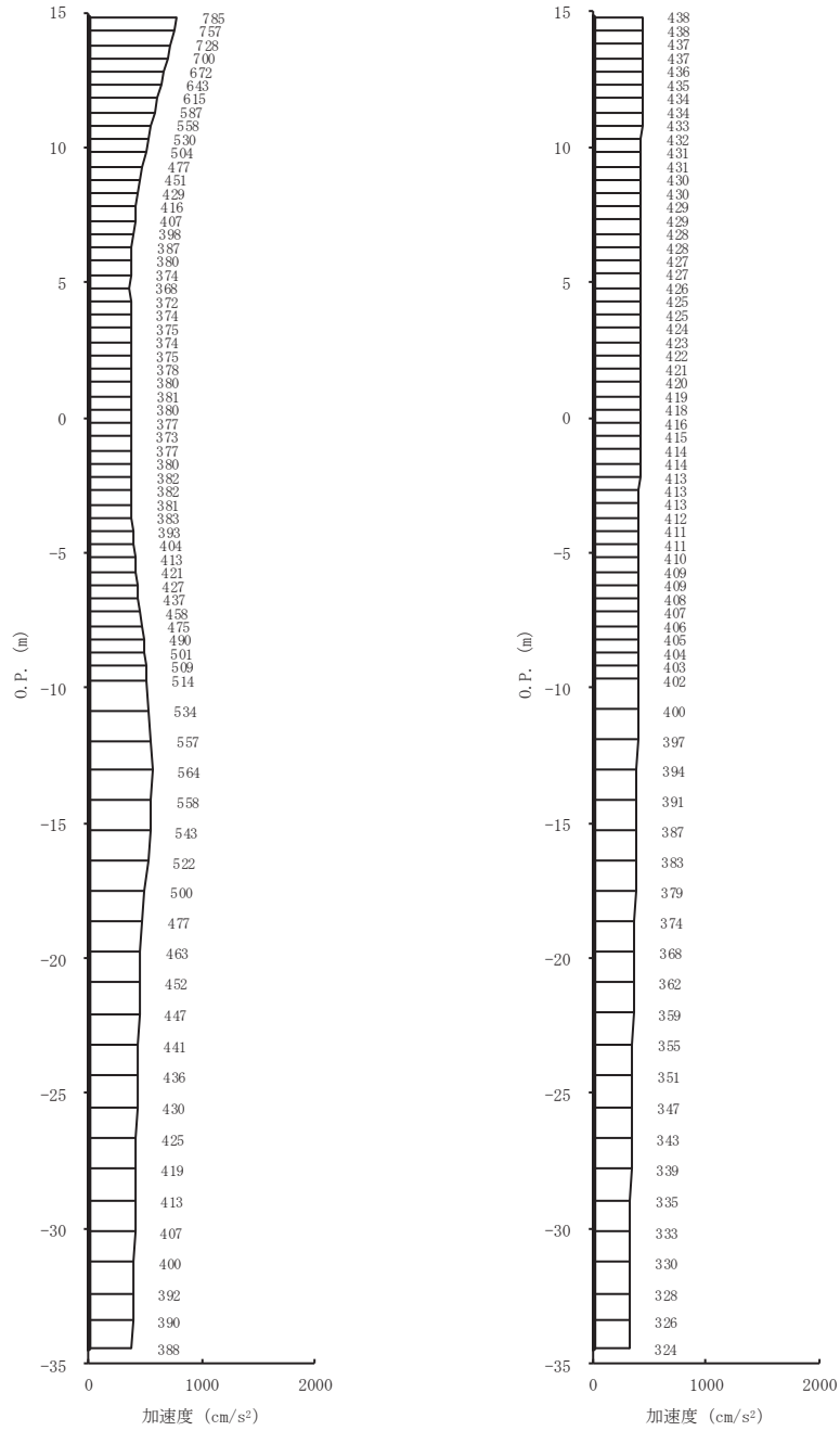
(a) S s - D 2 (++) 水平 (b) S s - D 2 (++) 鉛直 図 4-6(2) 最大加速度分布図 (2/14) (No.2 揚水井戸, 解析ケース⑥)
