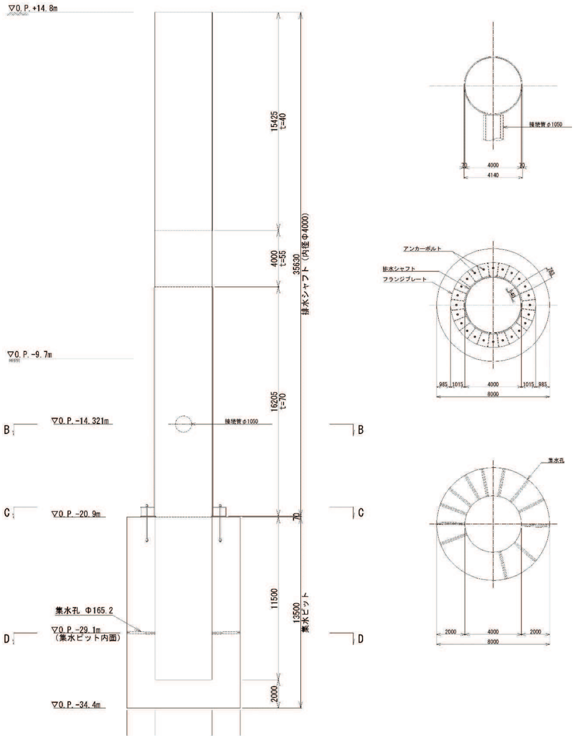
図 2-3(2) No.2 揚水井戸 構造図 (単位 : mm)
