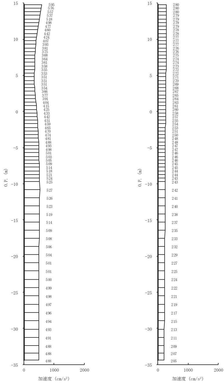
(a) S s - N 1 (-+) 水 (b) S s - N 1 (-+) 鉛直
