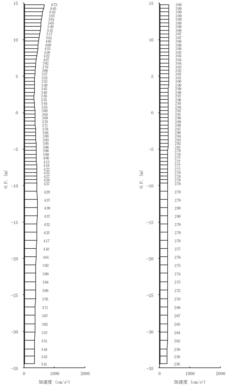
(a) S s - F 1 (++) 水平 (b) S s - F 1 (++) 鉛直 図 4-6(4) 最大加速度分布図 (4/14) (No. 2 揚水井戸, 解析ケース⑥)
