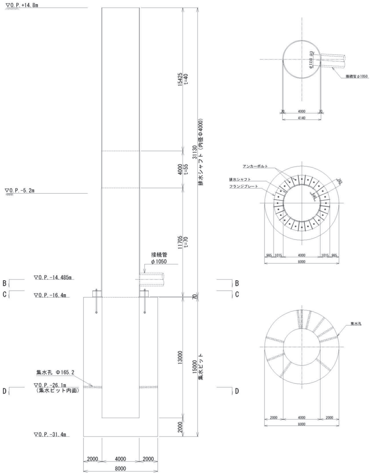
図 2-3(1) No.1 揚水井戸 構造図 (単位: mm)
