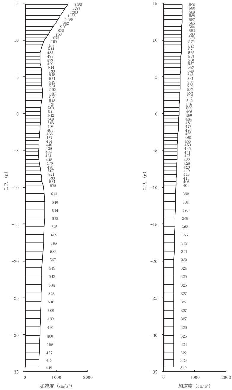
(a) S s - D 3 (++) 水平 (b) S s - D 3 (++) 鉛直
