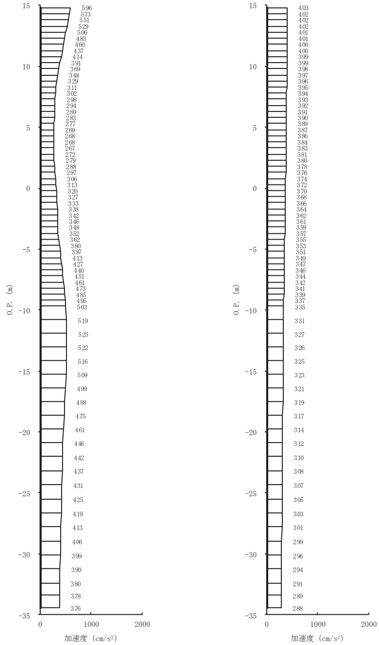
(a) S s - F 3 (++) 水平 (b) S s - F 3 (++) 鉛直 図 4-6(6) 最大加速度分布図 (6/14) (No. 2 揚水井戸, 解析ケース⑥)
