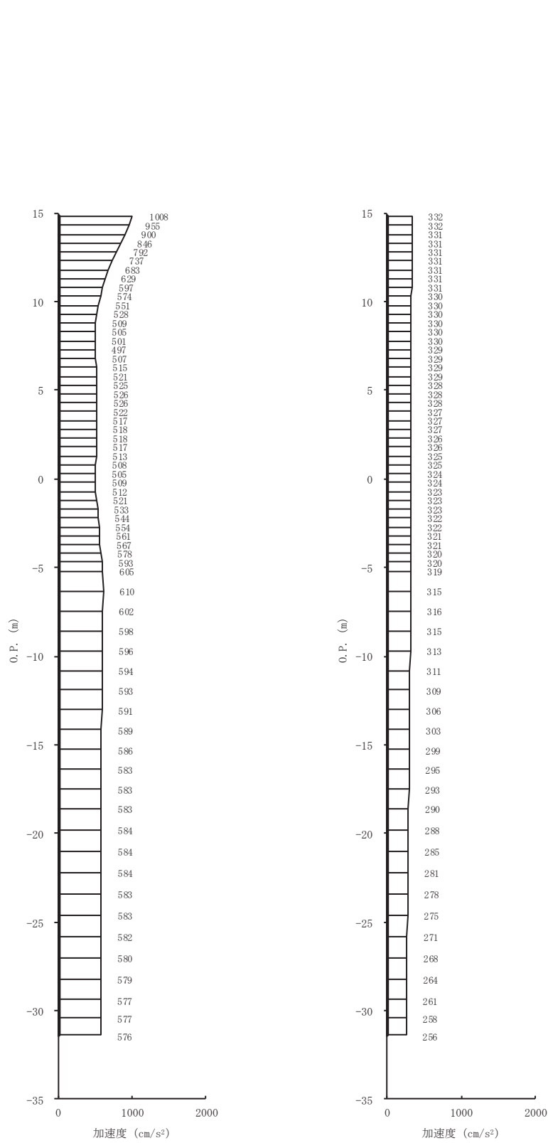
(a) S s - N 1 (++) 水平 (b) S s - N 1 (++) 鉛直 図 4-1(7) 最大加速度分布図 (7/28) (No. 1 揚水井戸, 解析ケース①)
