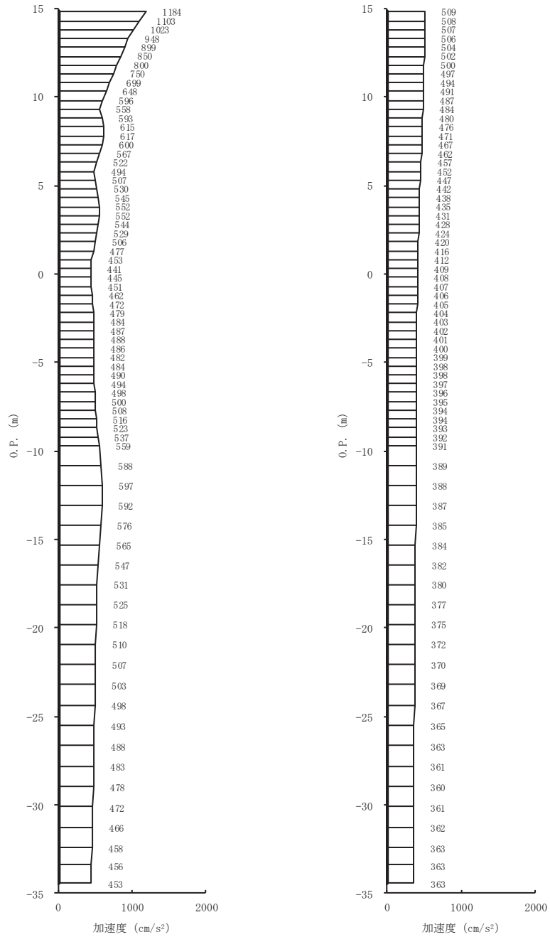
図 4-5(15) 最大加速度分布図 (15/28) (No. 2 揚水井戸, 解析ケース③)
