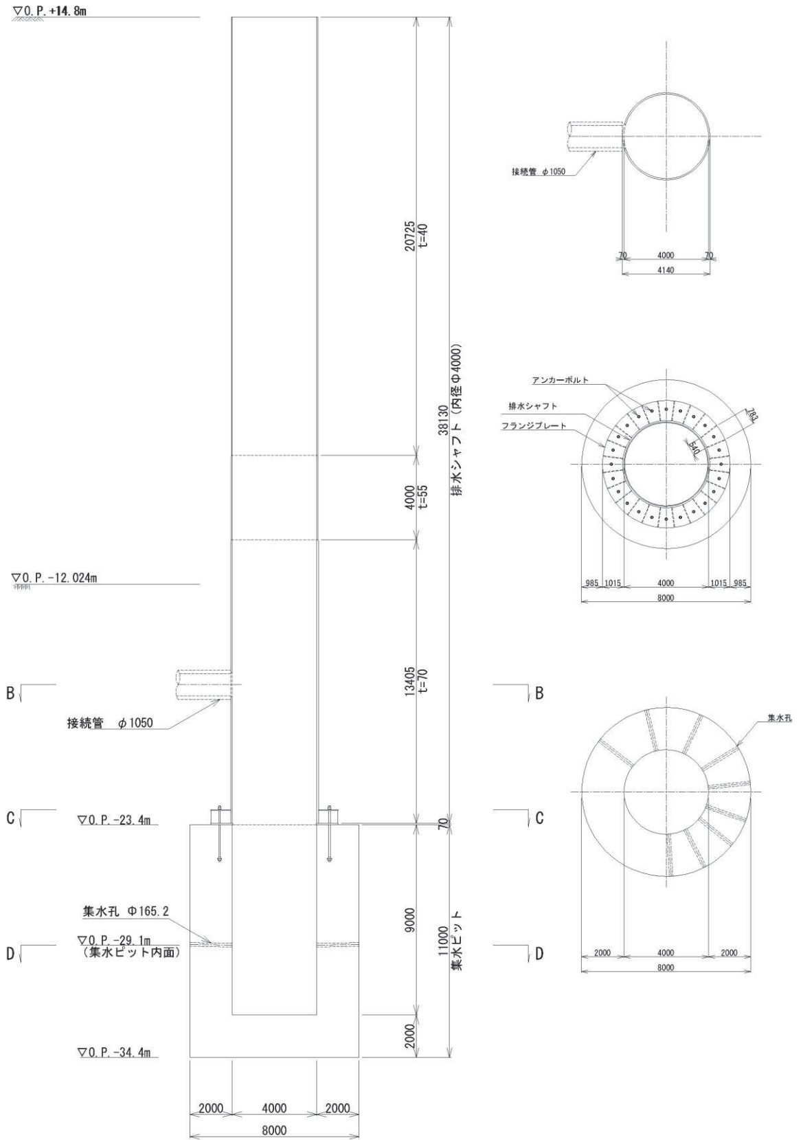
図 2-3(4) No.4 揚水井戸 構造図 (単位 : mm)
