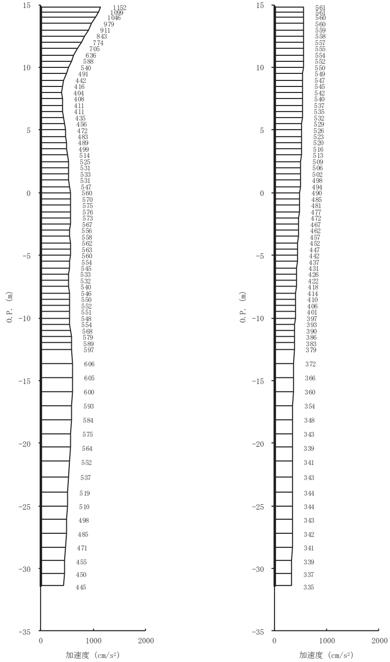
(a) Ss-D3 (++) 水平 (b) Ss-D3 (++) 鉛直
