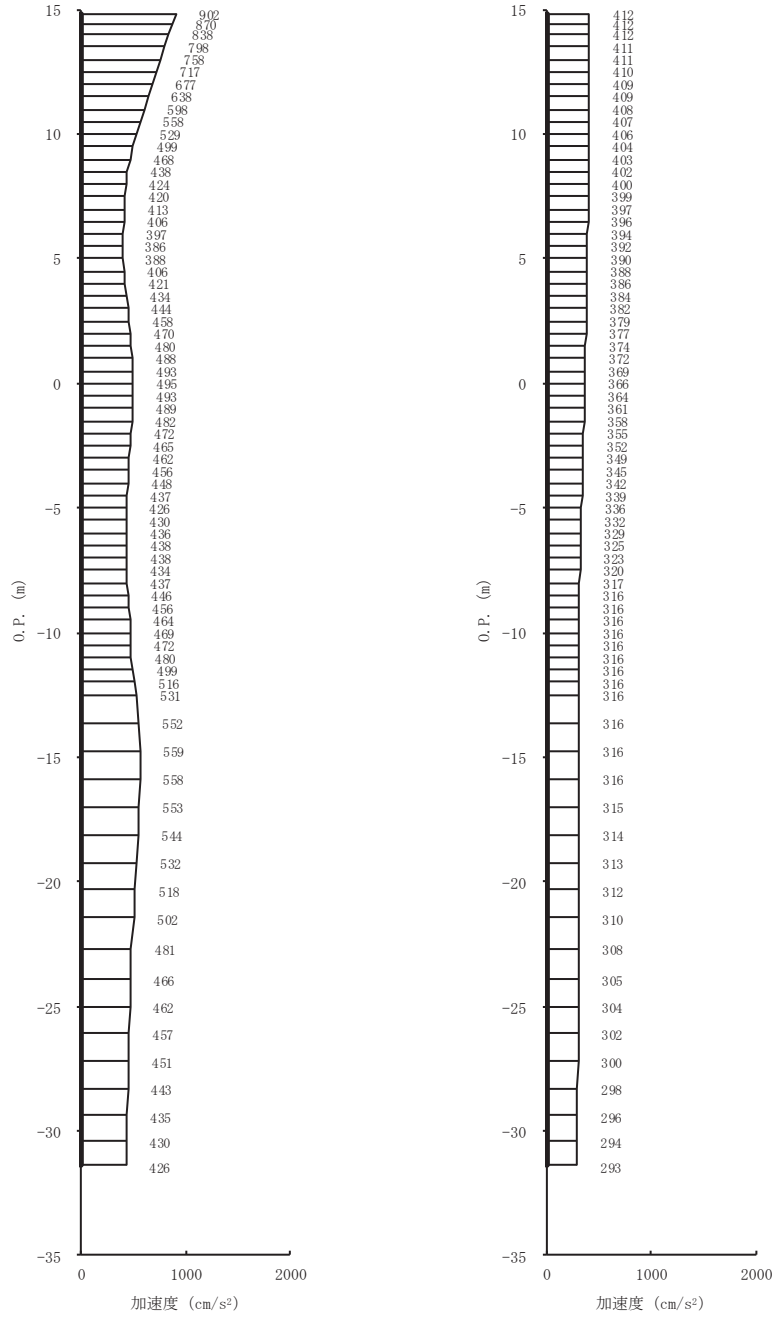
(a) Ss-F1 (++) 水平 (b) Ss-F1 (++) 鉛直
