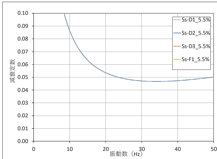
図 3.2-17(4) 設定した Ryaleigh 減衰 (鋼桁6) (地盤改良 (改良幅 2D 未満) 考慮)
