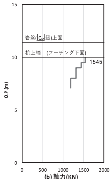
図 4.1-48 基礎地盤の支持性能照査時刻での軸力（押し込み時） (断面⑥, S s - D 2 ( - - ) , t = 11.43s) 解析ケース① : 基本ケース
