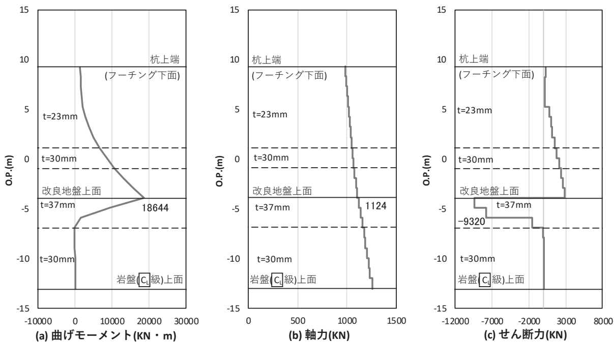
図 4.1-27 鋼管杭の曲げ・軸力系の破壊に対する照査における照査時刻での断面力 (断面①, S s - N 1 (-+), t = 7.82s)
