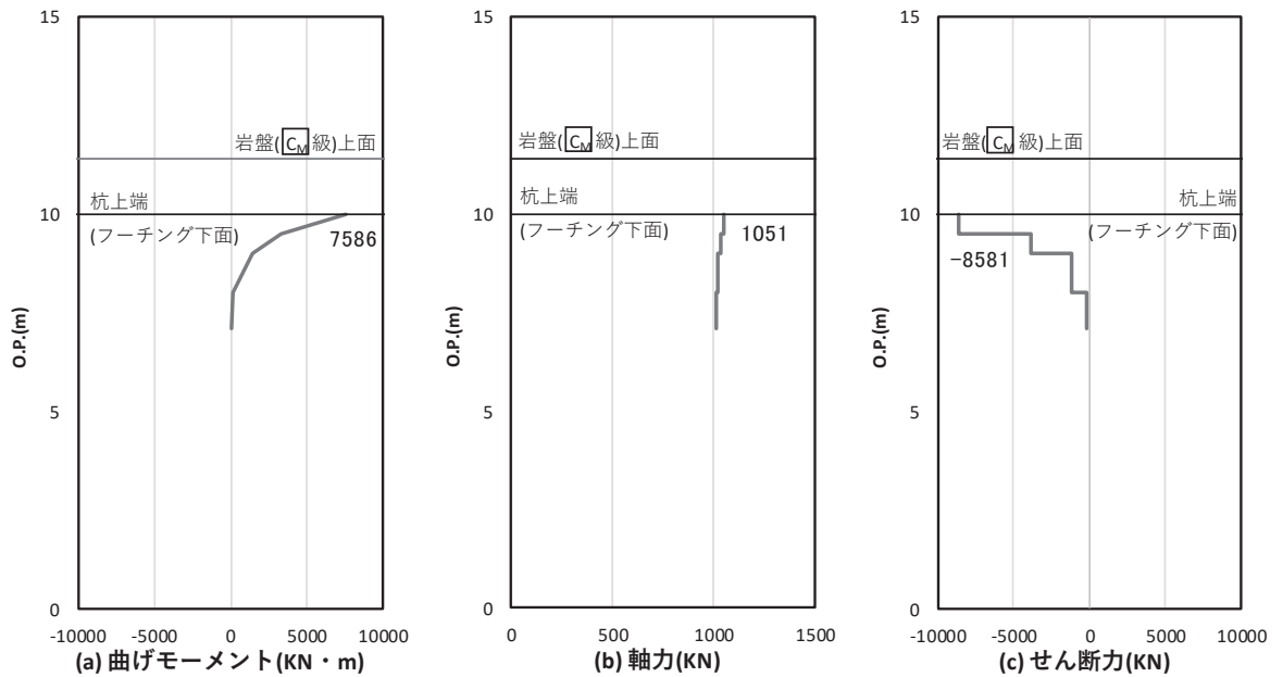
図 4.1-32 鋼管杭の曲げ・軸力系の破壊に対する照査における照査時刻での断面力 (断面⑥, S s - D 2 ( + - ) , t = 26.94s)
