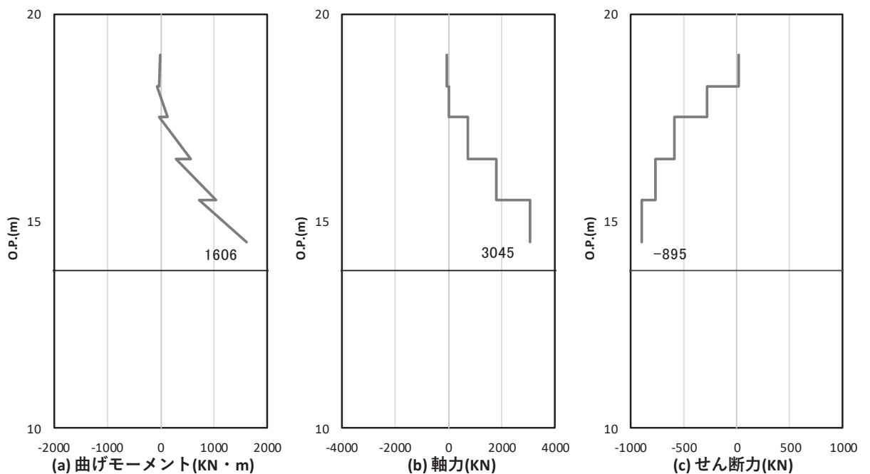
図 4.1-15(4) 鋼製支柱のせん断破壊に対する照査における照査時刻での断面力 (断面⑦張出部, S s - D 2 (++) , t = 26. 82s)
