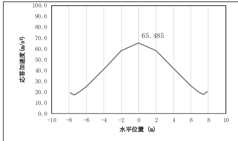
図 4.1-9(4) 鋼桁の水平応答震度分布 (鋼桁 3, S s-D 1 (一一))
