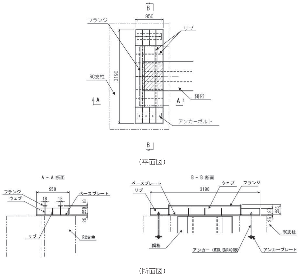
図 2.2-9(5) 鋼製遮水壁 (鋼桁 6) 上揚力反力梁
