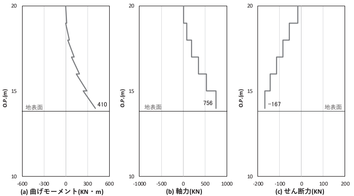
図 4.1-9(2) 鋼製支柱のせん断破壊に対する照査における照査時刻での断面力 (断面①, S s - N 1 (-+), t = 7.55s)
