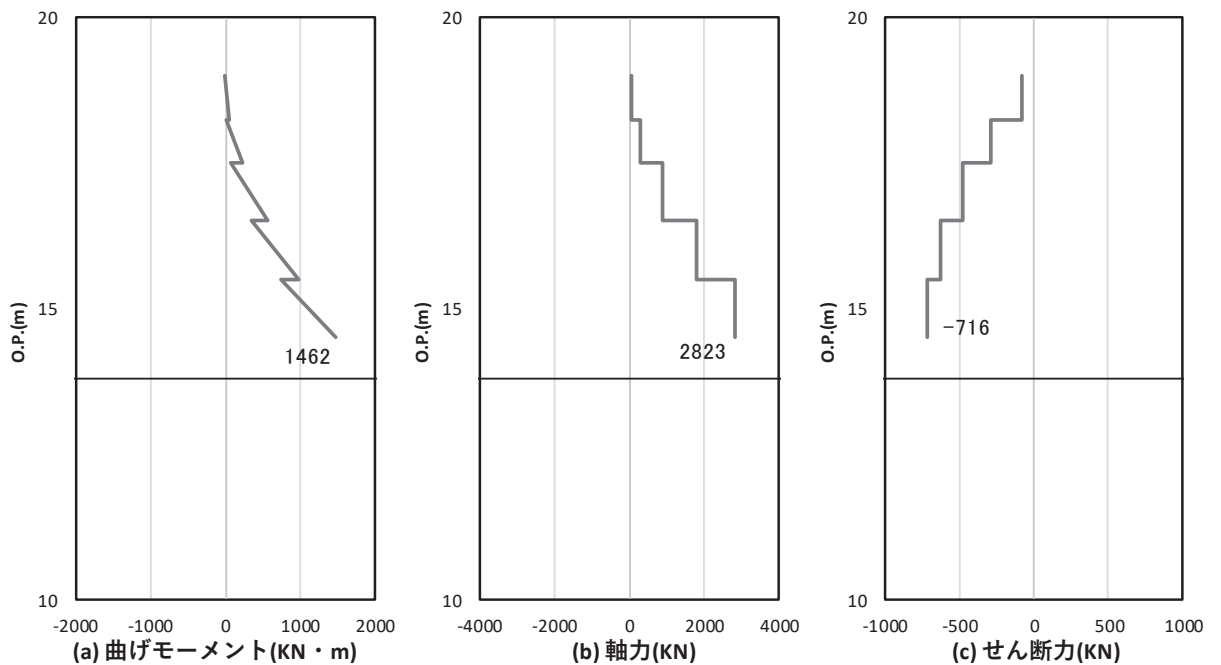
図 4.1-15(2) 鋼製支柱のせん断破壊に対する照査における照査時刻での断面力 (断面⑦一般部, S s - D 2 (+ -), t = 18.00s)
