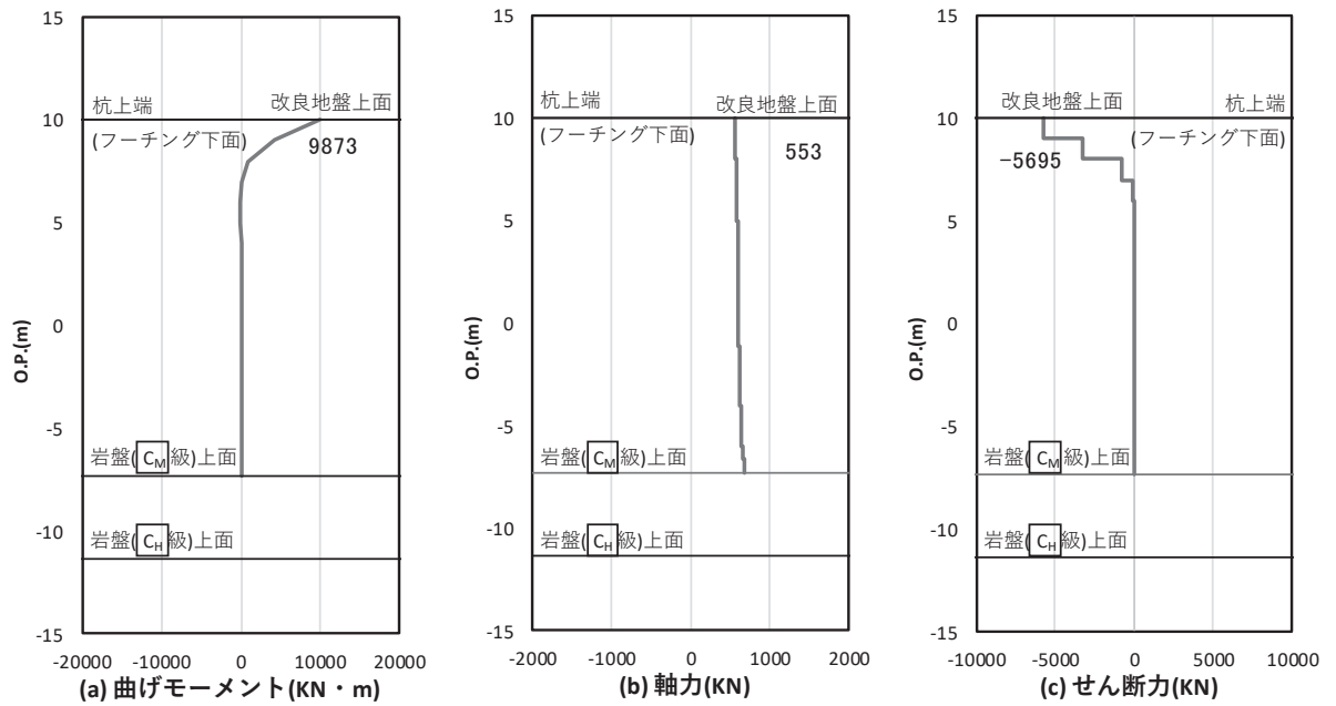
図 4.1-31 鋼管杭の曲げ・軸力系の破壊に対する照査における照査時刻での断面力 (断面⑤, S s - D 2 ( - + ) , t = 6.94s)
