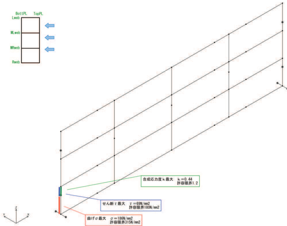
図 4.1-6(1) 鋼桁の曲げ・軸力系の破壊及びせん断破壊に対する最大照査値発生箇所（鋼桁 6）
