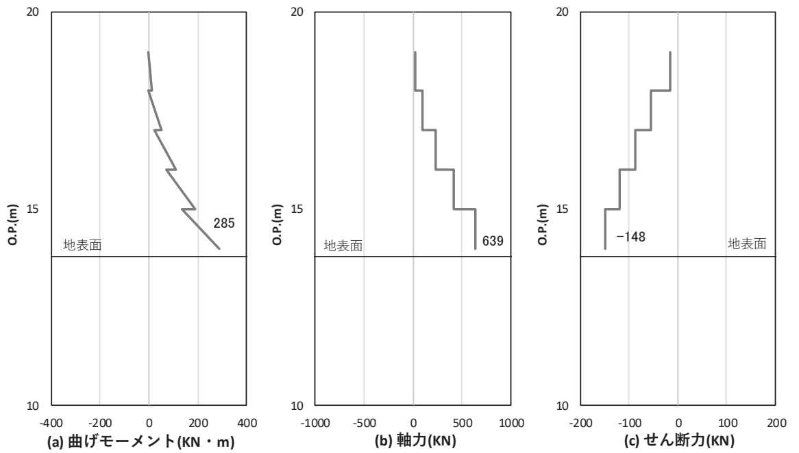
図 4.1-16(1) 鋼製支柱の曲げ・軸力系の破壊に対する照査における照査時刻での断面力 (断面⑧, S_s-N1 (-+), t=7.59s )
