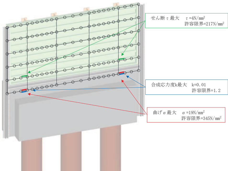
図 4.1-8 鋼板の曲げ・軸力系の破壊及びせん断破壊に対する 最大照査値発生箇所 (断面⑧)
