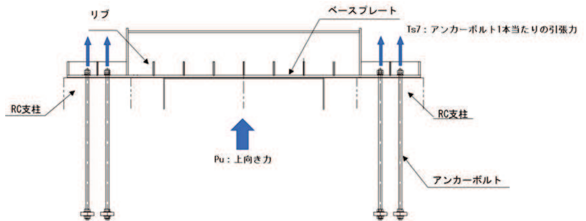
図 3.8-26 アンカーボルト荷重概念図
