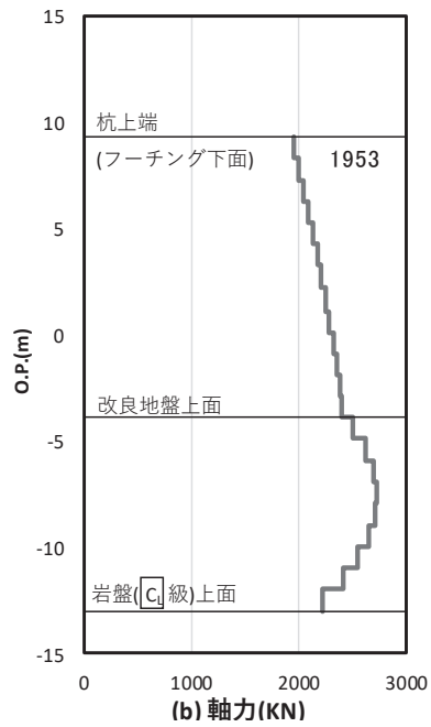
図 4.1-43 基礎地盤の支持性能照査時刻での軸力（押し込み時） (断面①, S_s - D2 (++) , t = 23.56s )
