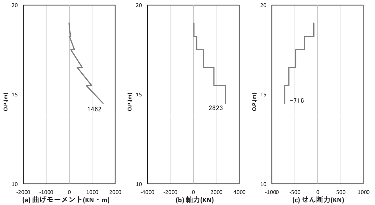
図 4.1-15(1) 鋼製支柱の曲げ・軸力系の破壊に対する照査における照査時刻での断面力 (断面⑦一般部, S s - D 2 (+ -), t = 18.00s)
