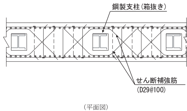
図 4.5-1 ペDESTAL配筋概要図 (断面④の例)
