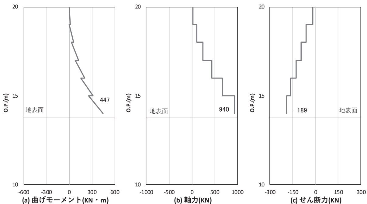
図 4.1-10(1) 鋼製支柱の曲げ・軸力系の破壊に対する照査における照査時刻での断面力 (断面②, S s - N 1 (++) , t = 7.61s) 解析ケース①: 基本ケース
