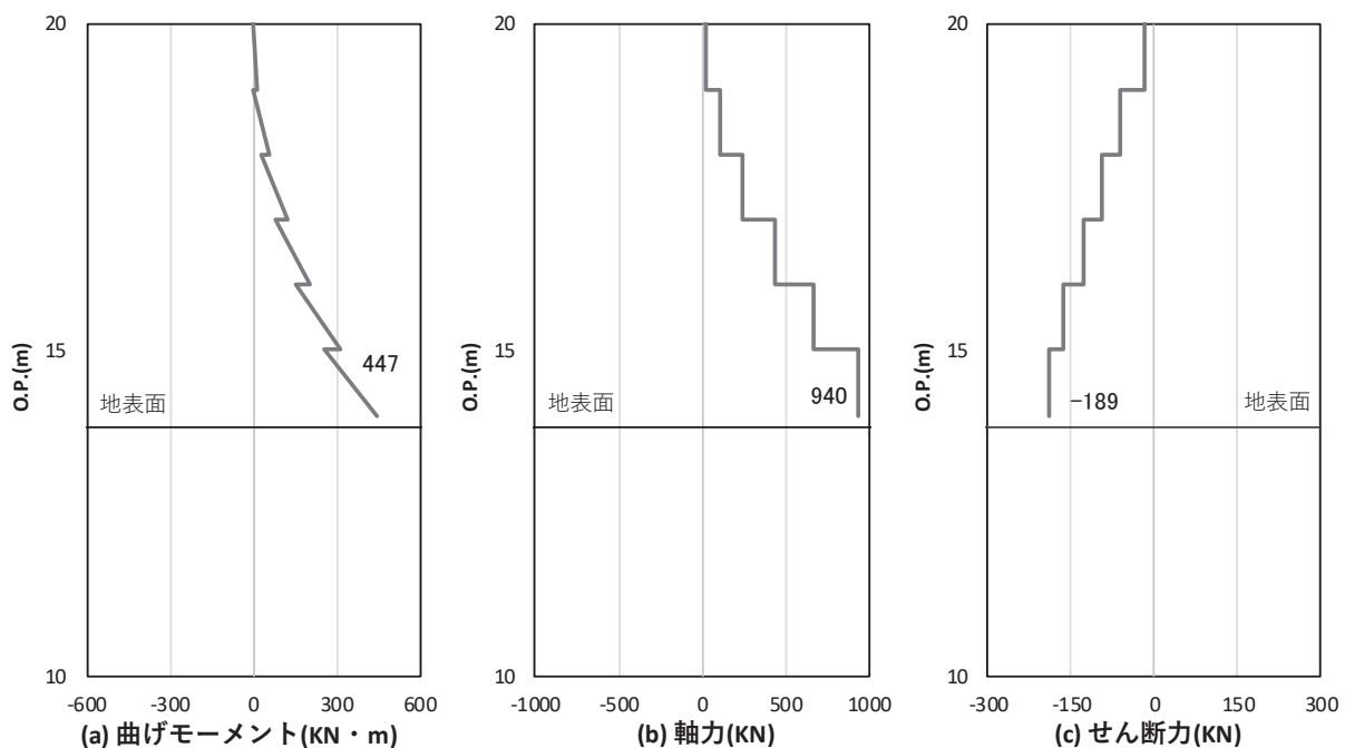
図 4.1-10(2) 鋼製支柱のせん断破壊に対する照査における照査時刻での断面力 (断面②, S s - N 1 (++) , t = 7.61s) 解析ケース①: 基本ケース
