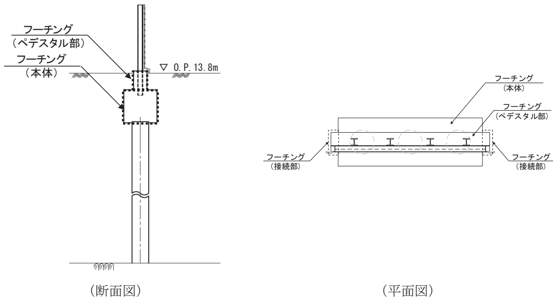
図 3.7-5 フーチングの照査範囲の概念図
