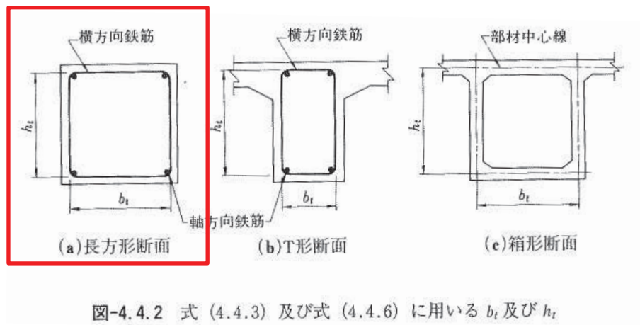
図 3.8-3 ねじりによる応力度算出に用いる b_t 及び h_t (道路橋示方書 (I 共通編・III コンクリート橋編) ・同解説 (平成 14 年 3 月) より抜粋)
