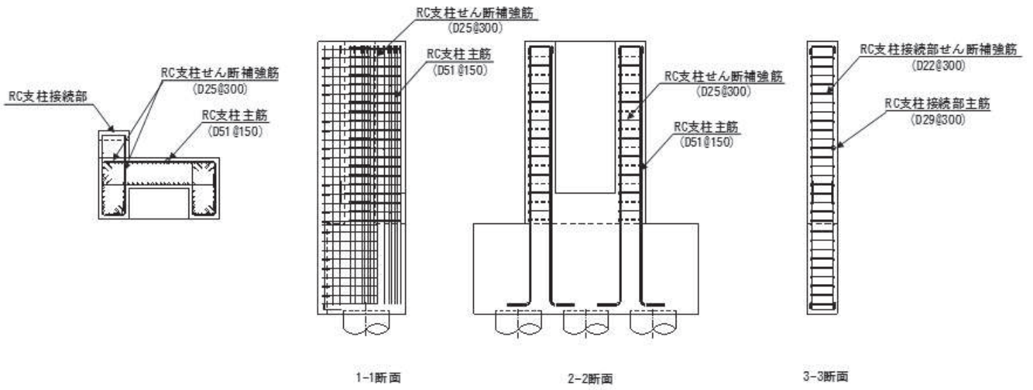
図 2.2-13 鋼製遮水壁（鋼桁）の RC 支柱配筋概要図
