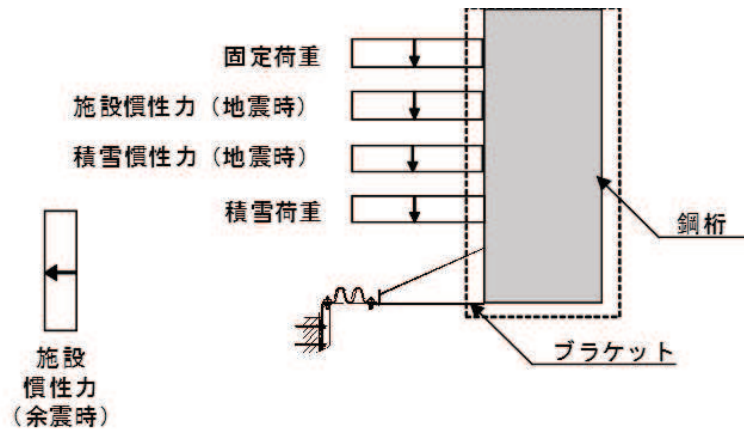
図 3.8-10 作用荷重図
