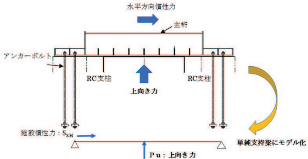
図 3.8-21 解析モデル図
