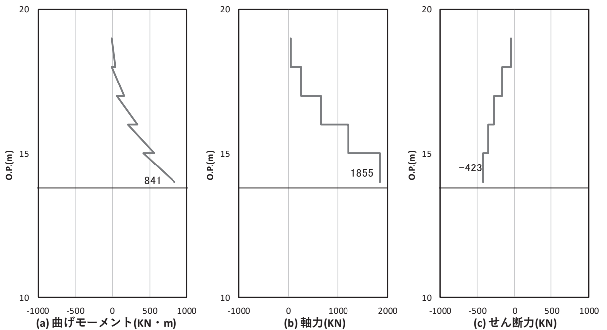
図 4.1-12(2) 鋼製支柱のせん断破壊に対する照査における照査時刻での断面力 (断面④, S s - D 2 (+ -), t = 13.40s)
