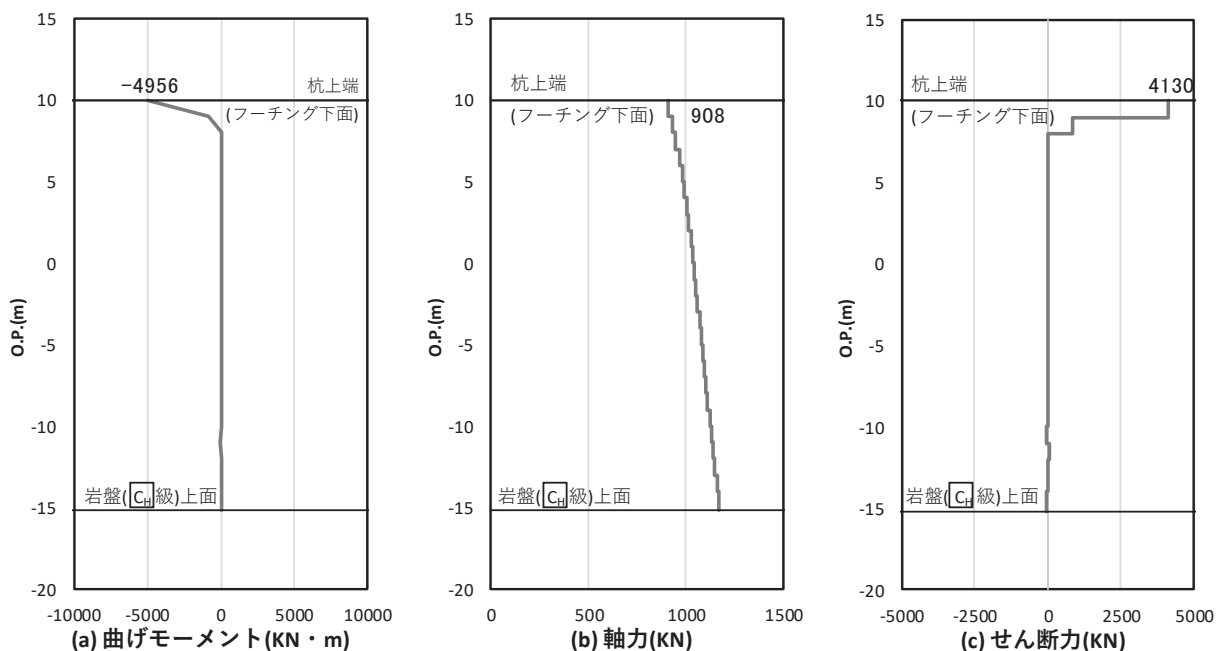
図 4.1-38 鋼管杭のせん断破壊に対する照査における照査時刻での断面力 (断面④, S_s - D2 (+ -) , t = 13.40s )
