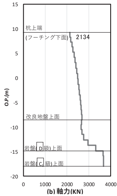
図 4.1-44 基礎地盤の支持性能照査時刻での軸力（押し込み時） (断面②, S_s - D2 (++) , t = 23.56s )
