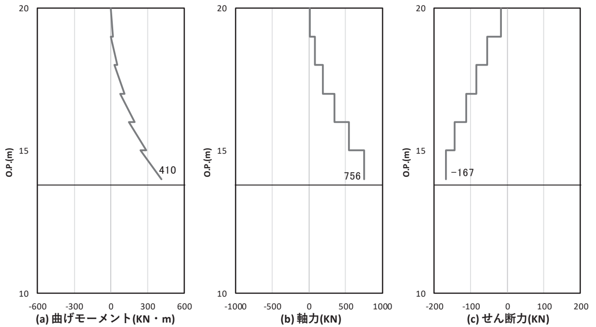
図 4.1-9(1) 鋼製支柱の曲げ・軸力系の破壊に対する照査における照査時刻での断面力 (断面①, S s - N 1 (-+), t = 7.55s)
