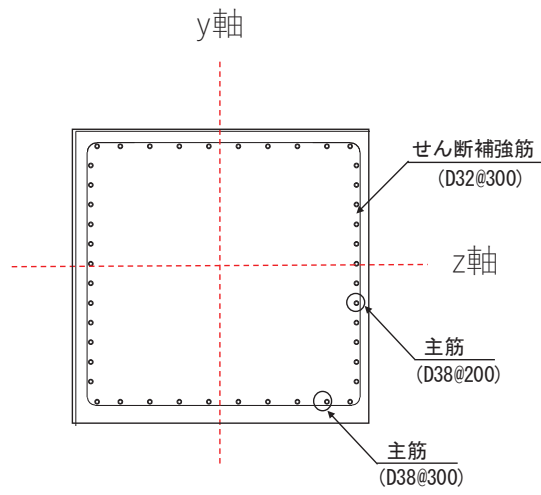
図 4.1-17 フーチング配筋概要図 (断面①の例)
