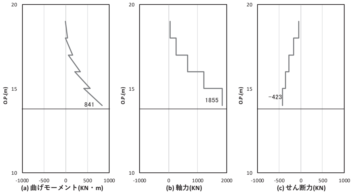
図 4.1-12(1) 鋼製支柱の曲げ・軸力系の破壊に対する照査における照査時刻での断面力 (断面④, S s - D 2 (+ -), t = 13.40s)
