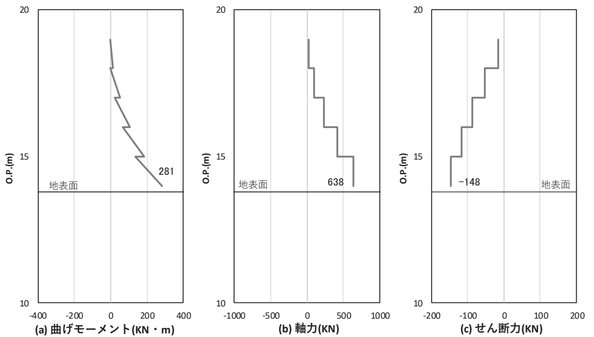
図 4.1-16(2) 鋼製支柱のせん断破壊に対する照査における照査時刻での断面力 (断面⑧, S_s-N1 (-+), t=7.60s )
