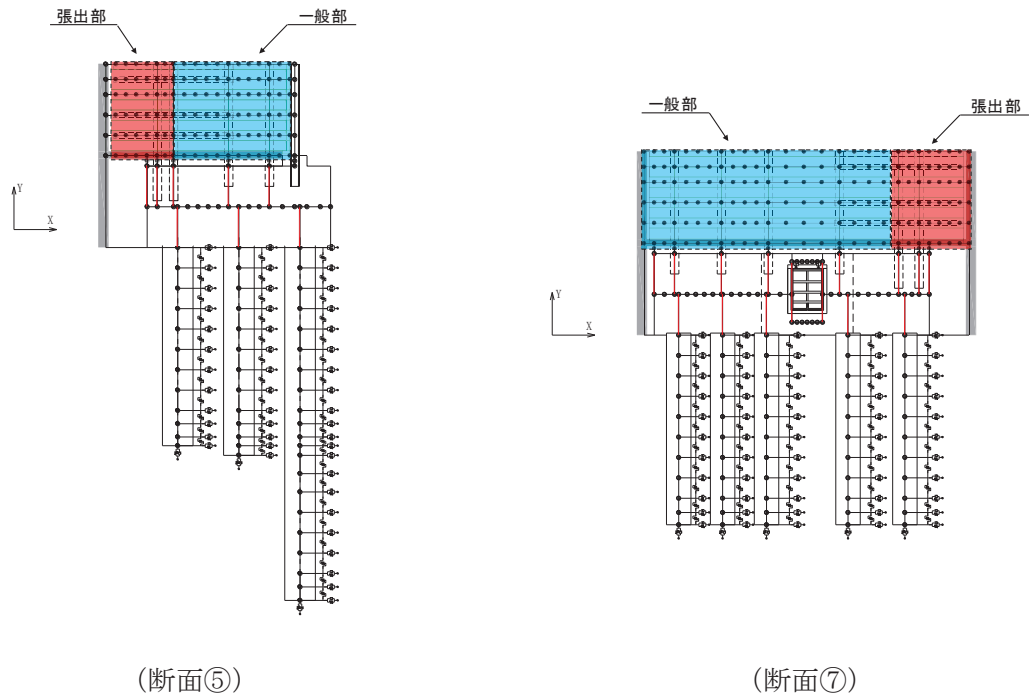
図 3.7-3 断面⑤, ⑦に関する鋼板の名称
