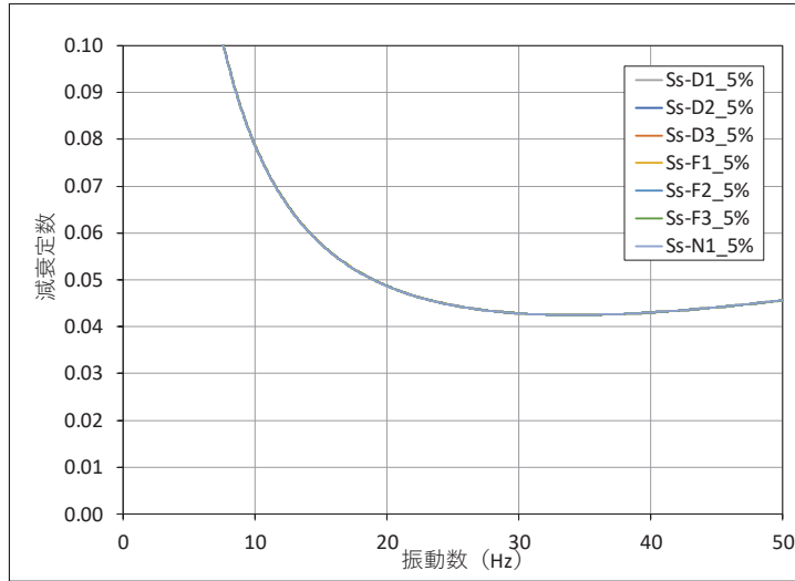
図 3.2-17(3) 設定した Ryaleigh 減衰 (鋼桁6) (地盤改良 (改良幅 2D 未満) 考慮)
