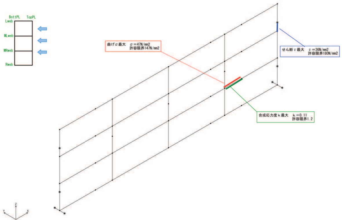
図 4.1-5(1) 鋼桁の曲げ・軸力系の破壊及びせん断破壊に対する 最大照査値発生個所 (鋼桁 5)
