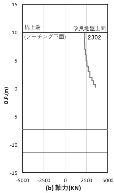
図 4.1-47 基礎地盤の支持性能照査時刻での軸力（押し込み時） (断面⑤, S s - D 3 ( - + ) , t = 7.54s) 解析ケース③ : 地盤物性のばらつき ( - 1 \sigma ) を考慮した解析ケース
