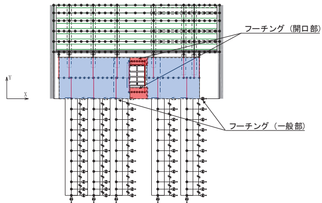
図 3.7-6(1) 断面⑦に関するフーチング（本体）の照査分類
