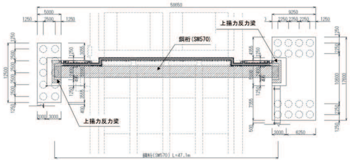
図 2.2-7(2) 鋼製遮水壁（鋼桁4） 平面図
