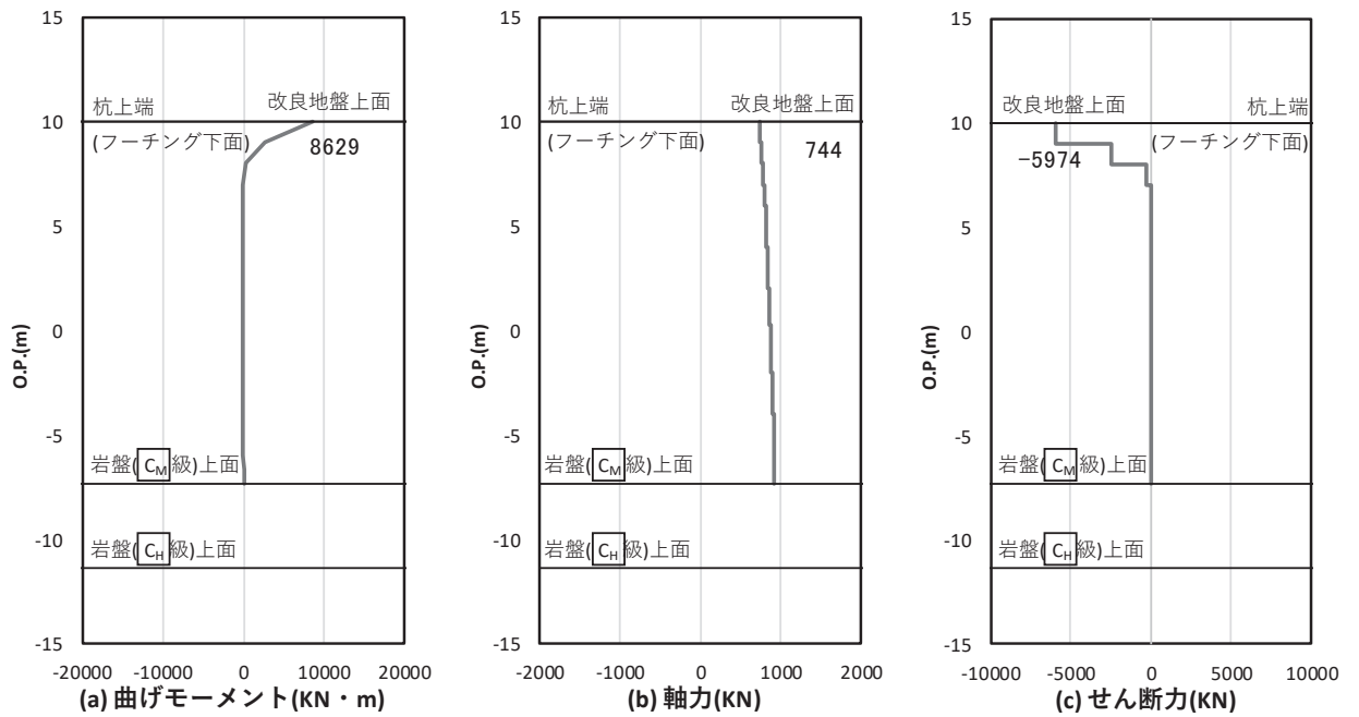
図 4.1-39 鋼管杭のせん断破壊に対する照査における照査時刻での断面力 (断面⑤, S s - D 3 (-+), t = 7.23s) 解析ケース①: 基本ケース
