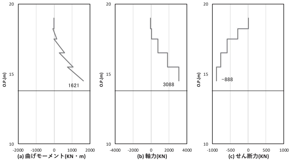
図 4.1-15(3) 鋼製支柱の曲げ・軸力系の破壊に対する照査における照査時刻での断面力 (断面⑦張出部, S s - D 2 (++) , t = 26. 81s)
