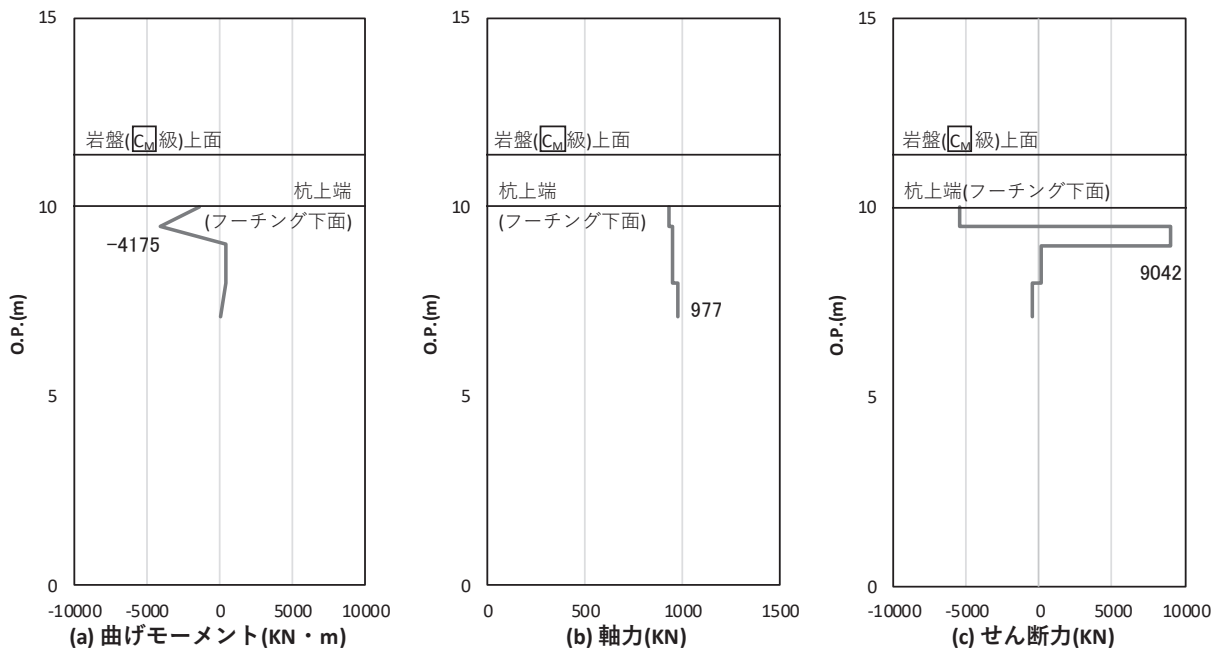
図 4.1-40 鋼管杭のせん断破壊に対する照査における照査時刻での断面力 (断面⑥, S s - D 1 (-+), t = 19.80s) 解析ケース①: 基本ケース
