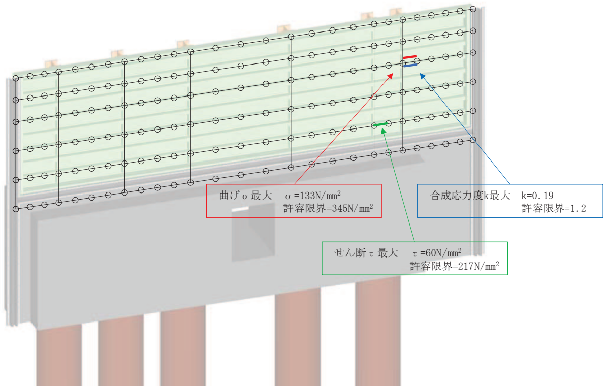
図 4.1-7(2) 鋼板の曲げ・軸力系の破壊及びせん断破壊に対する 最大照査値発生箇所 (断面⑦張出部)
