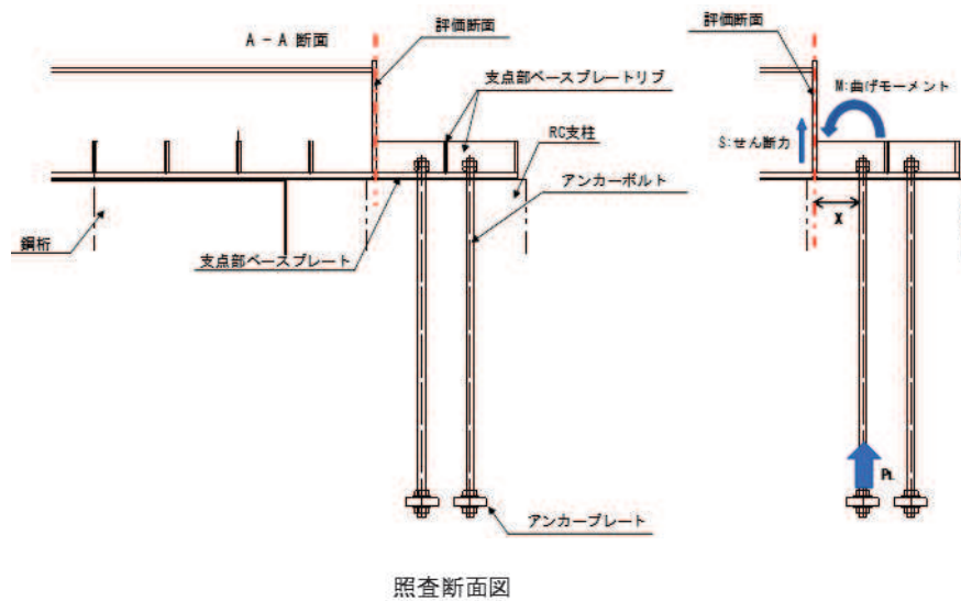
照査断面図
