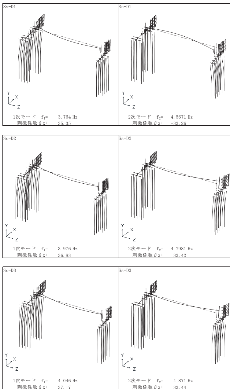
図 3.2-7(1) 固有値解析結果 (鋼桁 4 : モード図) 鋼桁軸直交方向
