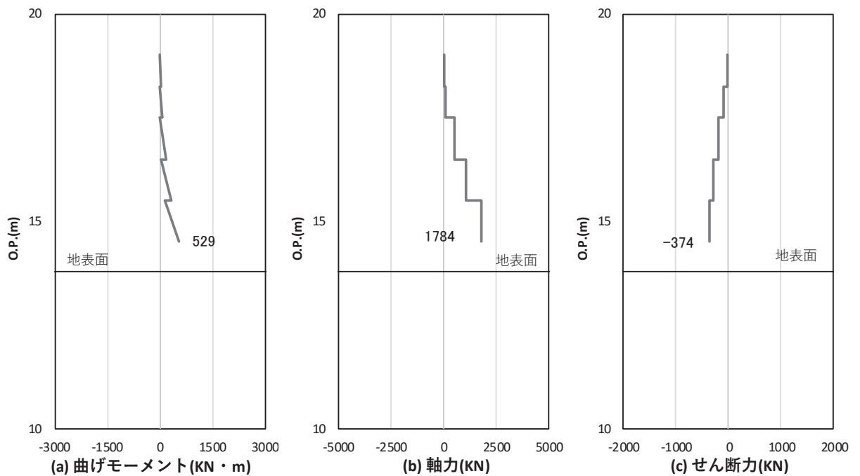
図 4.1-13(2) 鋼製支柱のせん断破壊に対する照査における照査時刻での断面力 (断面⑤一般部, S s - D 2 (-+), t = 20.45s)
