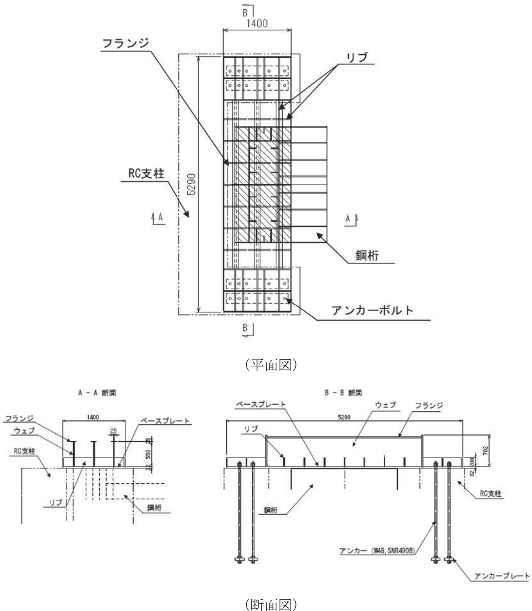
図3.8-18 上揚力反力梁構造概要
