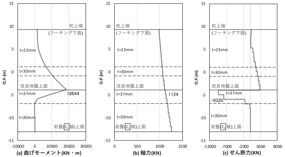
図 4.1-35 鋼管杭のせん断破壊に対する照査における照査時刻での断面力 (断面①, S_s - N1 (-+) , t = 7.82s )
