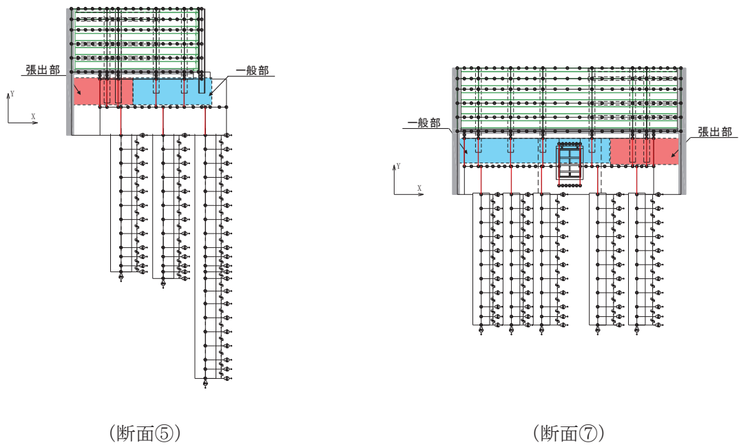
図 3.7-6(2) 断面⑤, ⑦に関するフーチング（ペDESTAL部）の照査分類
