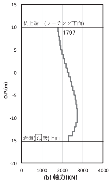
図 4.1-46 基礎地盤の支持性能照査時刻での軸力（押し込み時） （断面④， S_s - D 1 （--）， t = 20.40s ）
