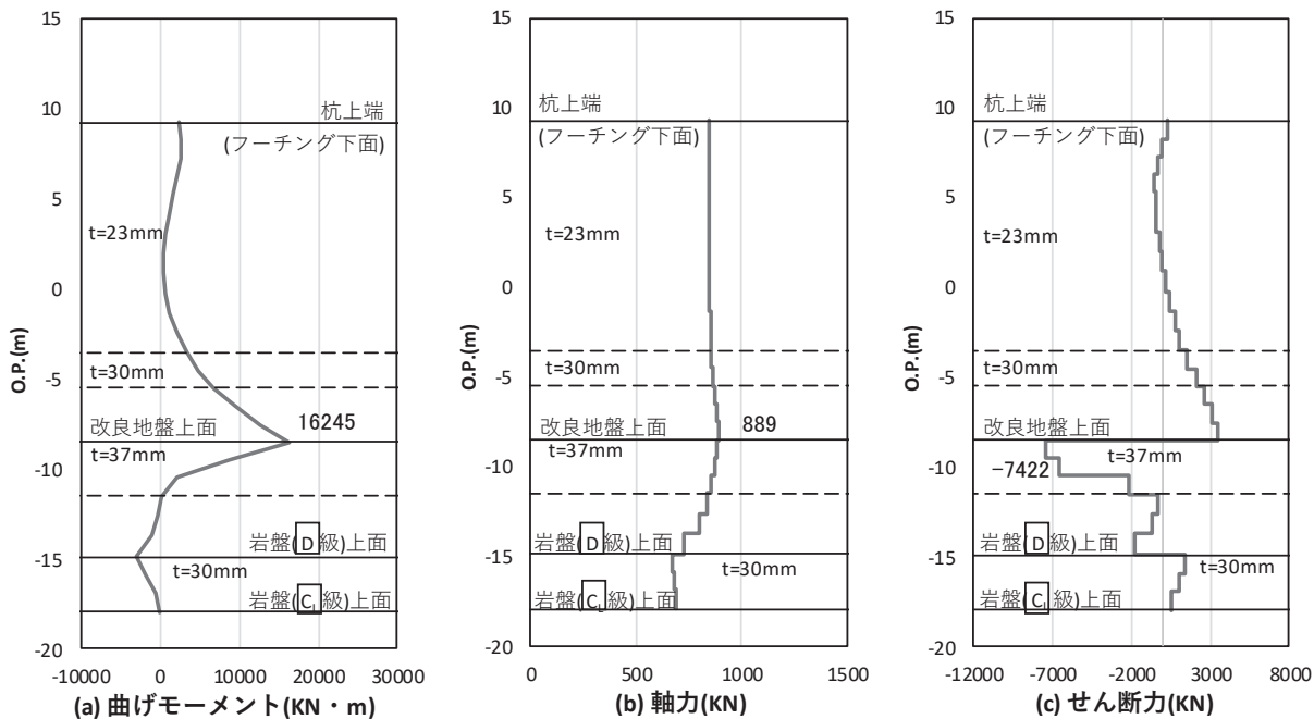
図 4.1-28 鋼管杭の曲げ・軸力系の破壊に対する照査における照査時刻での断面力 (断面②, S s - N 1 (++) , t = 7.77s)
