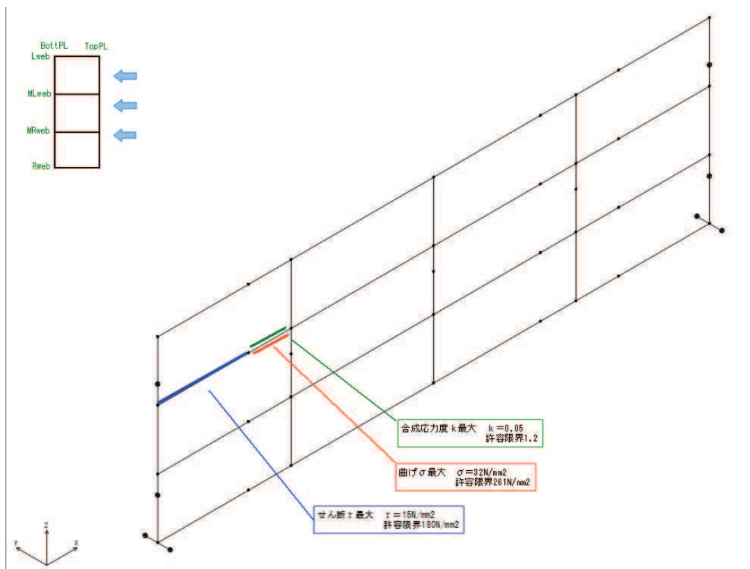
図 4.1-5(1) 鋼桁の曲げ・軸力系の破壊及びせん断破壊に対する 最大照査値発生個所 (鋼桁 5) (地盤改良 (改良幅 2D 未満) 考慮)
