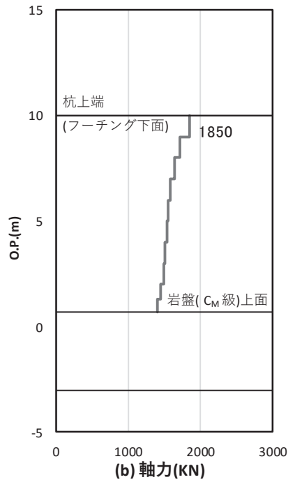
図 4.1-49 基礎地盤の支持性能照査時刻での軸力 (断面⑦, S_s - D2 (+) , t = 11.43s )
