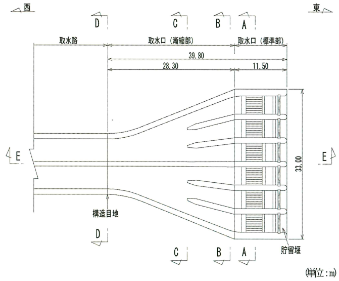
図 2-2 取水口平面図
