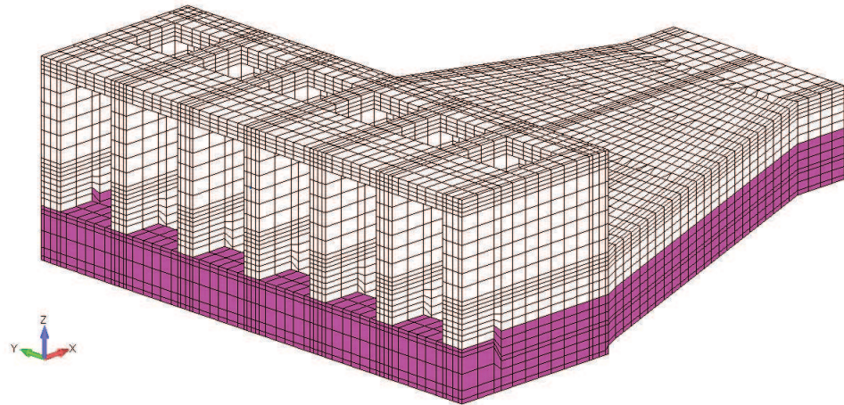
図 6-31 貯水機能が要求される部材の範囲
