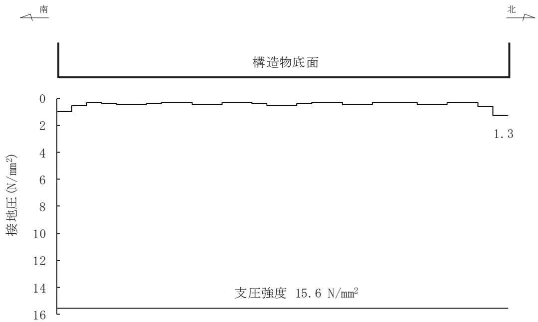
図 6-35(1) MMR (既設) の最大接地圧分布図 (全応力解析) (解析ケース①, S s - D 2 (++) , B-B 断面 (漸縮部))
