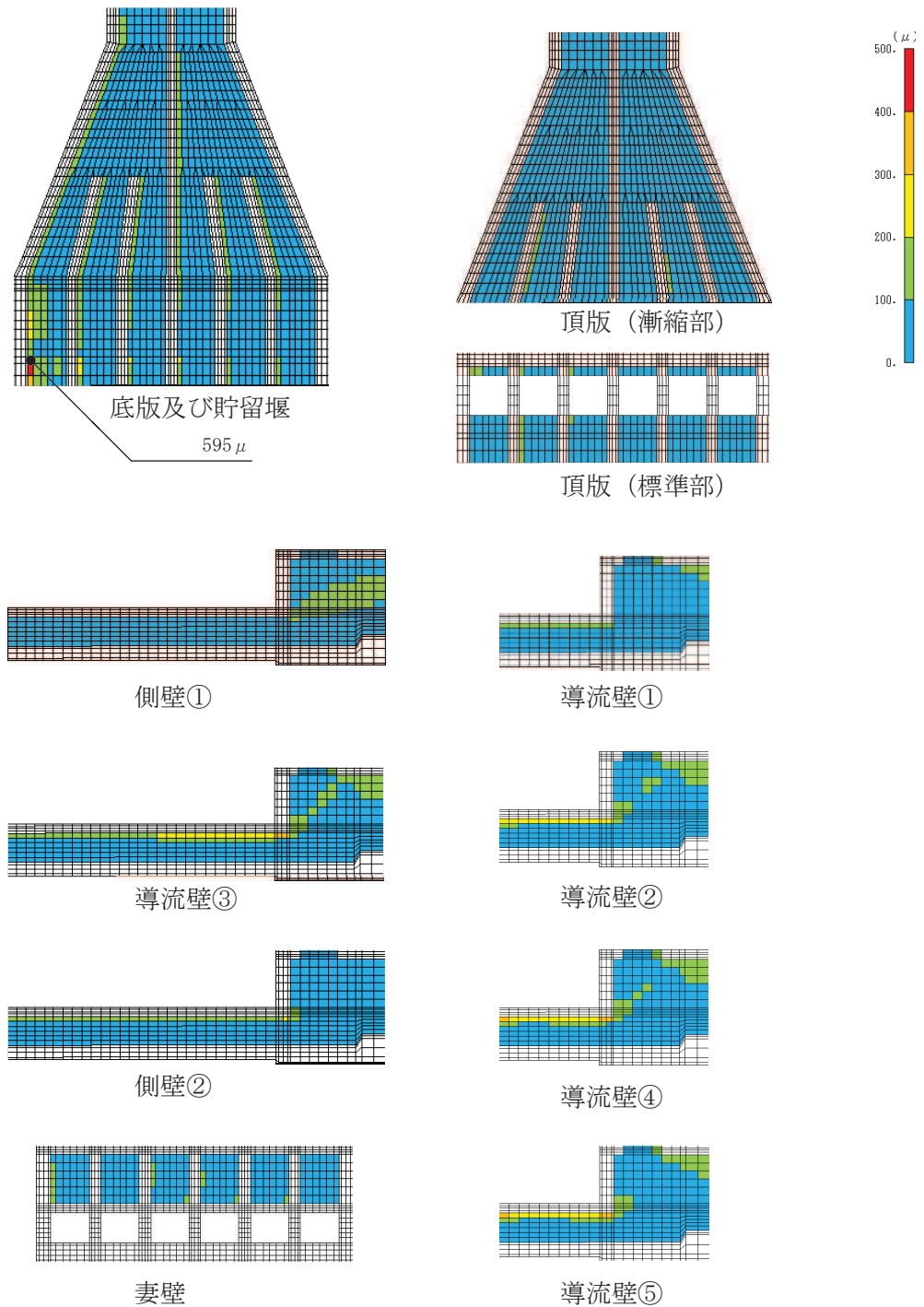
図 6-20(1) 曲げ・軸力系の破壊に対する照査値最大時のひずみ分布図 (全応力解析) (コンクリートの圧縮縁ひずみ) (貯留堰, 解析ケース③, 地震動 S_s - D2 (-+)) (標準部 t = 25.08s , 漸縮部 t = 25.06s )
