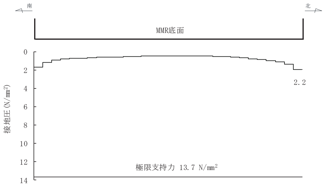
図 6-33(2) 基礎地盤の最大接地圧分布図（有効応力解析） （解析ケース⑥，S s -F2（-+），B-B断面（漸縮部））
