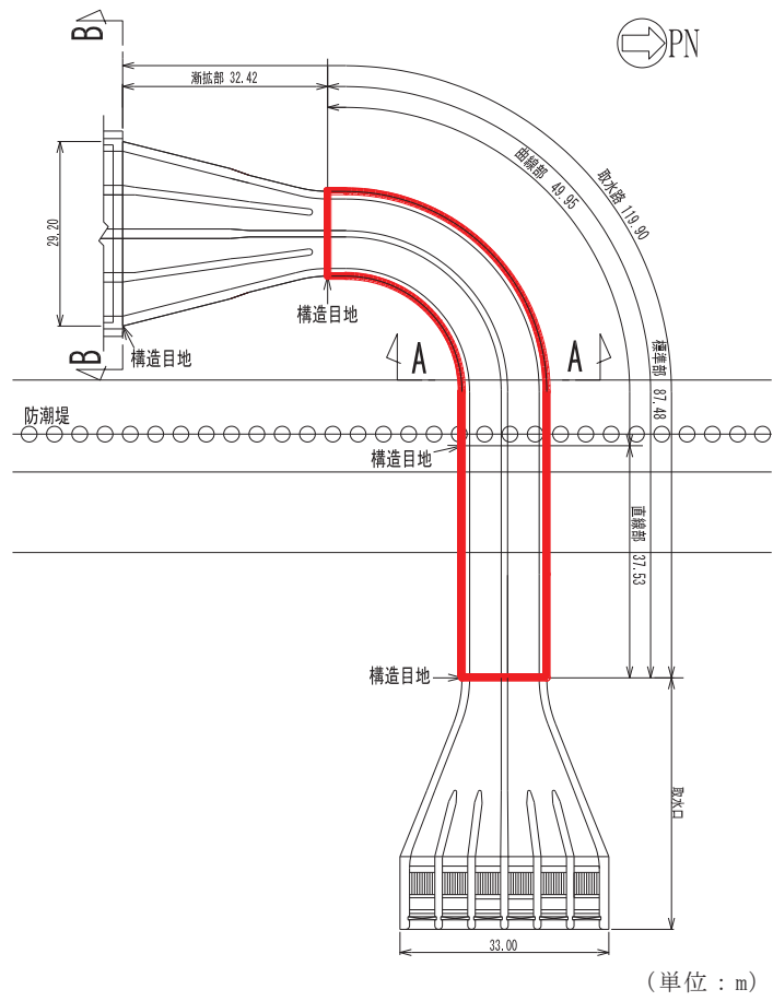
図 2-2 取水路（標準部）平面図
