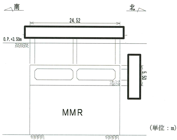
図 2-5 取水口断面図 (C-C 断面, 南北 (漸縮部))
