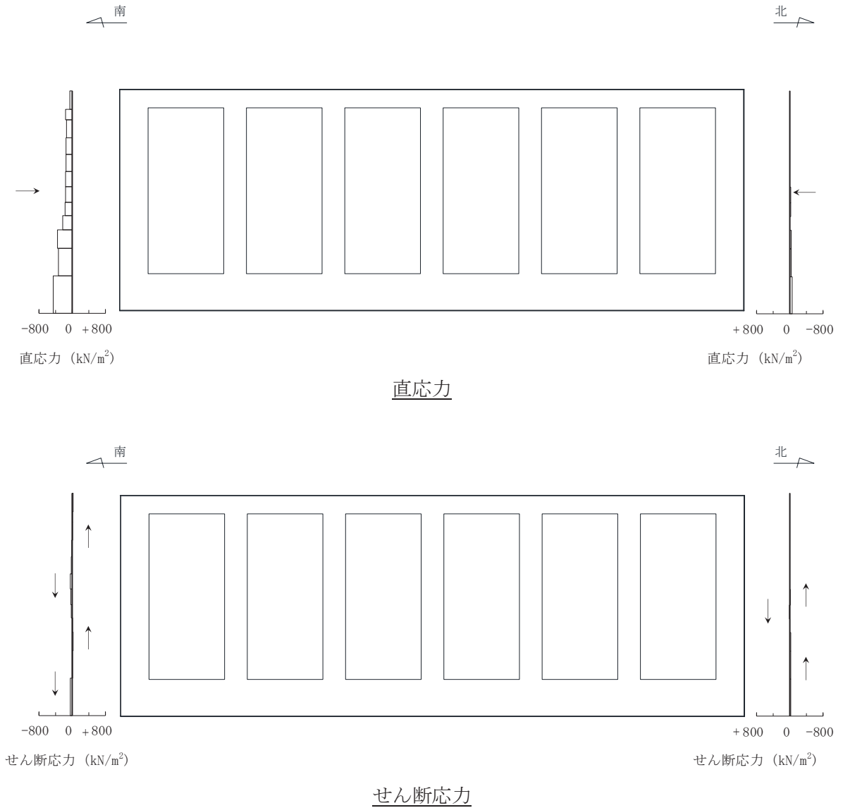
図6-1(1) 作用荷重分布図（直応力及びせん断応力）（全応力解析） （解析ケース①， S_s - D_2 （-+），A-A断面（標準部）， t = 25.07s ）
