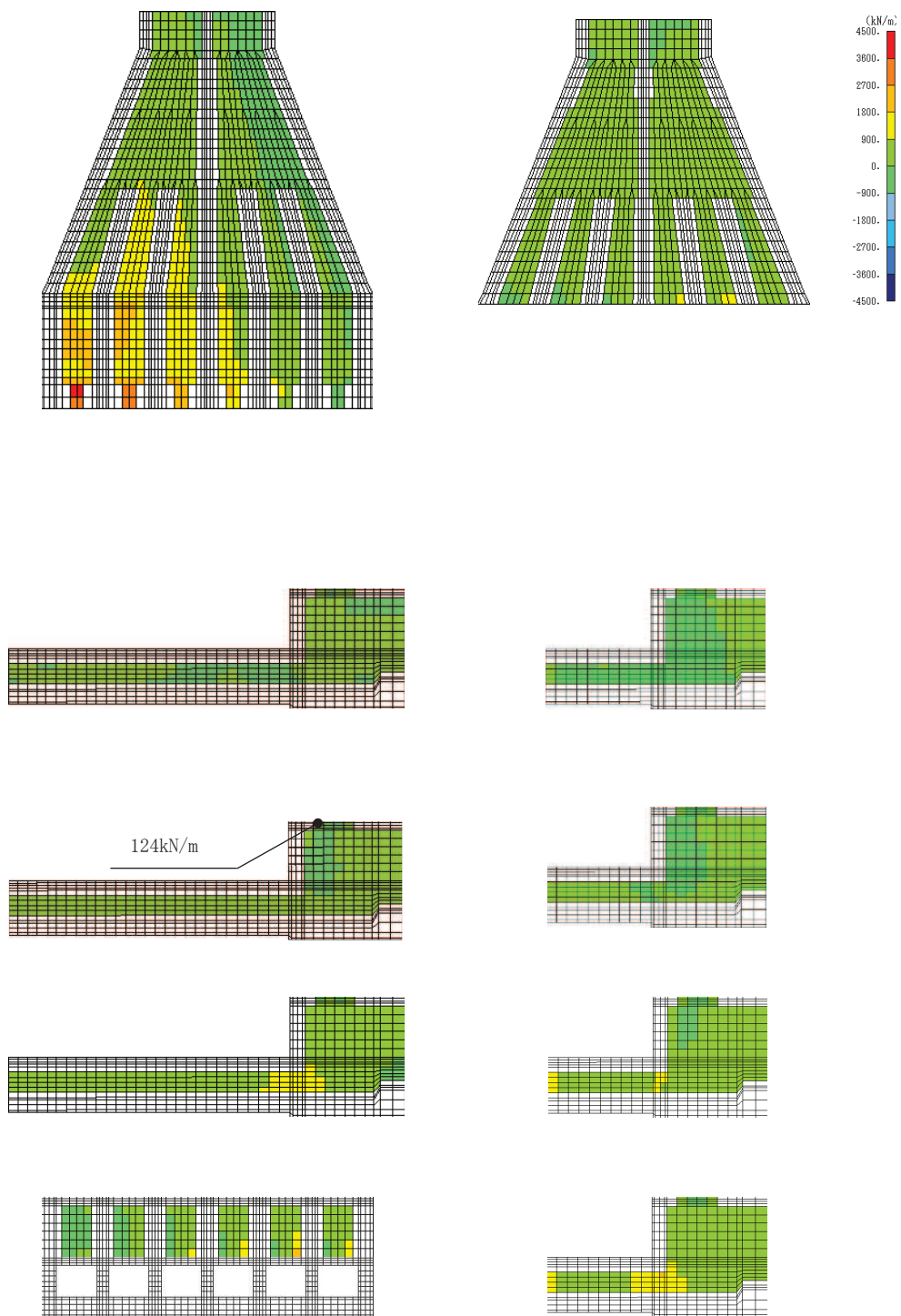
図 6-26(1) せん断破壊に対する照査値最大時の断面力分布図 (全応力解析) (軸力 (kN/m) : N_x ) (導流壁, 解析ケース①, 地震動 S_s - D2 (-+)) (標準部 t = 25.07s , 漸縮部 t = 25.06s )
