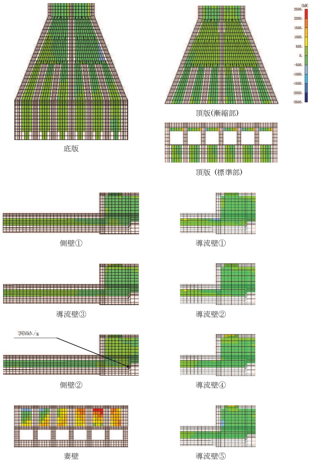
図 6-27(2) せん断破壊に対する照査値最大時の断面力分布図 (有効応力解析)
