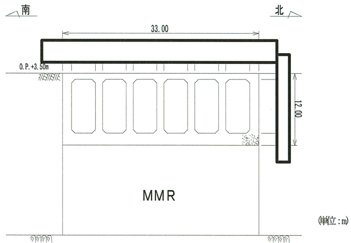
図 2-3 取水口断面図 (A-A 断面, 南北 (標準部))
