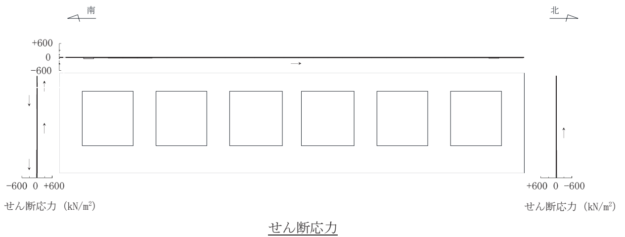
図 6-3(1) 作用荷重分布図 (直応力及びせん断応力) (全応力解析) (解析ケース①, S_s - D_2 (-+) , B-B 断面 (漸縮部), t = 25.06s )
