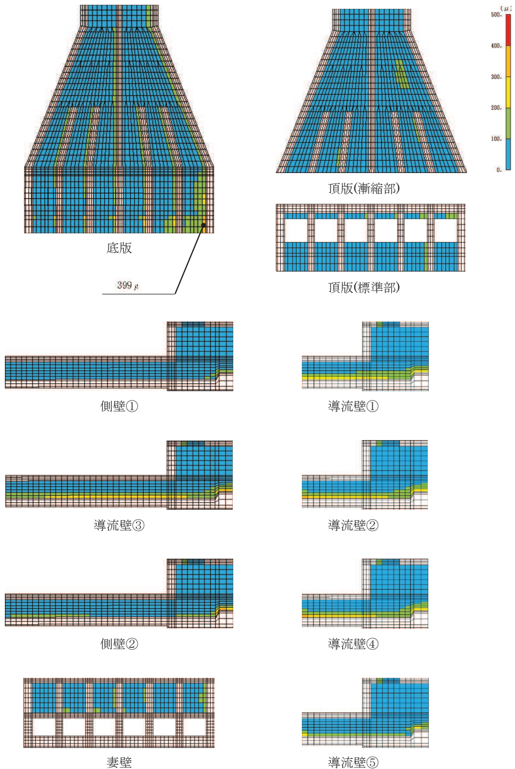
図 6-21(2) 曲げ・軸力系の破壊に対する照査値最大時のひずみ分布図
