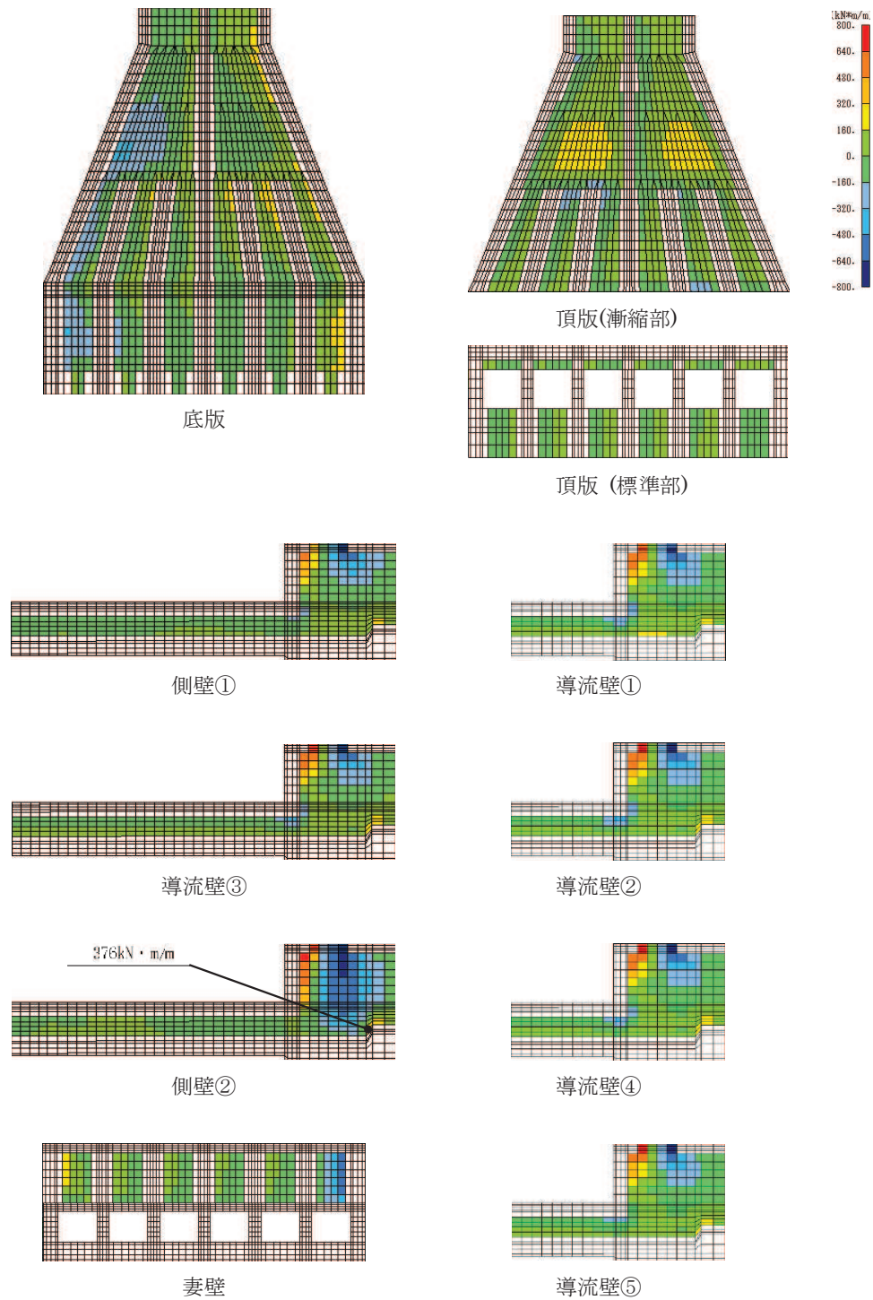
図 6-25(2) せん断破壊に対する照査値最大時の断面力分布図 (有効応力解析)
