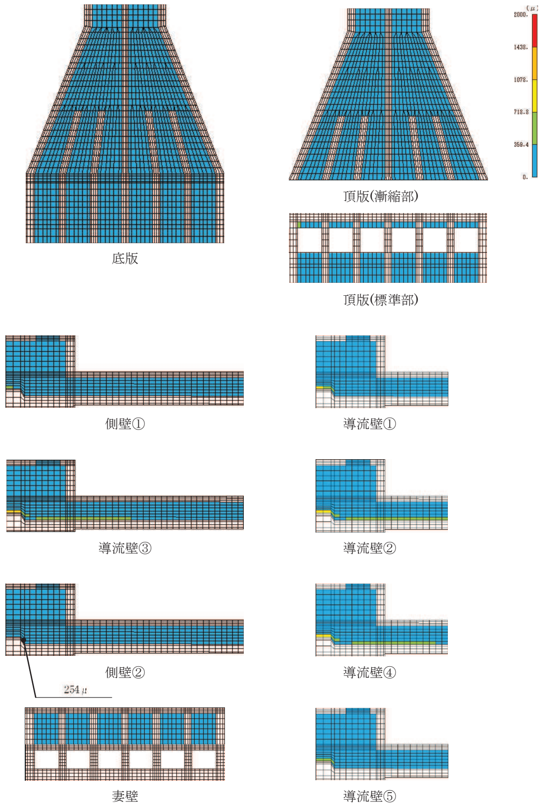
図 6-22 (2) 曲げ・軸力系の破壊に対する照査値最大時のひずみ分布図 (鉄筋：有効応力解析)
