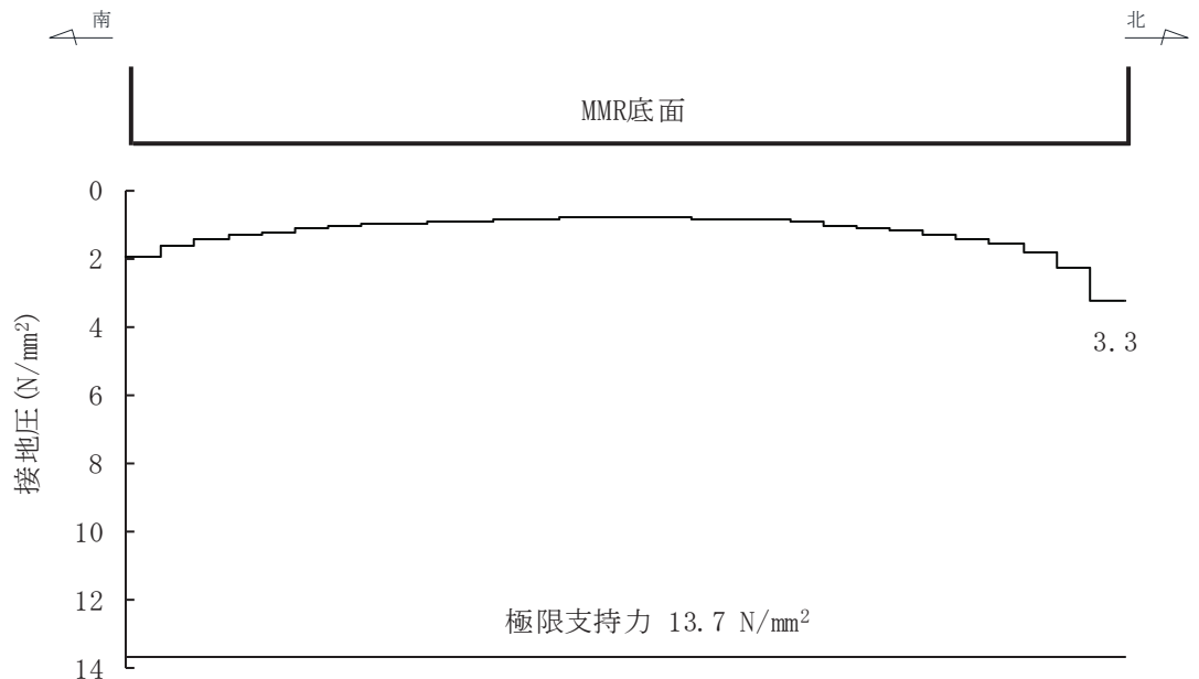
図 6-32(1) 基礎地盤の最大接地圧分布図（全応力解析） （解析ケース①，S s - D 1（++），A-A断面（標準部））
