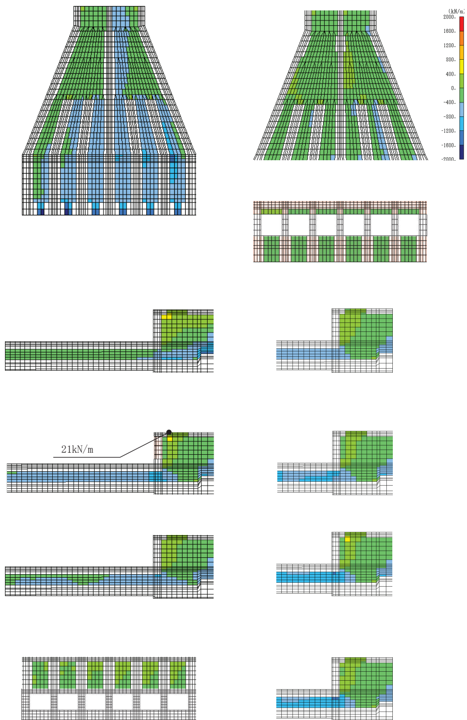
図 6-28(1) セン断破壊に対する照査値最大時の断面力分布図 (全応力解析) (せん断力 (kN/m) : Q_x ) (導流壁, 解析ケース①, 地震動 S_s - D2 (-+)) (標準部 t = 25.07s , 漸縮部 t = 25.06s )
