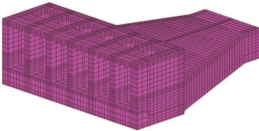
図 6-30 通水機能が要求される部材の範囲
