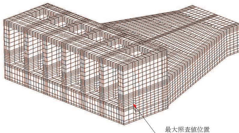
図 6-19 Ccb 工法適用部材におけるせん断破壊に対する最大照査値位置図
