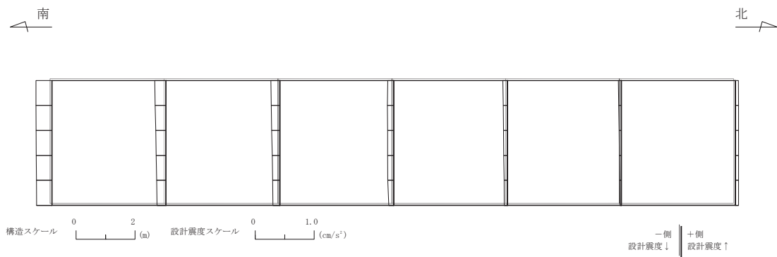
図 6-4(2) 作用荷重分布図 (設計震度分布) (有効応力解析) (解析ケース⑧, S_s - D2 (++) , B-B 断面 (漸縮部), t = 23.95s )
