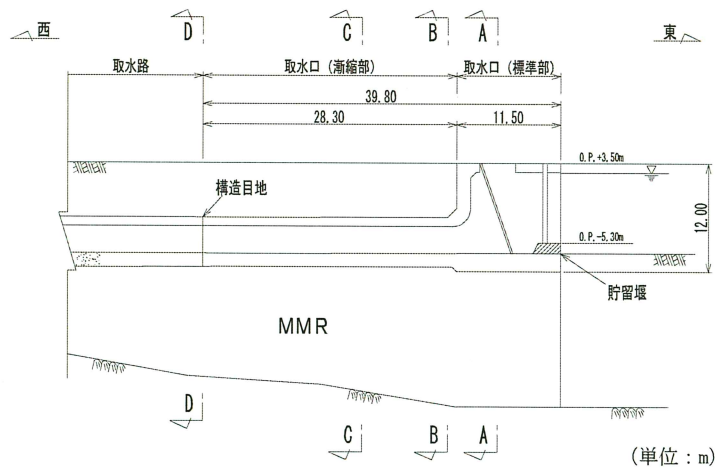
図 2-7 取水口断面図 (E-E 断面, 東西)
