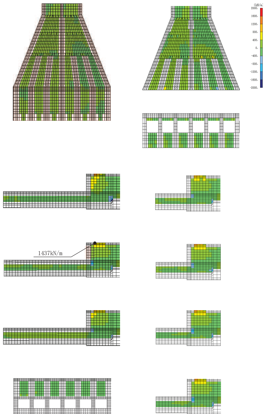
図 6-29 (1) せん断破壊に対する照査値最大時の断面力分布図 (全応力解析) (せん断力 (kN/m) : Q_y ) (導流壁, 解析ケース①, 地震動 S_s - D2 (-+) ) (標準部 t = 25.07s , 漸縮部 t = 25.06s )
