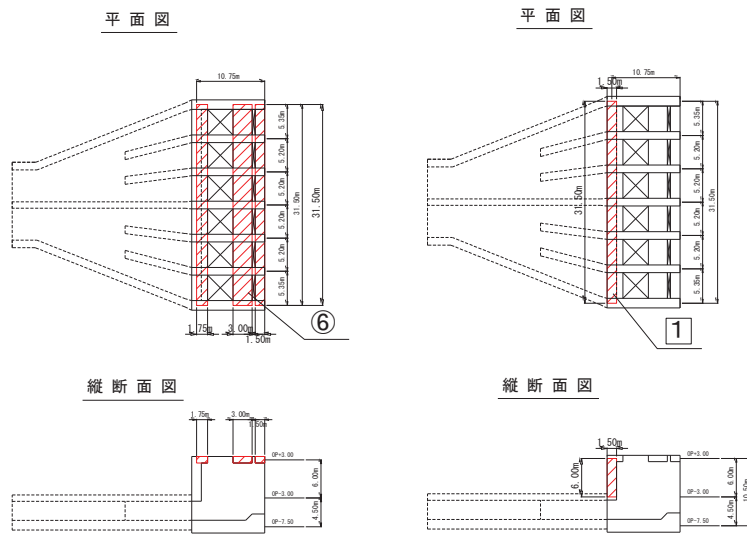
図3-11(3) 取水路（標準部）の等価剛性モデル（はり部材番号⑥，平面応力要素①）
