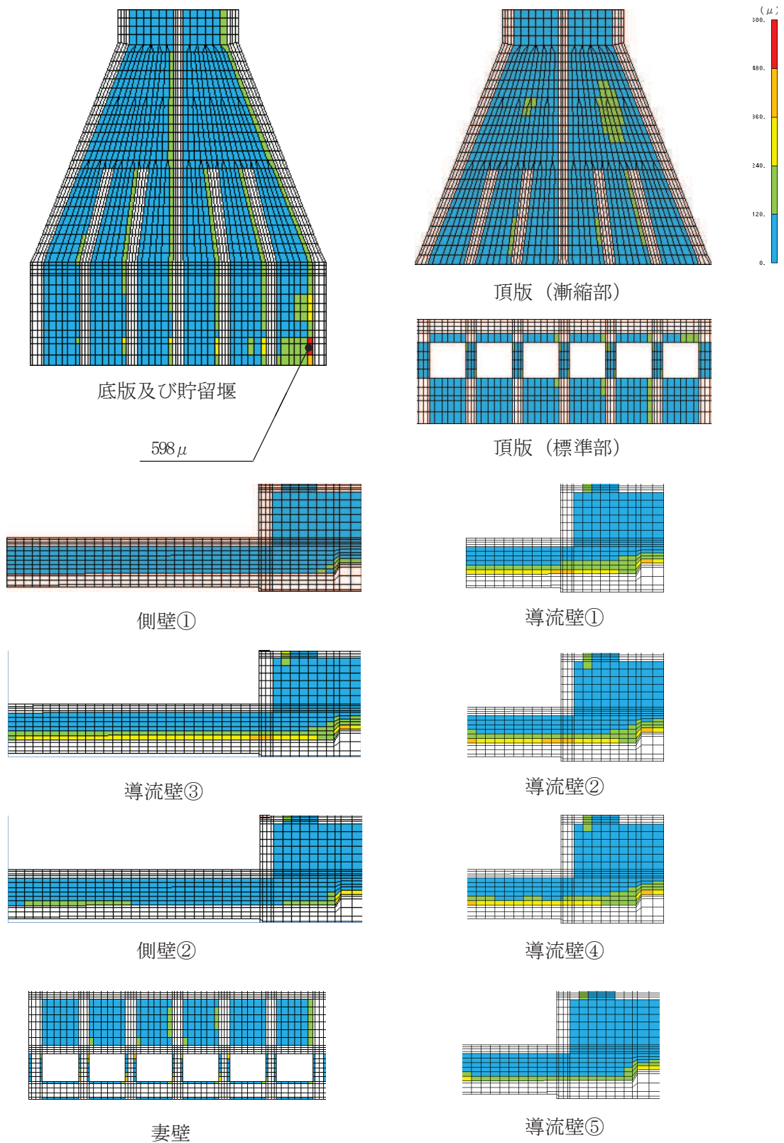
図 6-20(2) 曲げ・軸力系の破壊に対する照査値最大時のひずみ分布図（有効応力解析）
