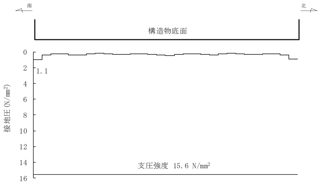
図 6-35(2) MMR (既設) の最大接地圧分布図 (有効応力解析) (解析ケース⑦, S s - D 2 (++) , B-B 断面 (漸縮部))
