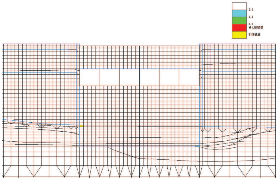
図 6-42 MMR (既設) の引張応力最大時刻の局所安全係数 (解析ケース①, 地震動 S_s - F 3 (++) , A-A 断面 (標準部), t = 28.59 s)
