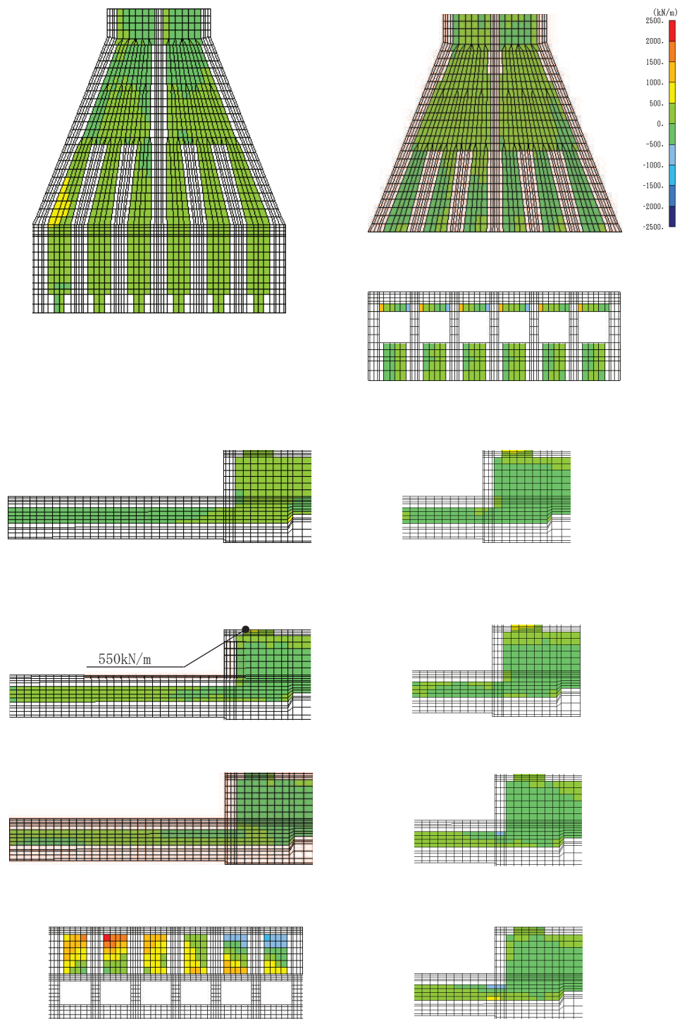
図 6-27(1) せん断破壊に対する照査値最大時の断面力分布図 (全応力解析) (軸力 (kN/m) : N_y ) (導流壁, 解析ケース①, 地震動 S_s - D2 (-+)) ((標準部 t = 25.07s , 漸縮部 t = 25.06s )
