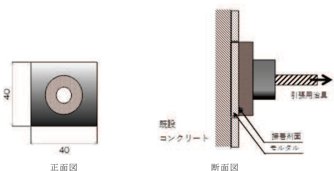
図 3-3 試験概要図
