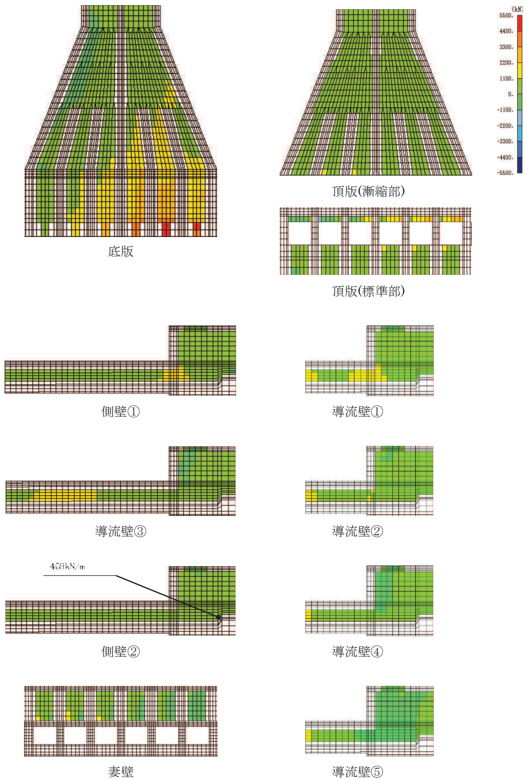
図 6-26 (2) せん断破壊に対する照査値最大時の断面力分布図 (有効応力解析)
