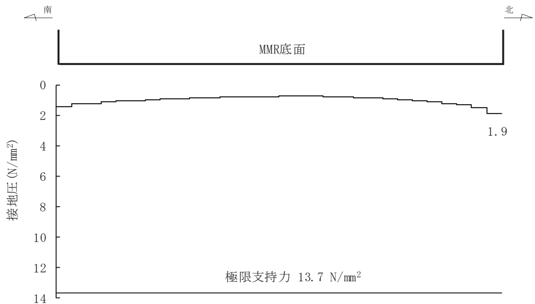
図 6-33(1) 基礎地盤の最大接地圧分布図（全応力解析） （解析ケース③，S s - N 1（++），B-B断面（漸縮部））
