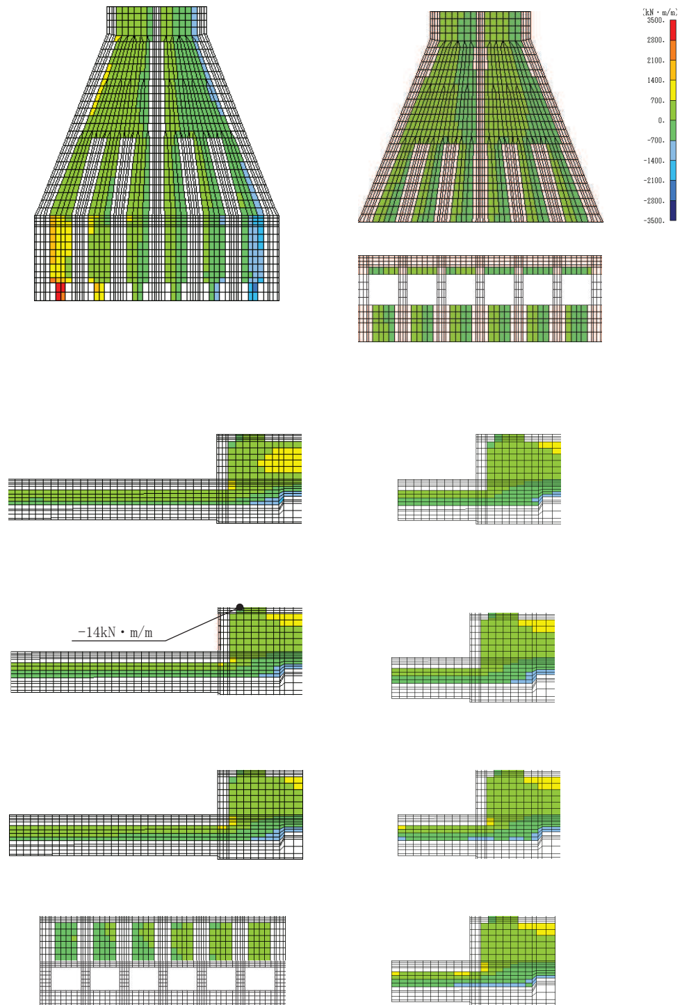
図 6-24(1) セン断破壊に対する照査値最大時の断面力分布図 (全応力解析) (曲げモーメント (kN・m/m) : M x ) (導流壁, 解析ケース①, 地震動 S s -D 2 (-+)) (標準部 t = 25.07s, 漸縮部 t = 25.06s)
