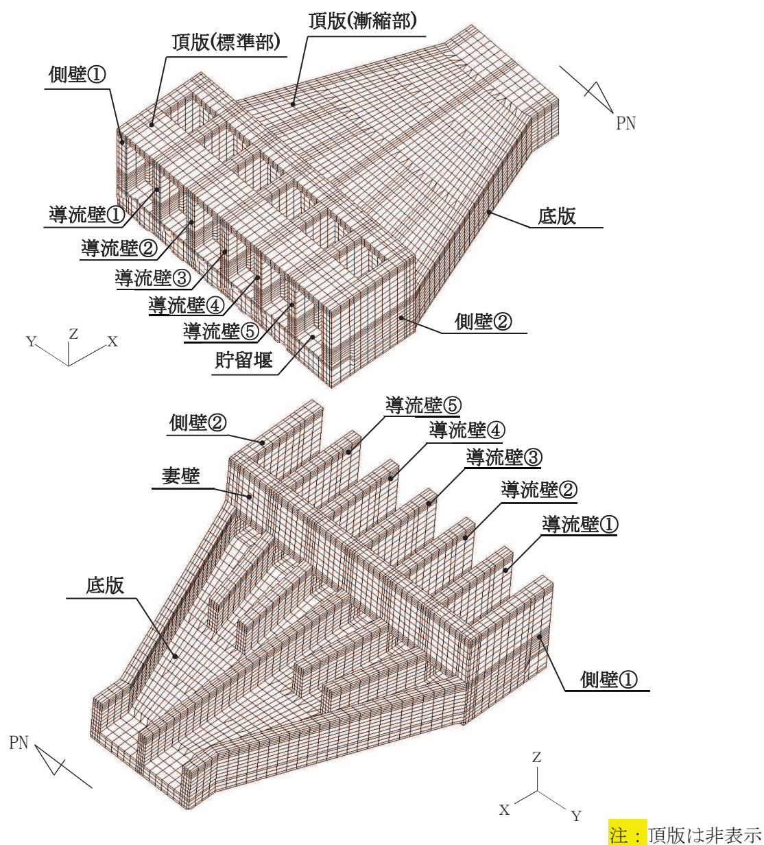
図6-13 各部材位置
