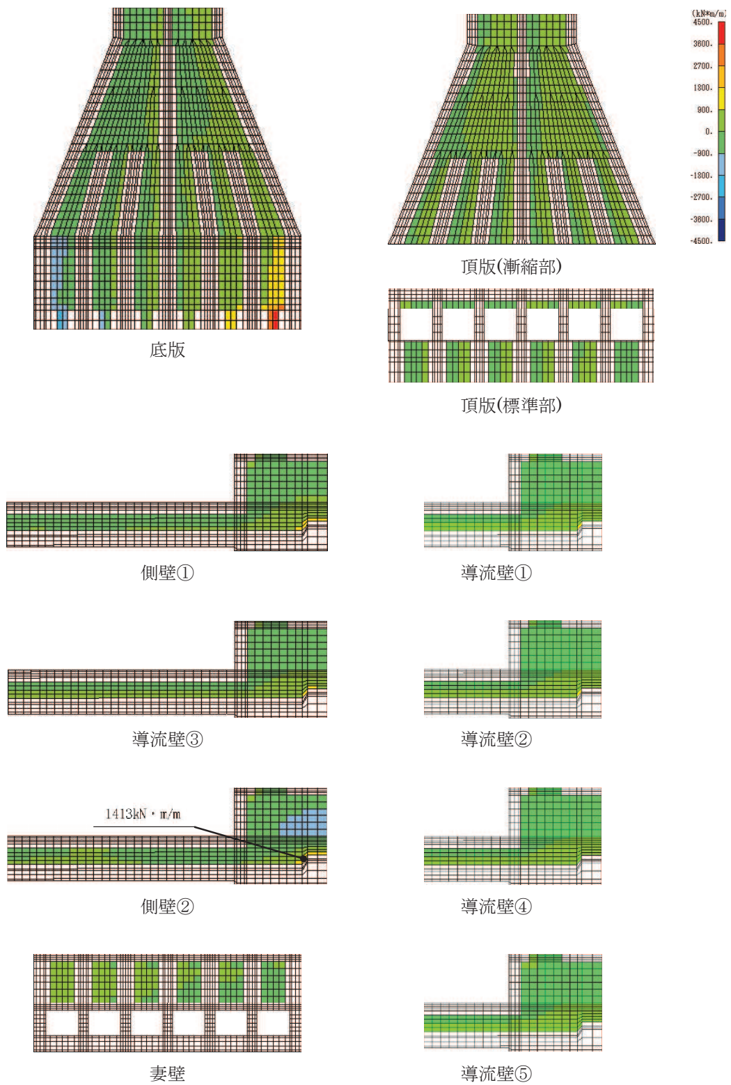
図 6-24(2) せん断破壊に対する照査値最大時の断面力分布図 (有効応力解析)
