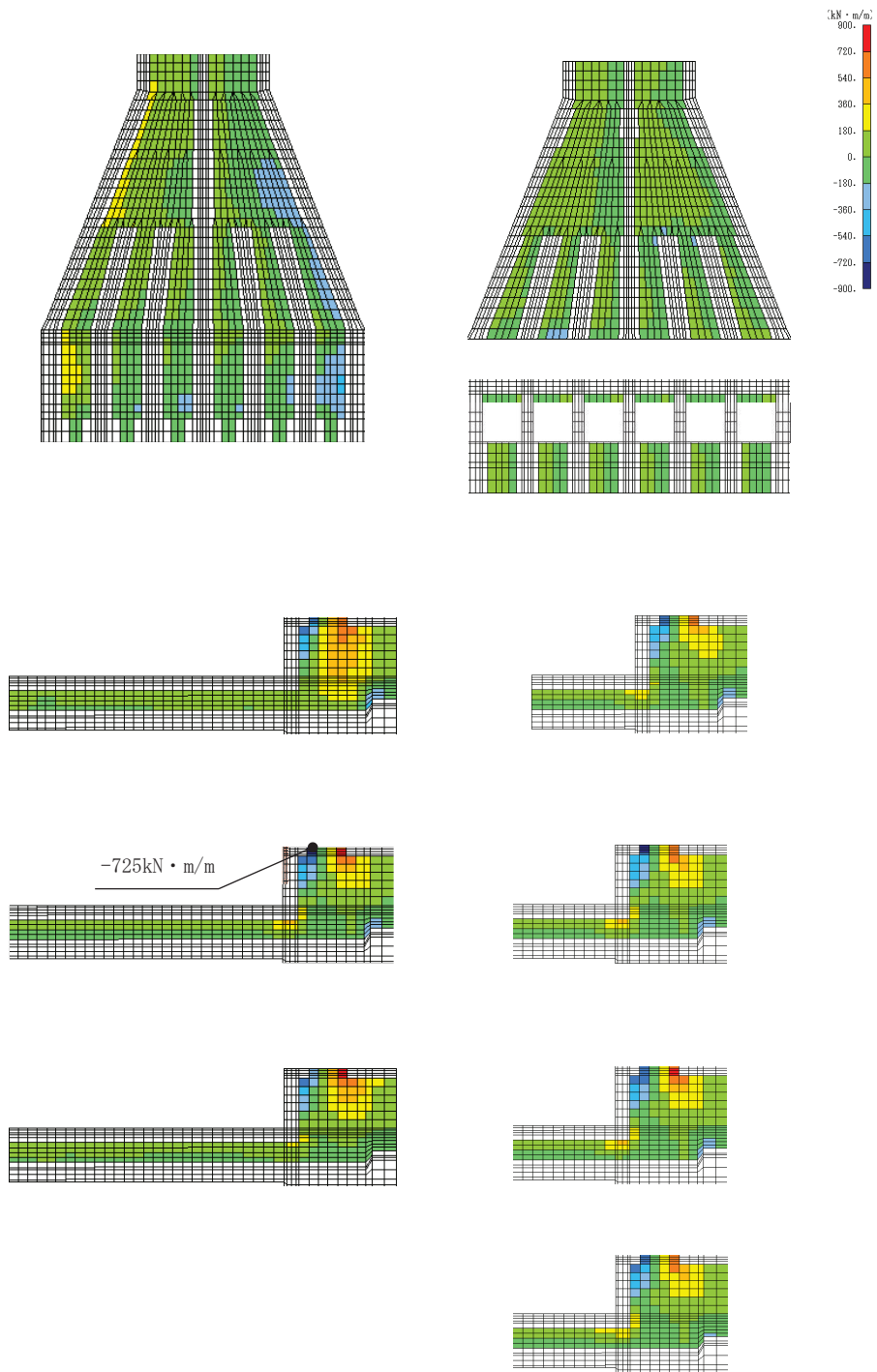
図 6-25(1) せん断破壊に対する照査値最大時の断面力分布図 (全応力解析) (曲げモーメント ( \text{kN} \cdot \text{m/m} ) : M_y ) (導流壁, 解析ケース①, 地震動 S_s - D2 (-+)) (標準部 t = 25.07\text{s} , 漸縮部 t = 25.06\text{s} )
