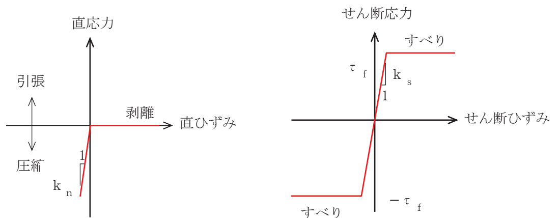
図 3-17 ジョイント要素の力学特性
