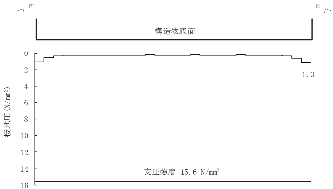
図 6-34(2) MMR (既設) の最大接地圧分布図 (有効応力解析) (解析ケース⑧, S s -D 2 (++) , B-B 断面 (標準部))
