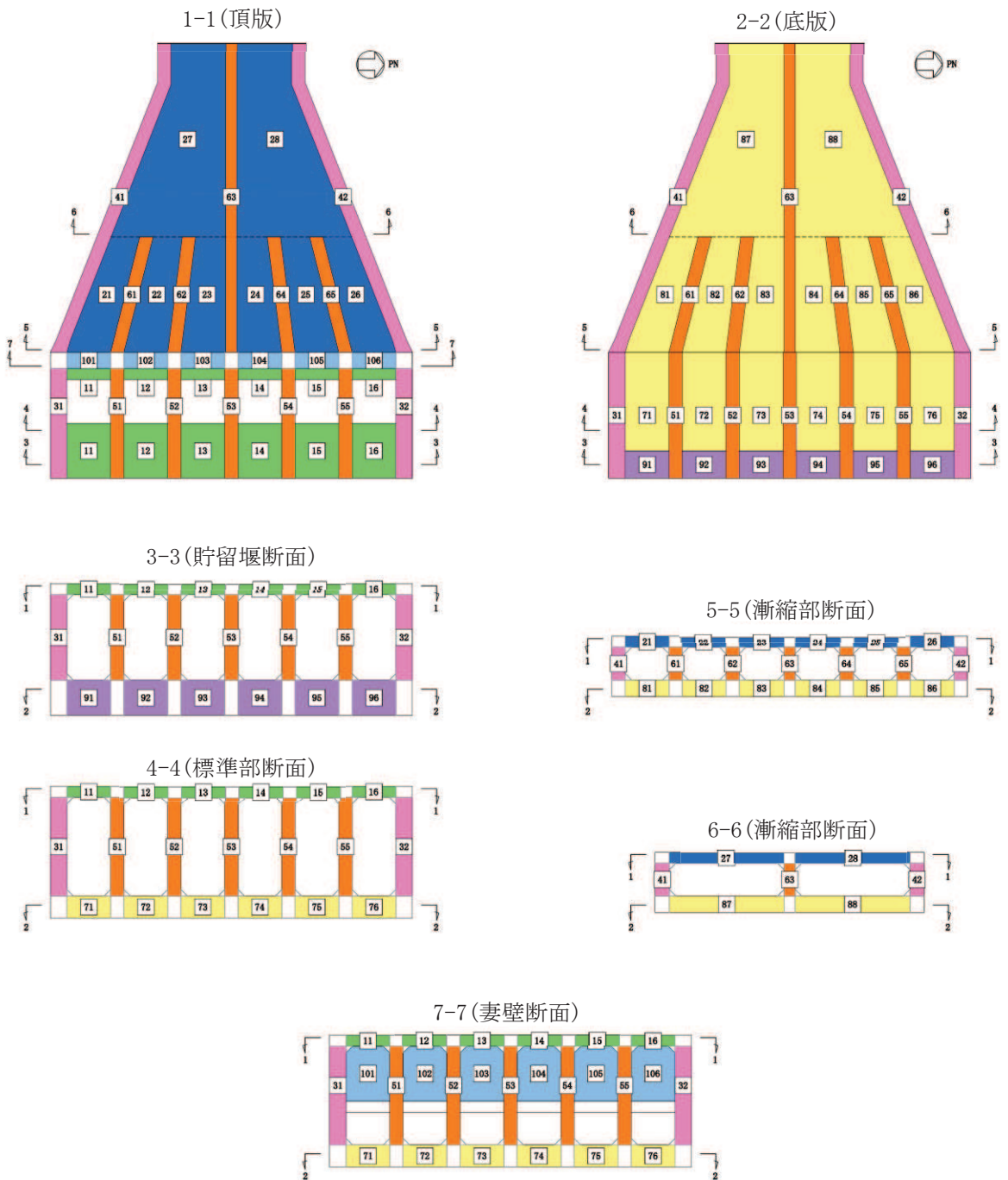
図 6-23 評価位置図 (曲げ・軸力系の破壊及びせん断破壊)
