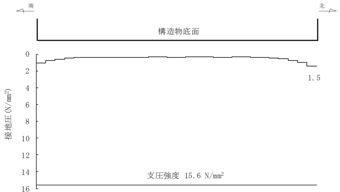
図 6-34 (1) MMR (既設) の最大接地圧分布図) (全応力解析) (解析ケース②, S s - D 2 (-+), A-A 断面 (標準部))
