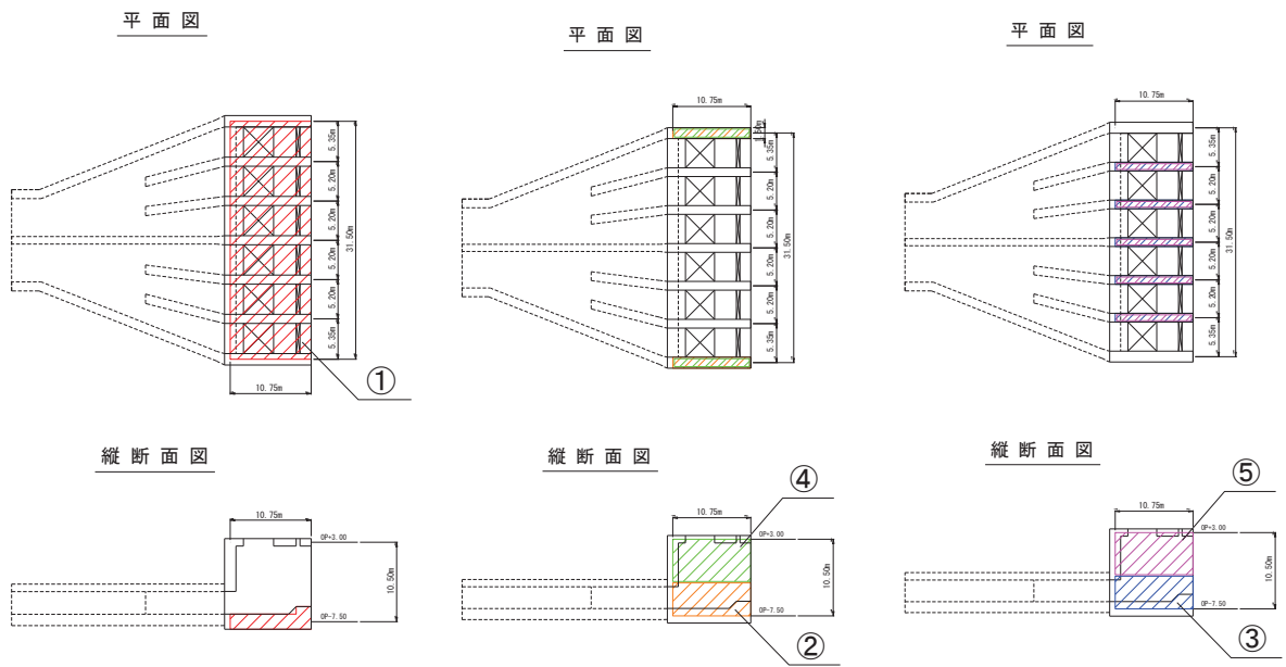
図3-11(2) 取水路（標準部）の等価剛性モデル（はり部材番号①，②，③，④，⑤）
