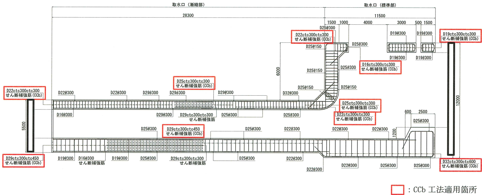
図 2-12 取水口，貯留堰側配筋図 (E-E断面，東西)
