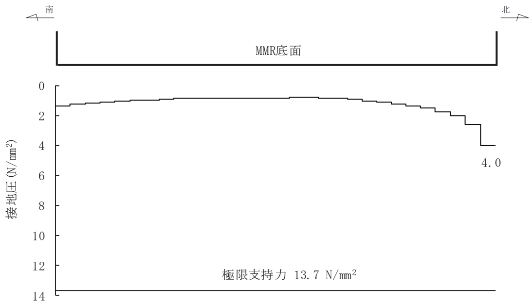
図 6-32(2) 基礎地盤の最大接地圧分布図（有効応力解析） （解析ケース⑧，S s - D 2（++），A-A 断面（標準部））
