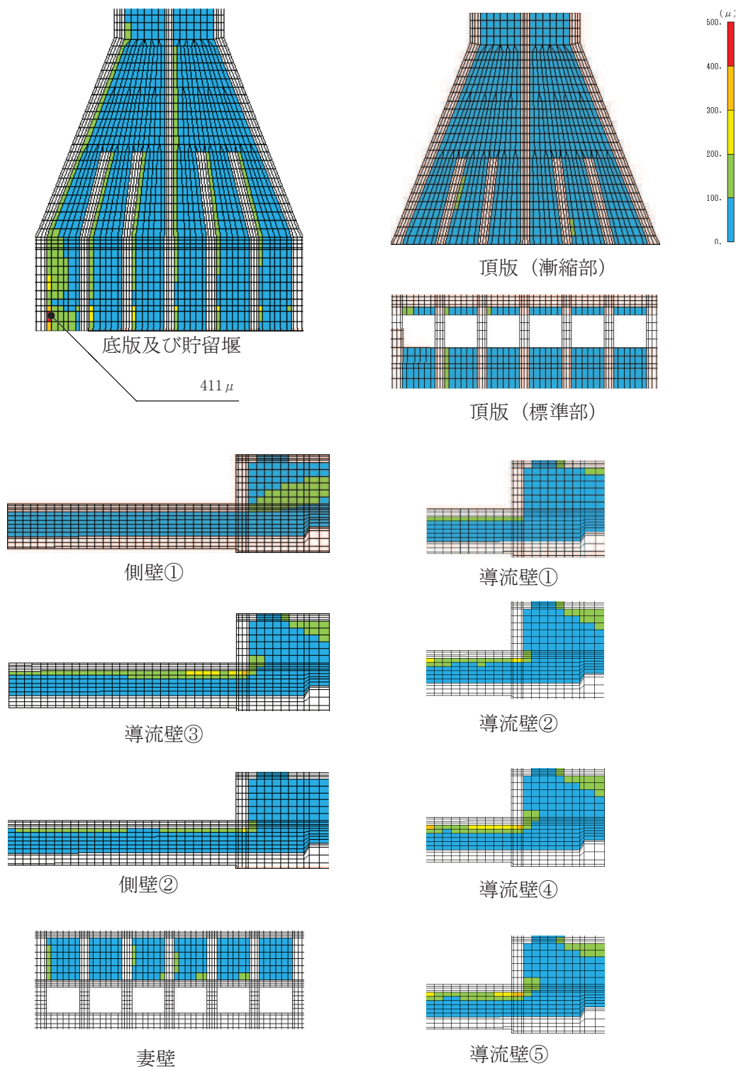
図 6-21 (1) 曲げ・軸力系の破壊に対する照査値最大時のひずみ分布図 (コンクリートの圧縮ひずみ：全応力解析) (貯留堰，解析ケース③，地震動 S_s - D2 (-+) ) (標準部 t = 25.08s ，漸縮部 t = 25.06s )
