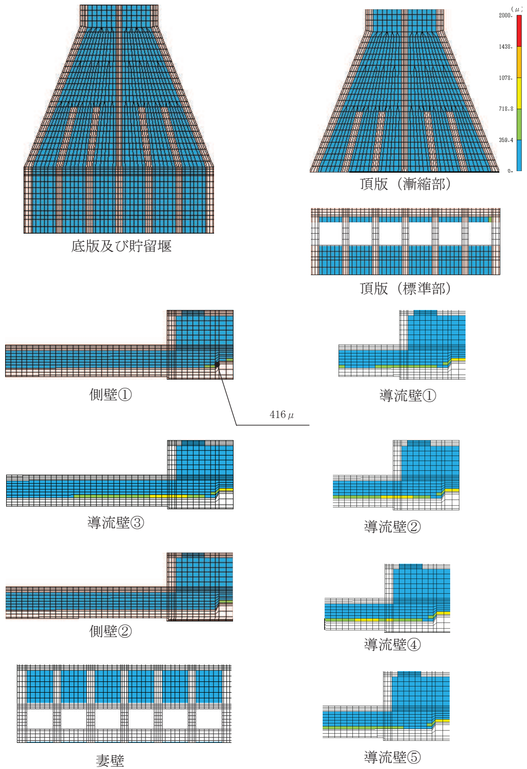
図 6-22(1) 曲げ・軸力系の破壊に対する照査値最大時のひずみ分布図 (鉄筋：全応力解析) (側壁，解析ケース③，地震動 S_s - D2 (-+) ) (標準部 t = 25.08s ，漸縮部 t = 25.06s )
