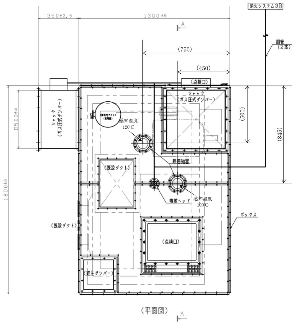
図-1.6-2 ボックス No. 2 の形状及びボックスに設置する機器の配置図
