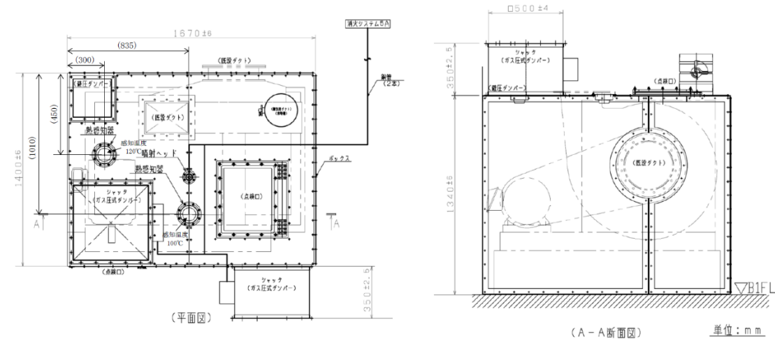
図-1.6-5 ボックス No. 5 の形状及びボックスに設置する機器の配置図
