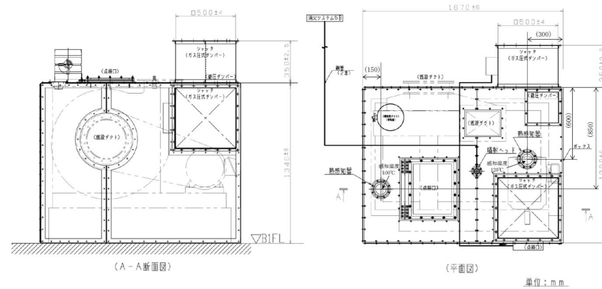
図-1.6-6 ボックス No. 6 の形状及びボックスに設置する機器の配置図
