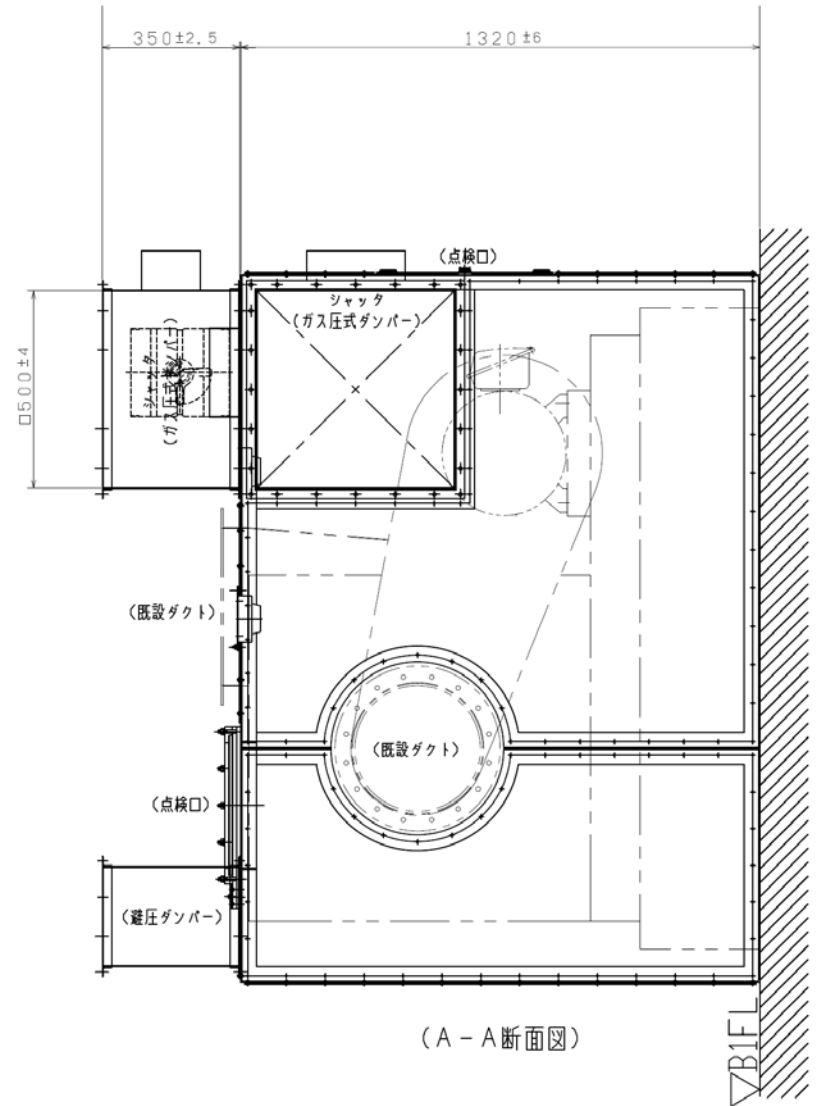
図-1.6-2 ボックス No. 2 の形状及びボックスに設置する機器の配置図
