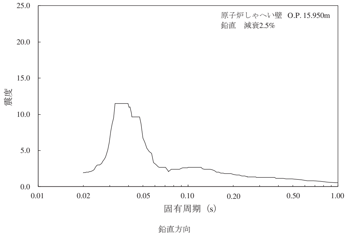
図 1-3 弁の動的機能維持に適用する床応答曲線
