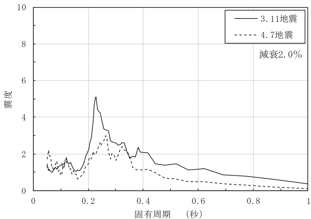
原子炉格納容器 O.P. 14. 295 水平方向
