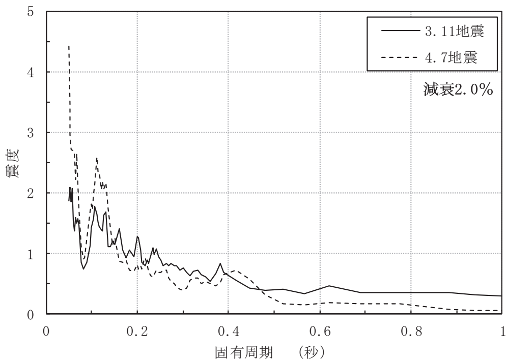
原子炉压力容器 O.P.9.334 鉛直方向
