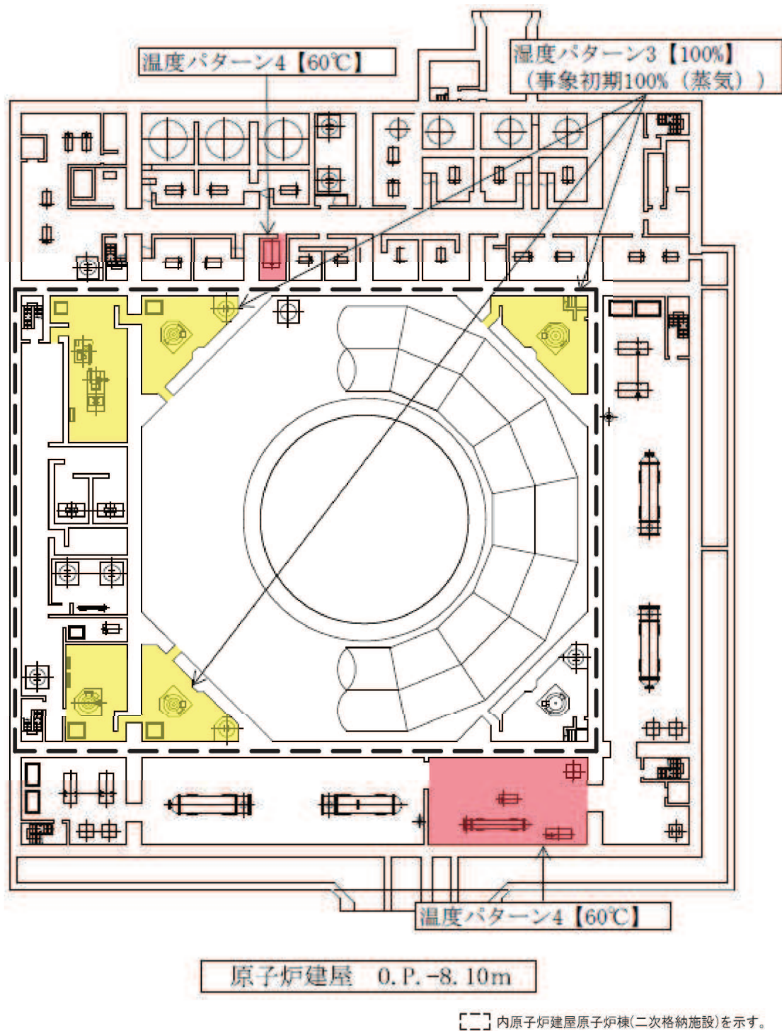
図1 重大事故等対処設備の環境条件設定 (1/7)
