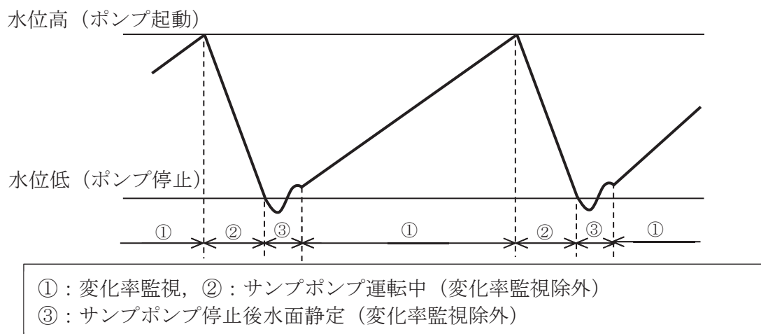
図2-2 ドライウェル床ドレンサンプ水位測定装置の演算時間
