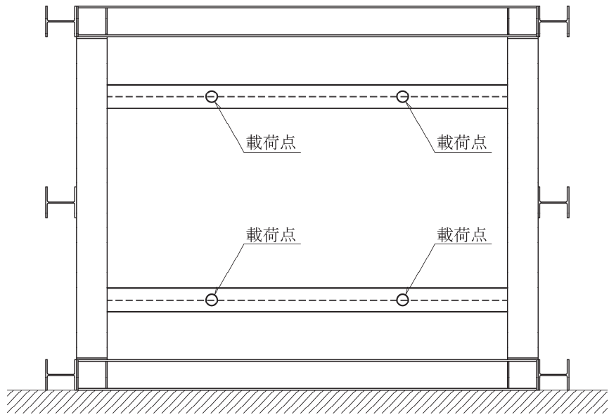
試験用架構図
