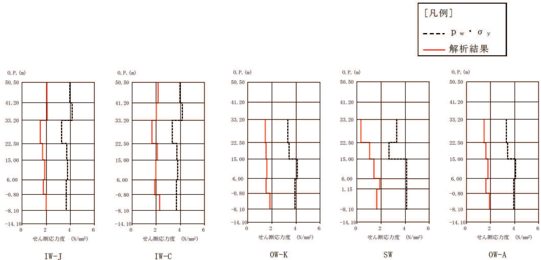
3.11地震時の耐震壁のせん断応力度(原子炉建屋, NS方向)
