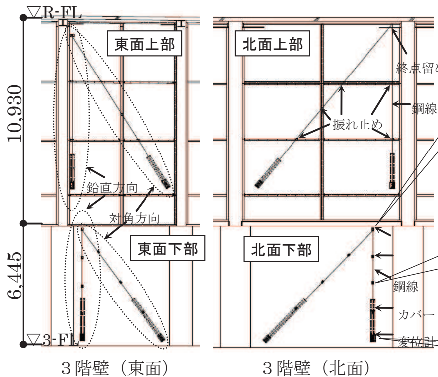
変位計測システムの設置詳細
