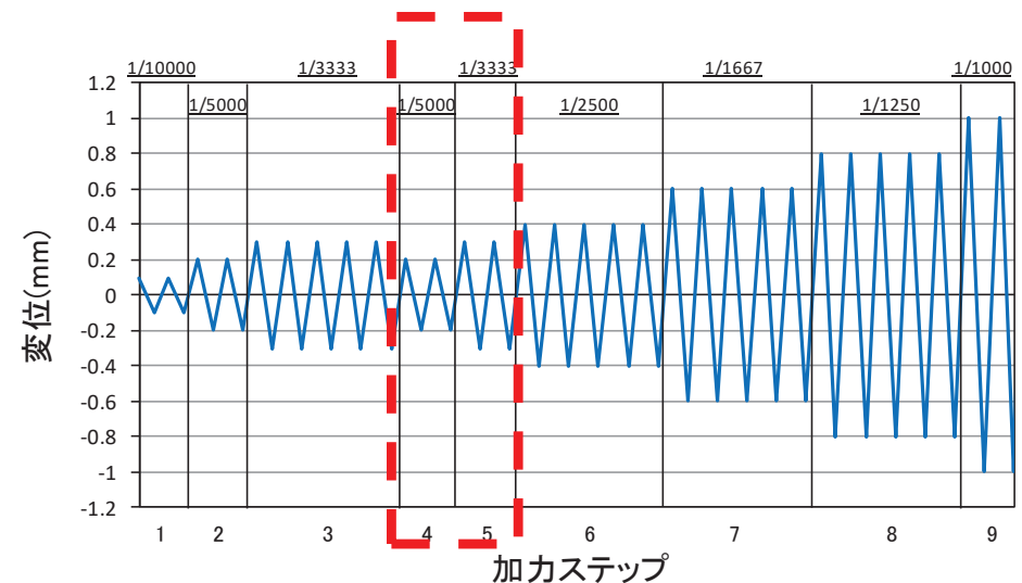
加力概念図
