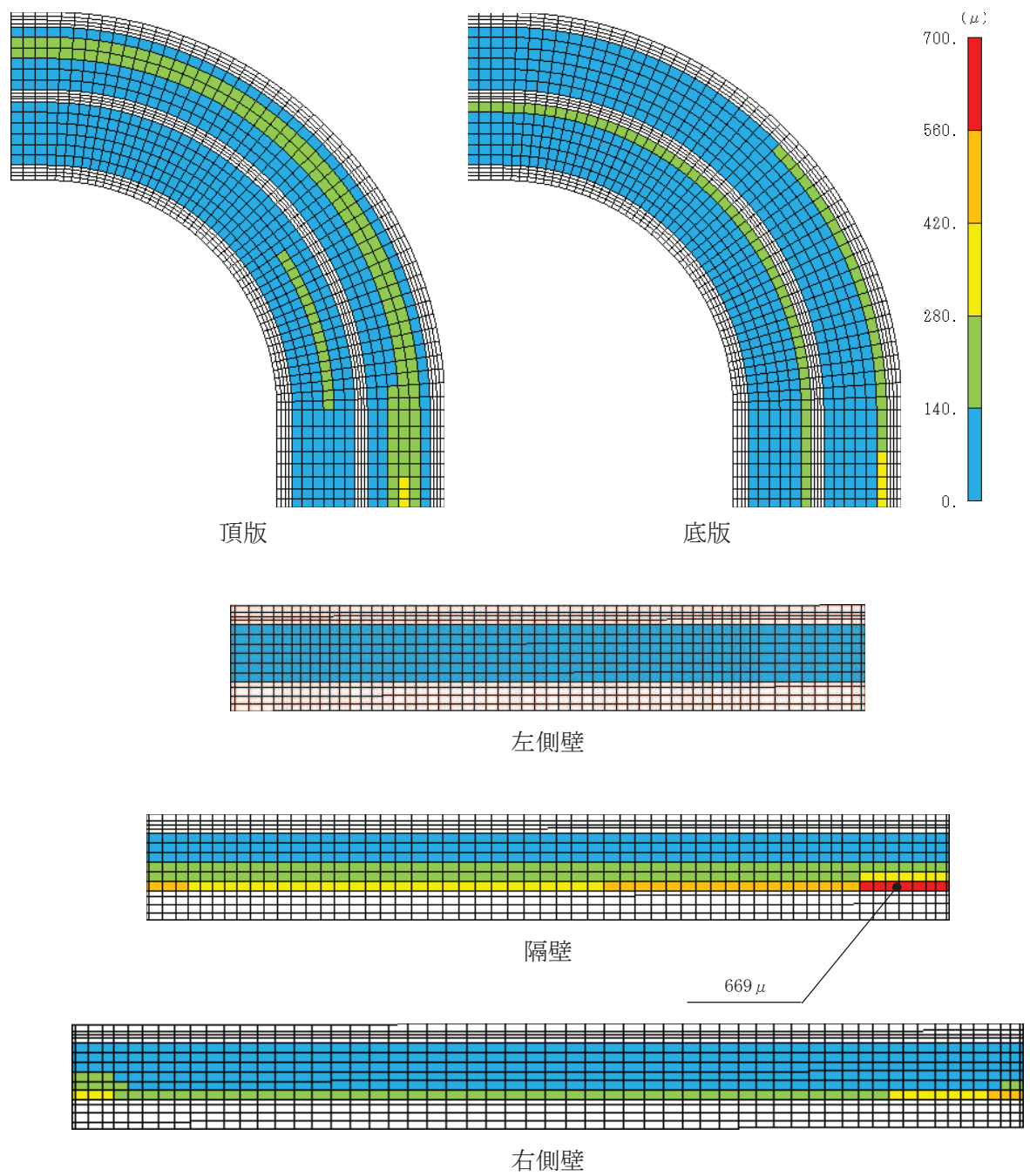
図 6-27 曲げ・軸力系の破壊に対する照査値最大時のひずみ分布図 (コンクリートの圧縮縁ひずみ) (曲線部, 隔壁, 解析ケース③, S s - N 1 (-+))
