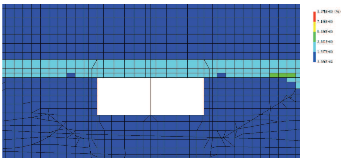
(b) 構造物周辺拡大図
