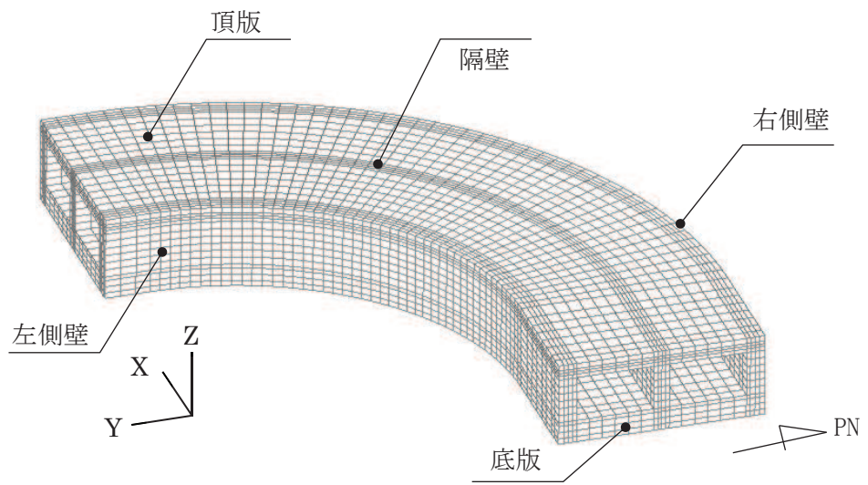
(a) 鳥瞰圖
