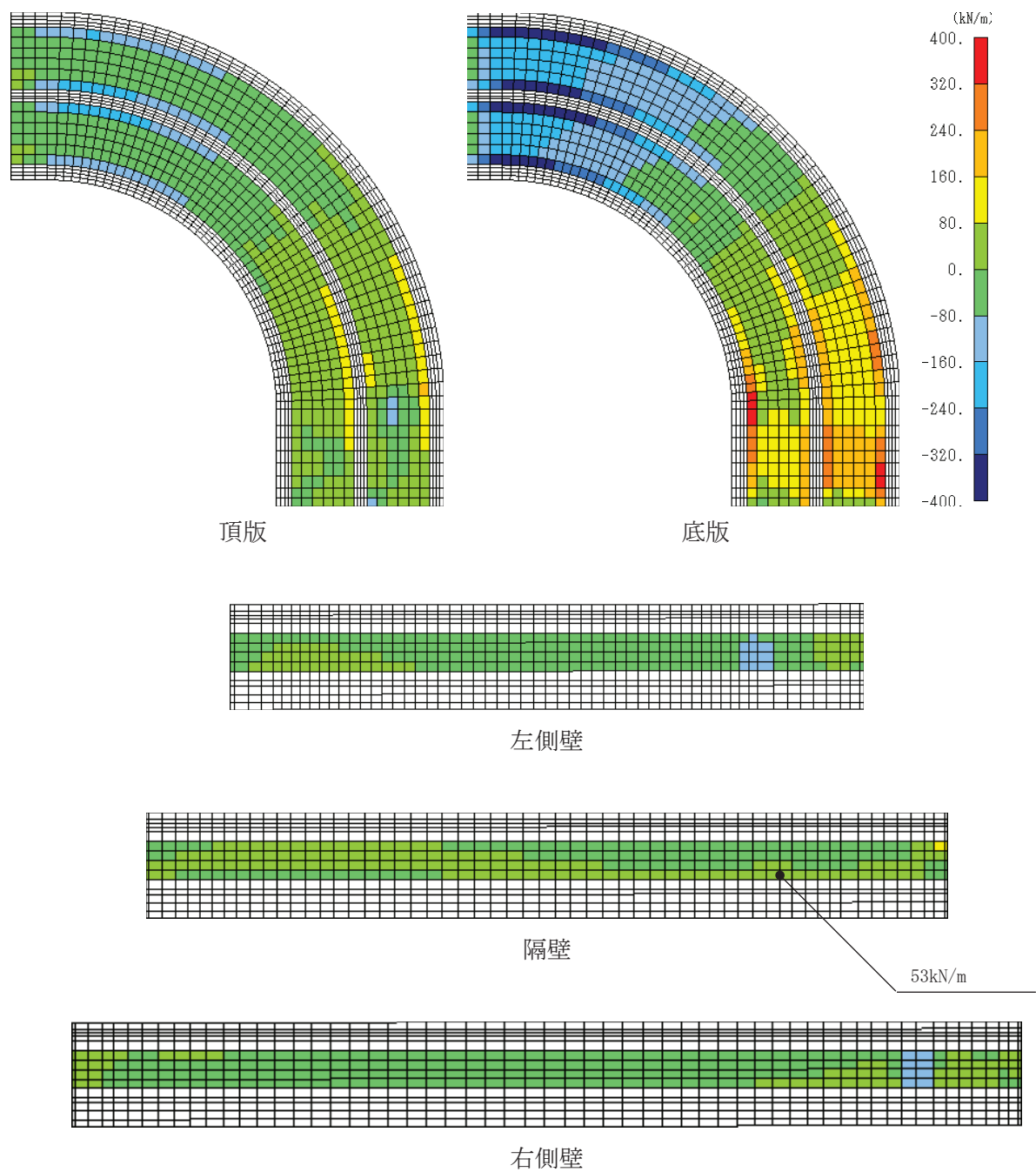
図 6-41 せん断破壊に対する照査値最大時の断面力分布図 (せん断力 (kN/m) : Q_y ) (曲線部, 隔壁, 解析ケース③, S_s - N1 (-+))
