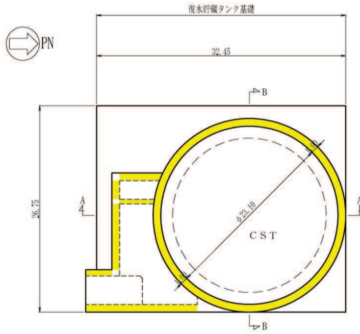
図 5-16(1) CCBによる耐震補強箇所 (平面図) (再掲)
