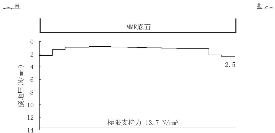
図 6-47 基礎地盤の最大接地圧分布図（断面⑤） （解析ケース③，S s -N1（-+））
