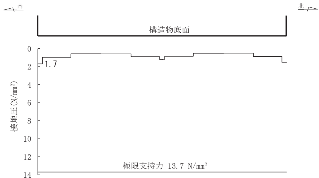
図 6-49 基礎地盤の最大接地圧分布図（断面⑦） （解析ケース①，S s -D1（-+））
