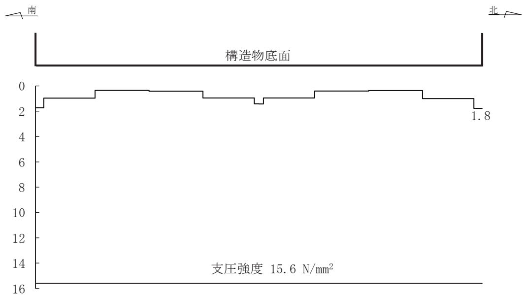
図 6-52 MMR (既設) の最大接地圧分布図 (断面④)
