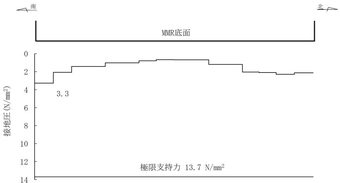
図 6-45 基礎地盤の最大接地圧分布図（断面③）
