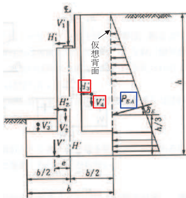
図4-18 仮想背面を考慮した地震時の荷重状態
