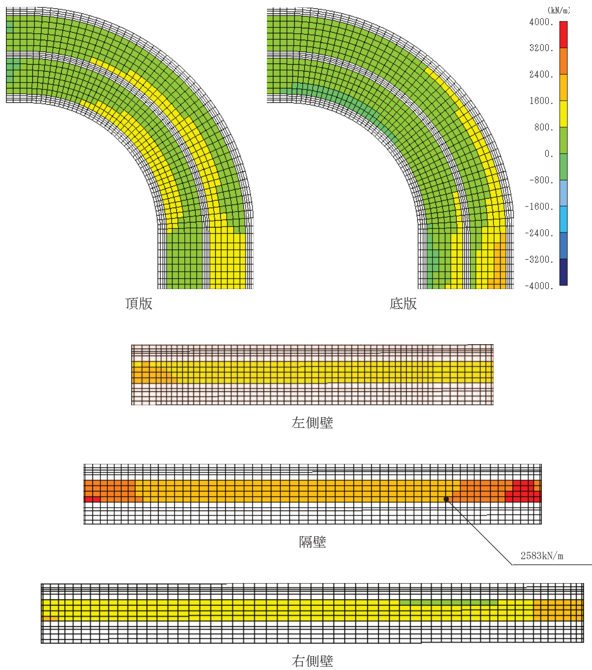
図 6-38 せん断破壊に対する照査値最大時の断面力分布図 (軸力 (kN/m) : N_x ) (曲線部, 隔壁, 解析ケース③, S_s - N_1 (-+))
