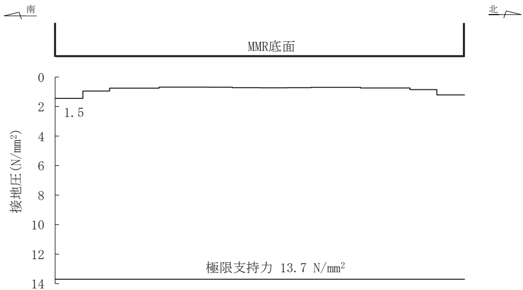
図 6-48 基礎地盤の最大接地圧分布図（断面⑥） （解析ケース①， S s -F3（++））
