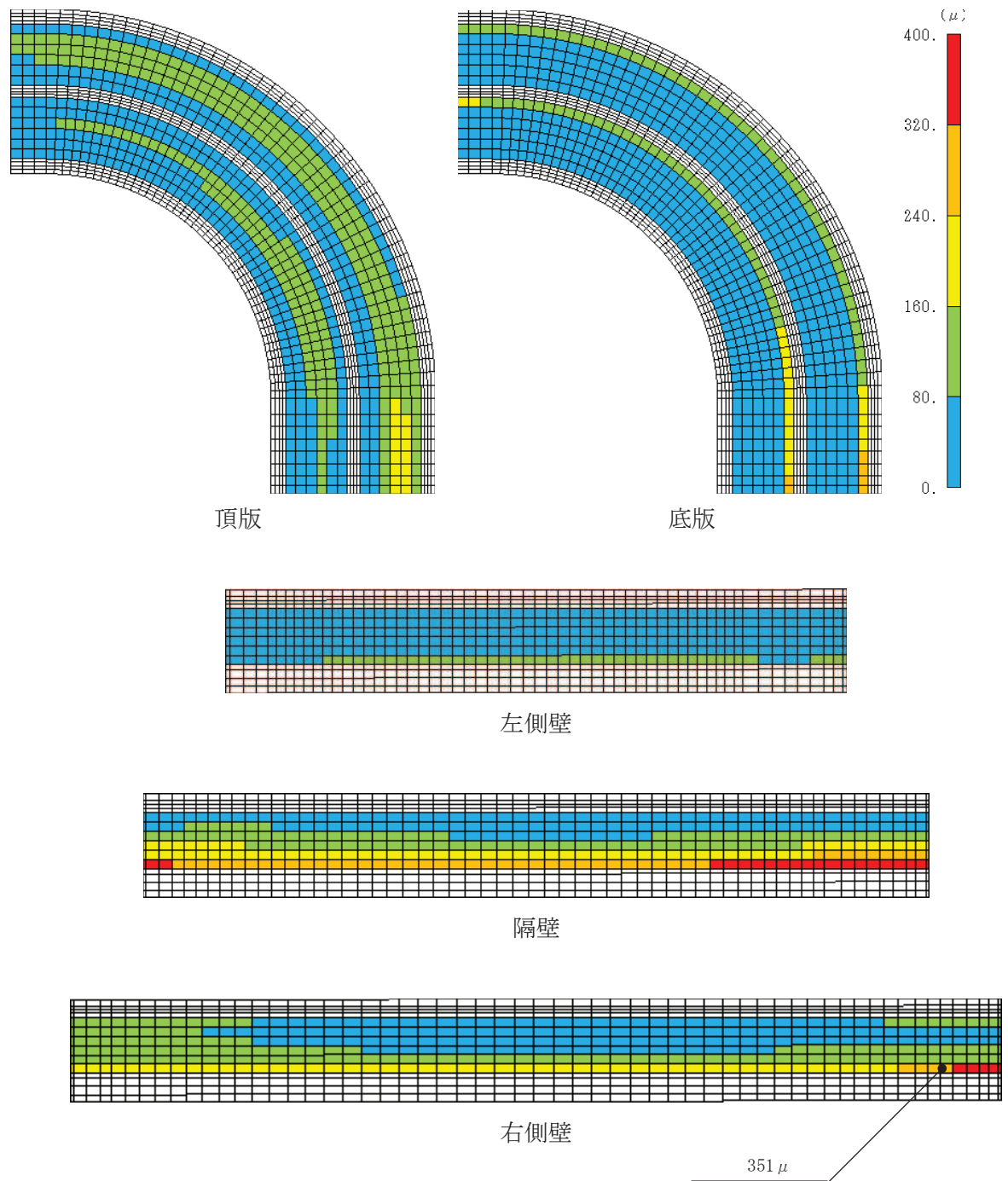
図 6-28 曲げ・軸力系の破壊に対する照査値最大時のひずみ分布図 (コンクリートの圧縮ひずみ) (曲線部, 右側壁, 解析ケース③, S s - N 1 (-+))
