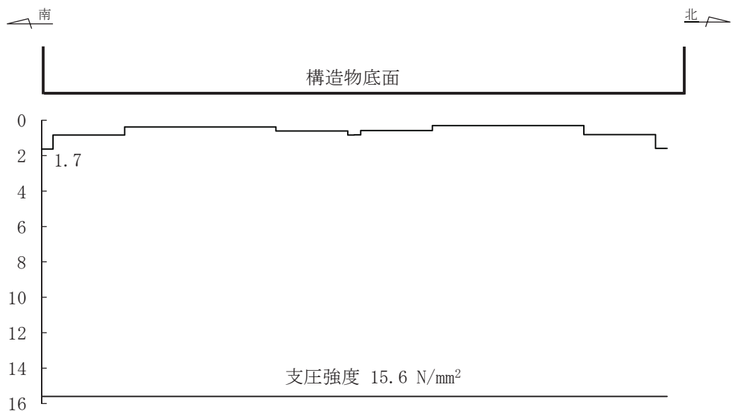
図 6-50 MMR (既設) の最大接地圧分布図 (断面②) (解析ケース①, S s -D2 (-+))
