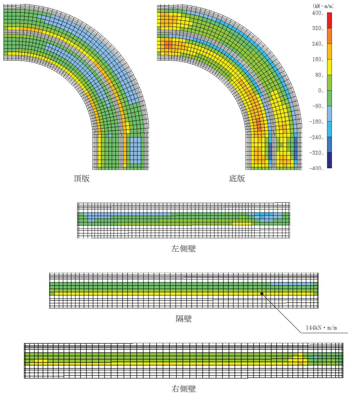
図 6-37 せん断破壊に対する照査値最大時の断面力分布図 (曲げモーメント (kN · m/m) : M_y ) (曲線部, 隔壁, 解析ケース③, S s - N 1 (-+))
