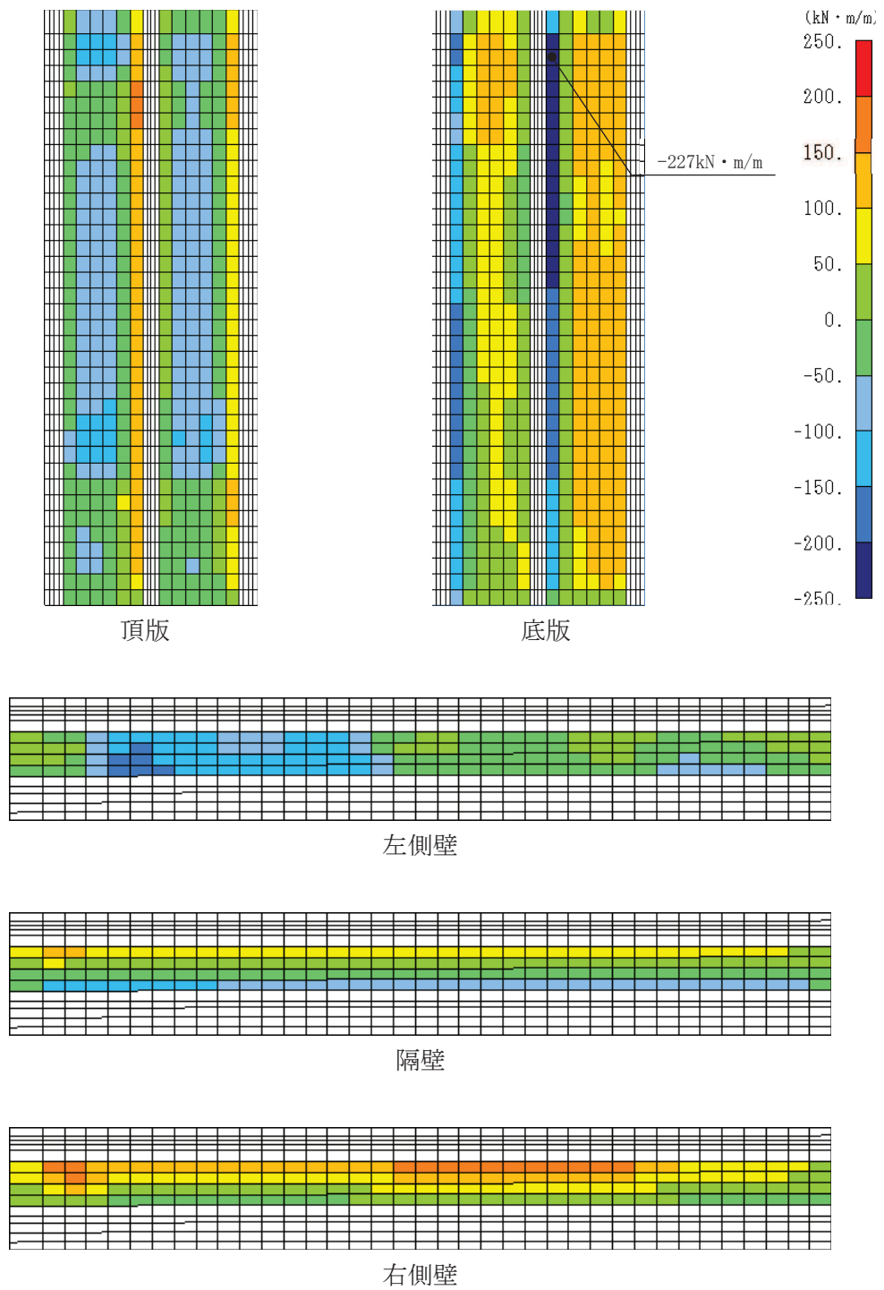
図 6-31 せん断破壊に対する照査値最大時の断面力分布図 (曲げモーメント ( \text{kN} \cdot \text{m}/\text{m} ) : M_y ) (直線部, 底版, 解析ケース③, S_s - N1 (++) )
