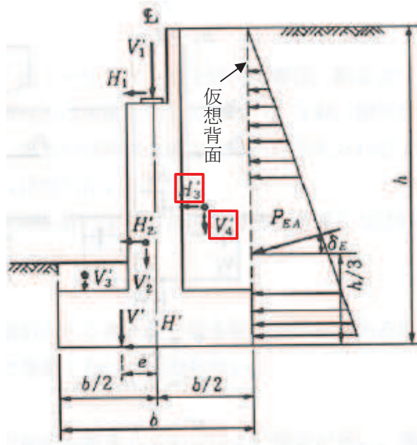
図 3-10 仮想背面を考慮した地震時の荷重状態
