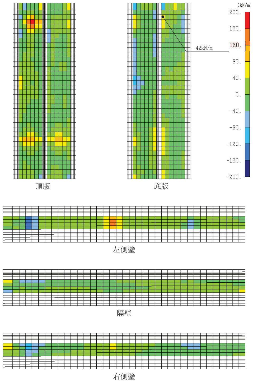
図 6-35 せん断破壊に対する照査値最大時の断面力分布図 (せん断力 (kN/m) : Q_y ) (直線部, 底版, 解析ケース③, S_s - N1 (++) )
