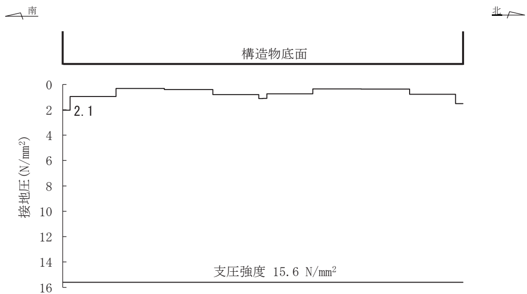
図 6-54 MMR (既設) の最大接地圧分布図 (断面⑥) (解析ケース③, S s -N1 (-+))
