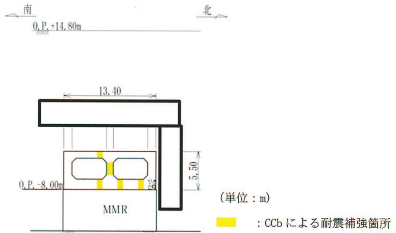
図 5-86(4) CCb による耐震補強箇所 (②断面, 曲線部; 取水口側) (再掲)
