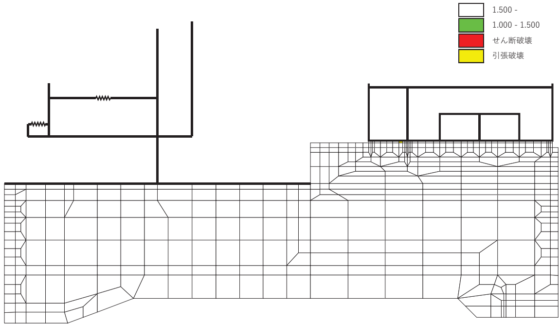
(a) 全体図
