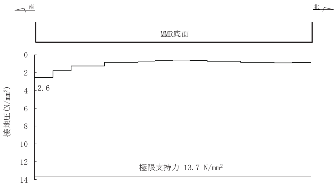
図 6-44 基礎地盤の最大接地圧分布図（断面②） （解析ケース①， S s -F2（++））
