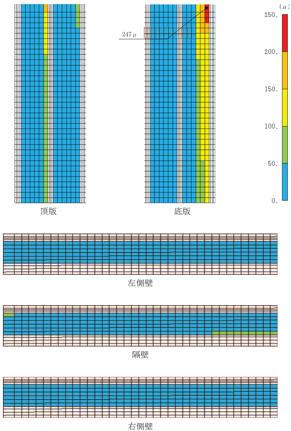
図 6-25 曲げ・軸力系の破壊に対する照査値最大時のひずみ分布図 (鉄筋) (直線部, 底板, 解析ケース③, S s - N 1 (++) )
