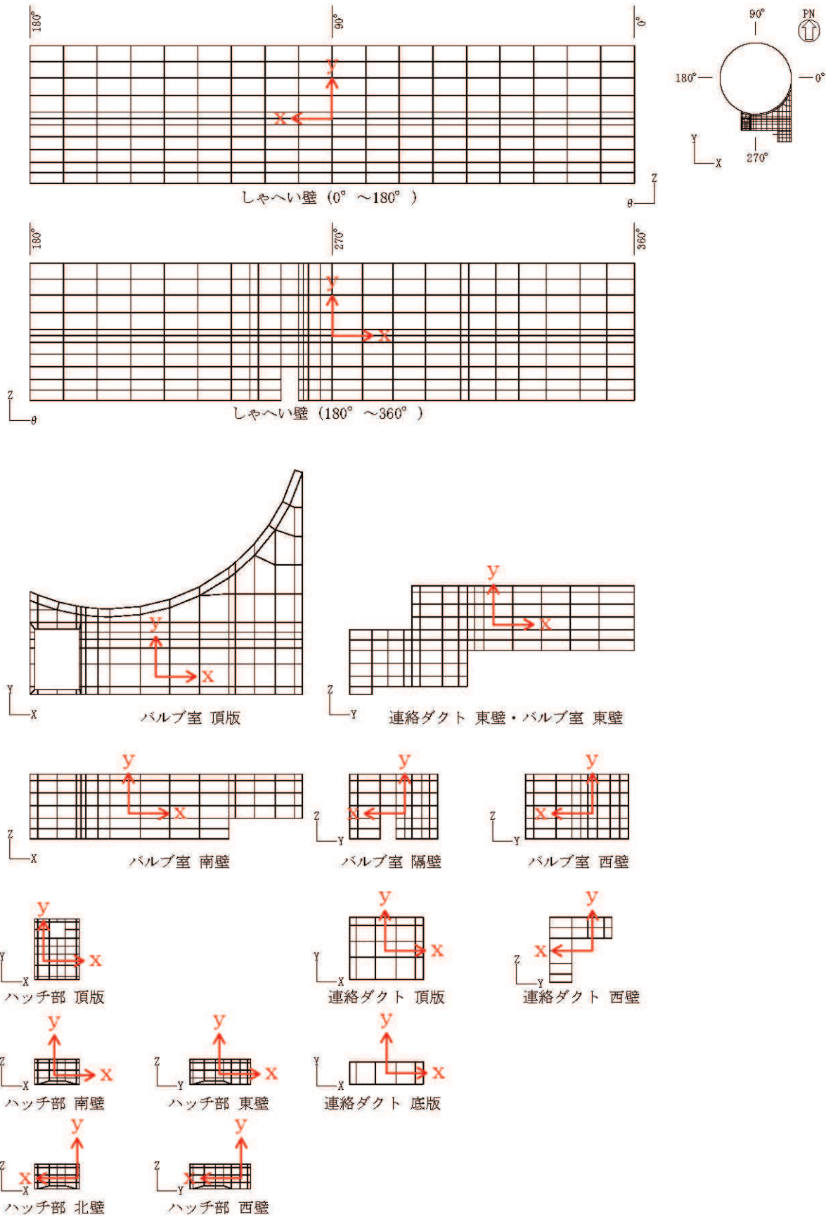
図 6-7(1) 各部材の要素座標系 (しゃへい壁, バルブ室及び連絡ダクト)
