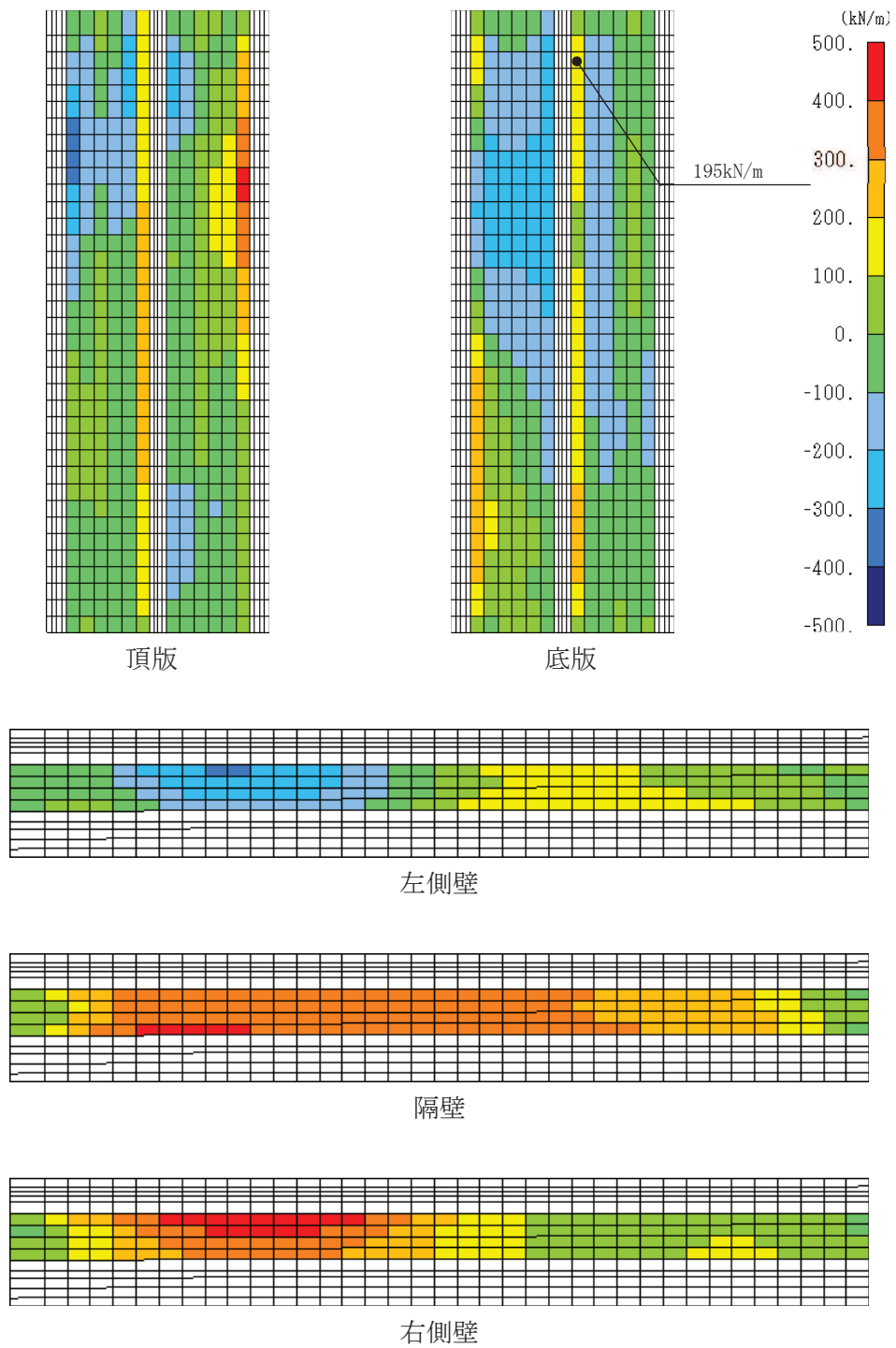
図 6-33 せん断破壊に対する照査値最大時の断面力分布図 (軸力 (kN/m) : N_y ) (直線部, 底版, 解析ケース③, S_s - N1 (++) )
