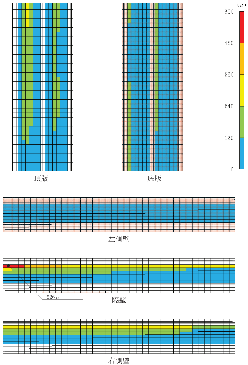
図 6-23 曲げ・軸力系の破壊に対する照査値最大時のひずみ分布図* (コンクリートの圧縮縁ひずみ) (直線部, 隔壁, 解析ケース③, S s - N 1 (++) )
