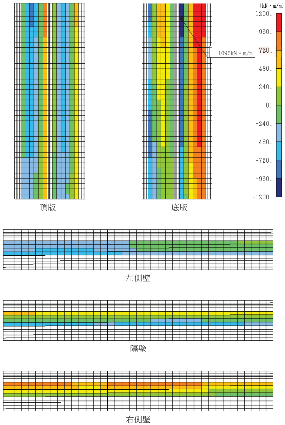
図 6-30 せん断破壊に対する照査値最大時の断面力分布図 (曲げモーメント ( \text{kN} \cdot \text{m}/\text{m} ) : M_x ) (直線部, 底版, 解析ケース③, S_s - N1 (++) )
