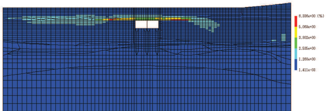
(a) 全体図
