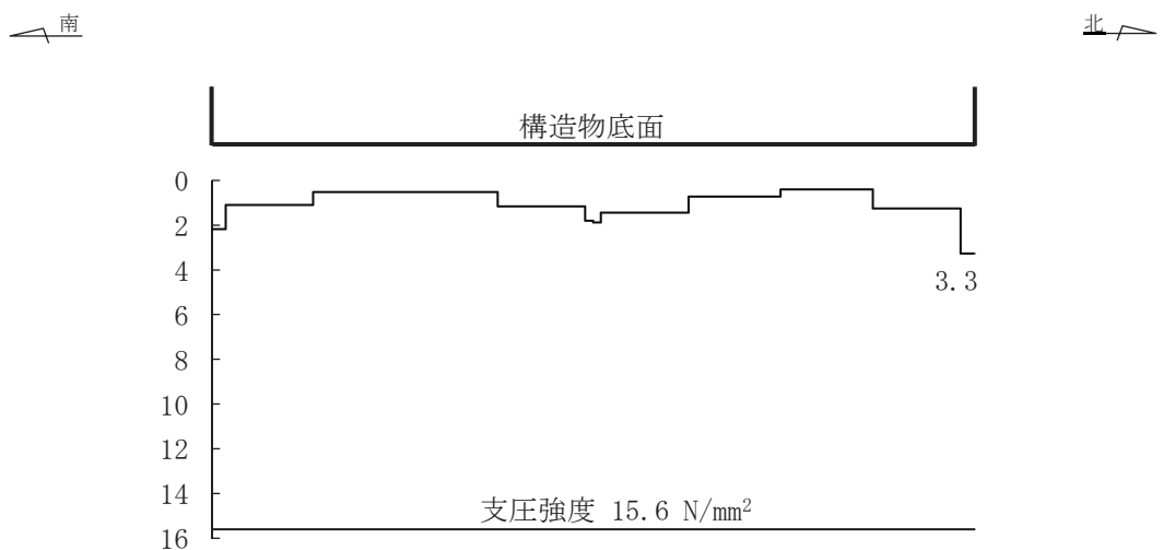
図 6-53 MMR (既設) 最大接地圧分布図 (断面⑤) (解析ケース③, S s -N1 (++) )
