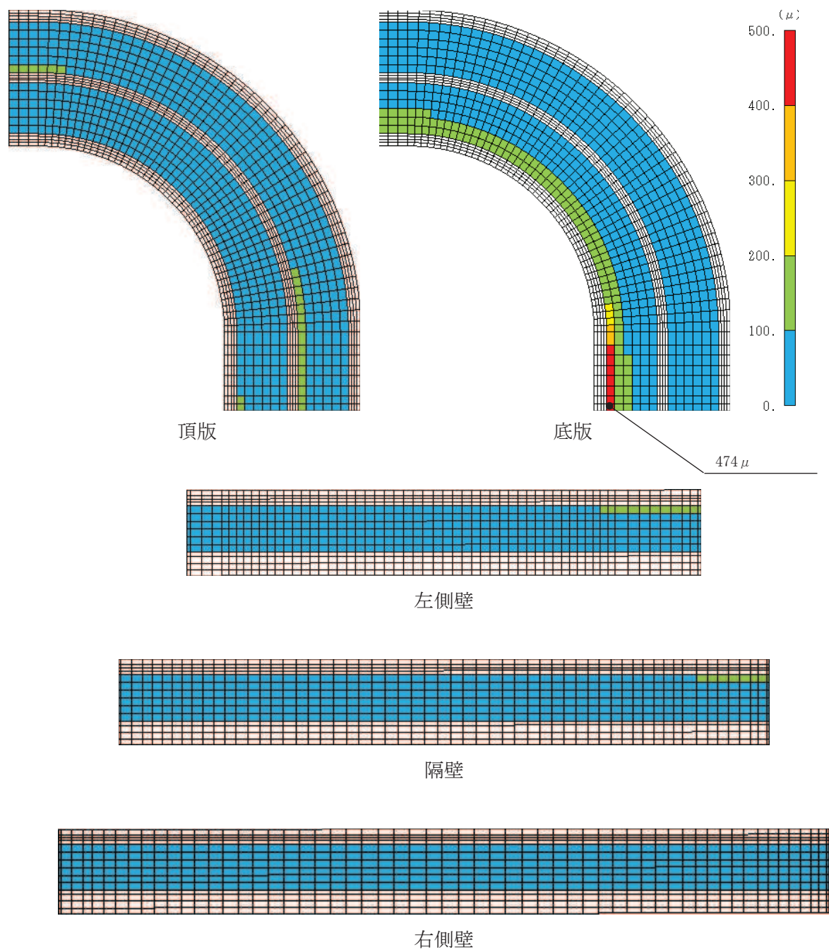
図 6-29 曲げ・軸力系の破壊に対する照査値最大時のひずみ分布図 (鉄筋) (曲線部, 底版, 解析ケース③, S_s - N1 (-+) )
