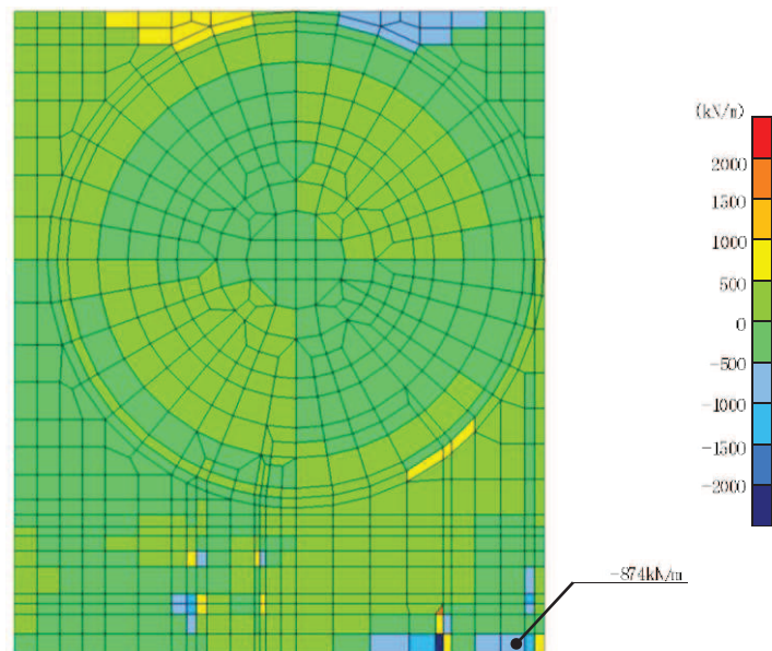
図 6-18(1) せん断破壊に対する照査値最大時の断面力分布図 (せん断力 (kN/m) : Q_x ) (解析ケース②, S s - D 2 (++) , t=6.86s , 南北)
