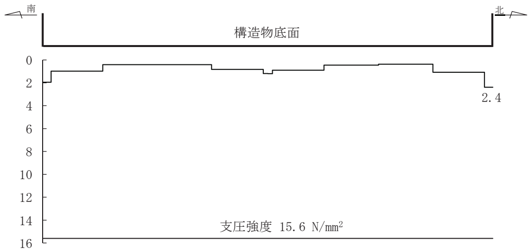
図 6-51 MMR (既設) の最大接地圧分布図 (断面③) (解析ケース①, S s -D1 (-+))
