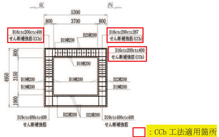
図 2-4(5) 復水貯蔵タンク基礎 概略配筋図 (4-4 断面)
