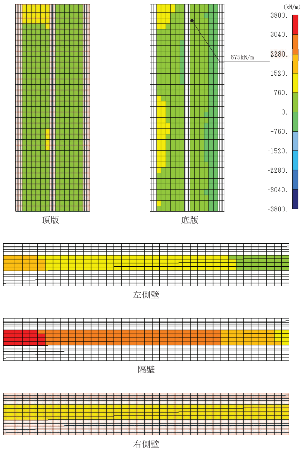
図 6-32 せん断破壊に対する照査値最大時の断面力分布図 (軸力 (kN/m) : N x ) (直線部, 底板, 解析ケース③, S s -N1 (++)
