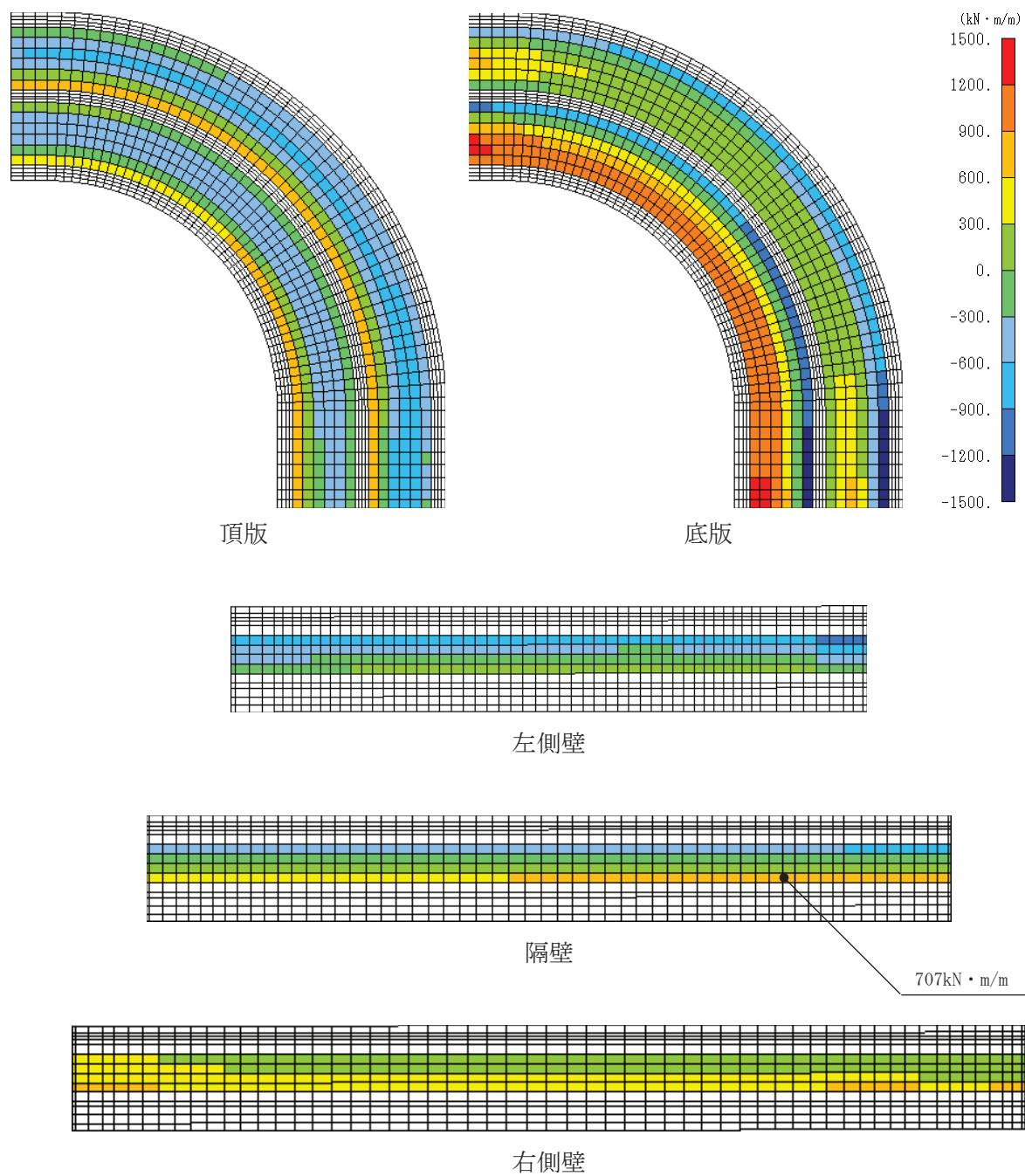
図 6-36 せん断破壊に対する照査値最大時の断面力分布図 (曲げモーメント ( \text{kN} \cdot \text{m}/\text{m} ) : M_x ) (曲線部, 隔壁, 解析ケース③, S s - N 1 (-+))
