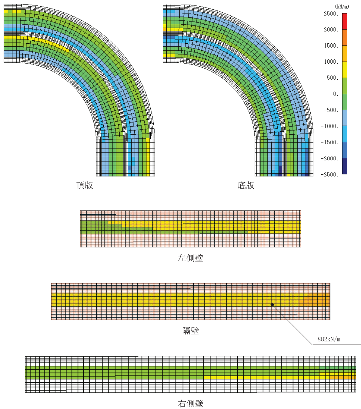
図 6-40 せん断破壊に対する照査値最大時の断面力分布図 (せん断力 (kN/m) : Q_x ) (曲線部, 隔壁, 解析ケース③, S_s - N1 (-+))
