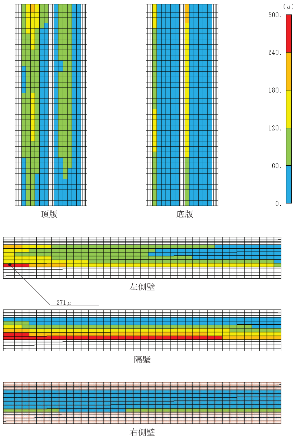
図 6-24 曲げ・軸力系の破壊に対する照査値最大時のひずみ分布図 (コンクリートの圧縮ひずみ) (直線部, 左側壁, 解析ケース③, S s - N 1 (++) )
