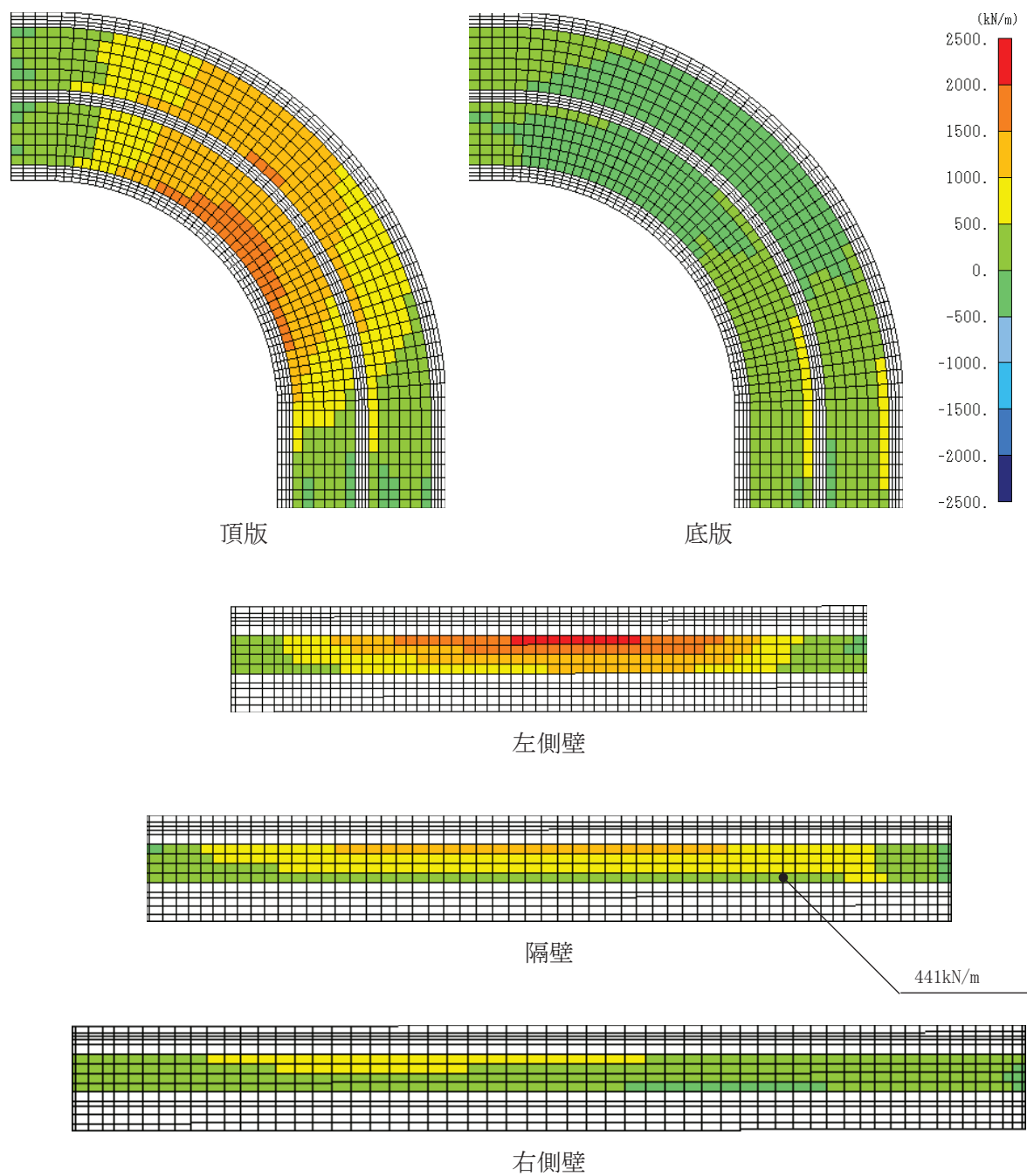
図 6-39 せん断破壊に対する照査値最大時の断面力分布図
