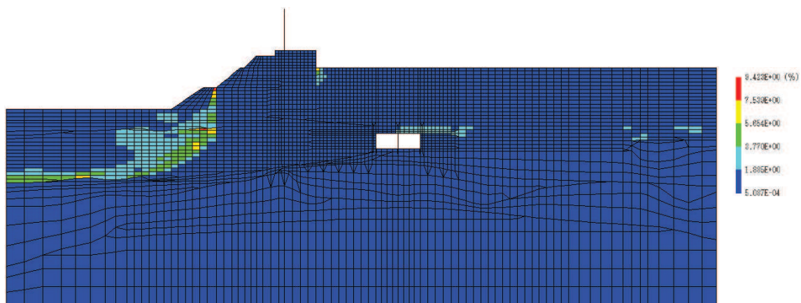
(a) 全体図
