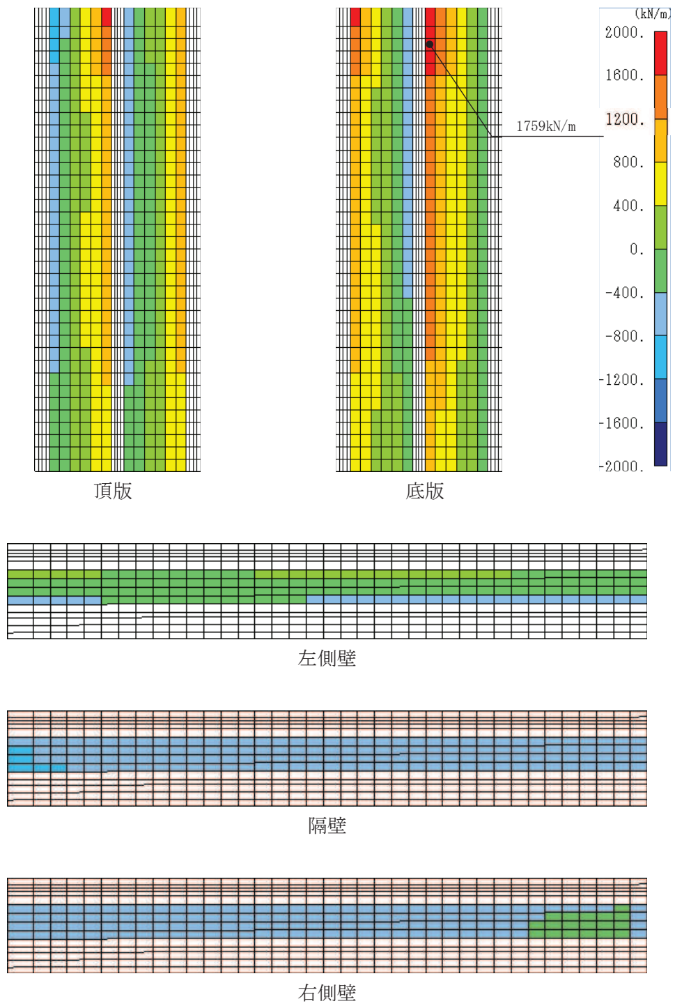
図 6-34 せん断破壊に対する照査値最大時の断面力分布図 (せん断力 (kN/m) : Q_x ) (直線部, 底板, 解析ケース③, S_s - N1 (++) )
