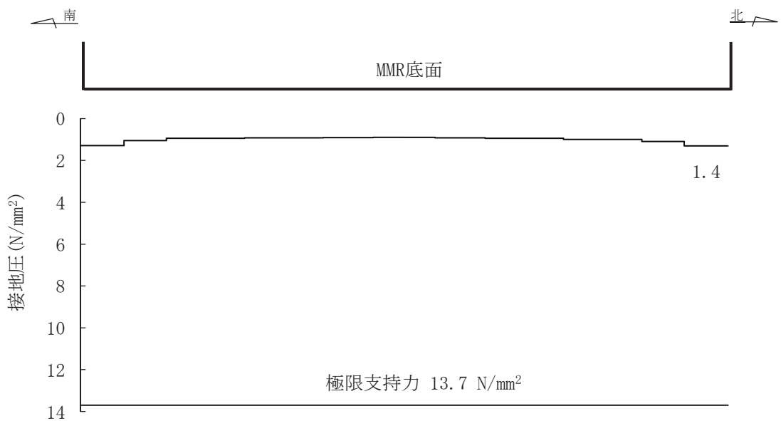
図 6-46 基礎地盤の最大接地圧分布図（断面④）
