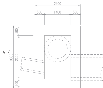
A-A 断面図
