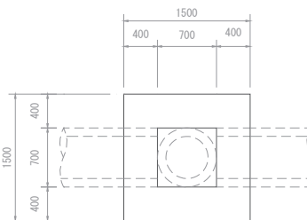
A-A 断面图
