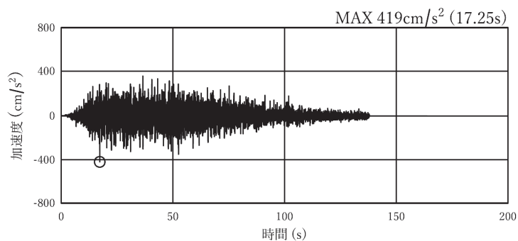
図 4-1(4) 加速度時刻歴波形（接続桧②）（鉛直方向：S s - D 1 : 解析ケース②）
