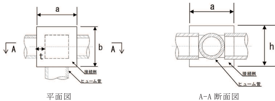
(1) 構造概要
