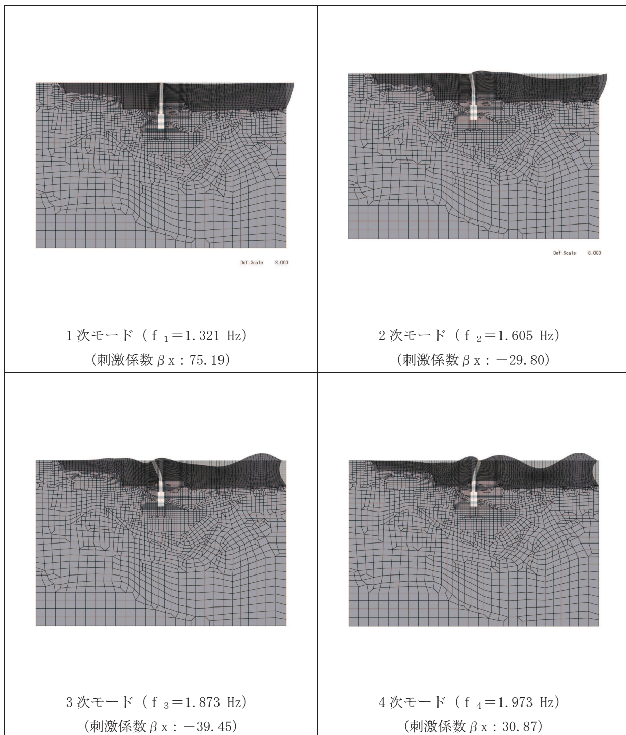
図 3-7(1) 固有値解析結果 (1/3) (No.1 揚水井戸)
