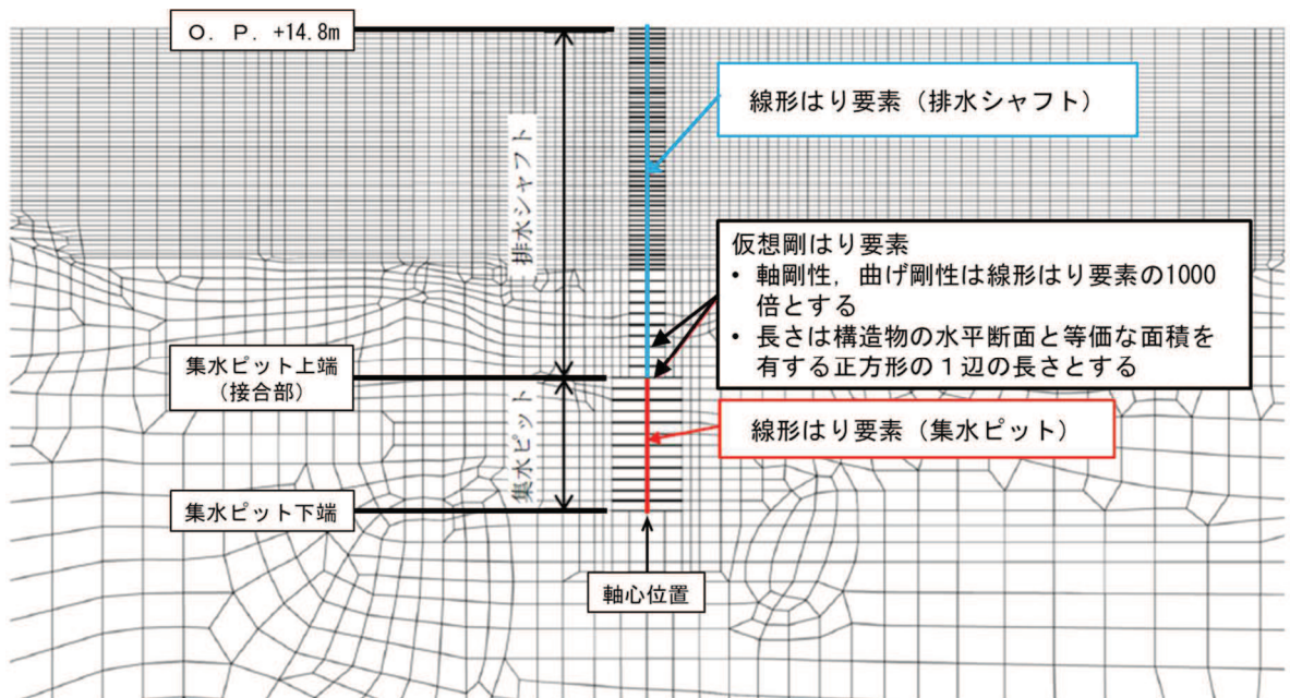
図 3-16 構造物の解析モデル
