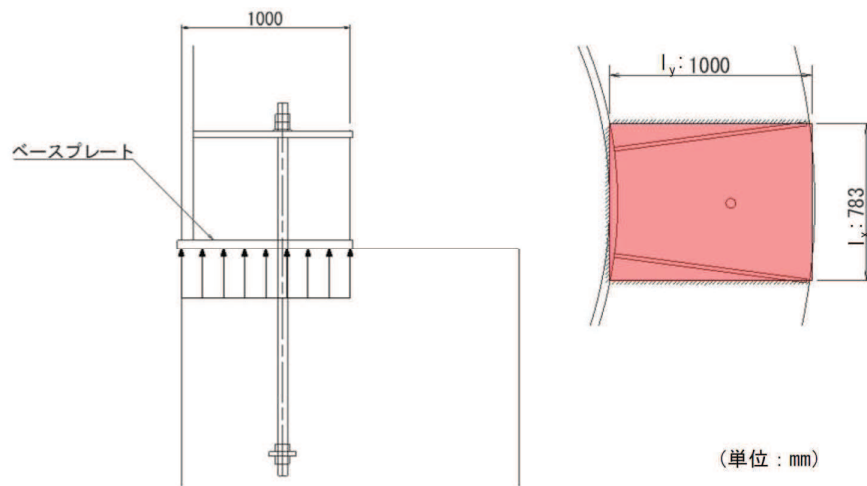
図 3-26 ベースプレート検討概念図
