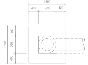
B-B 断面图
