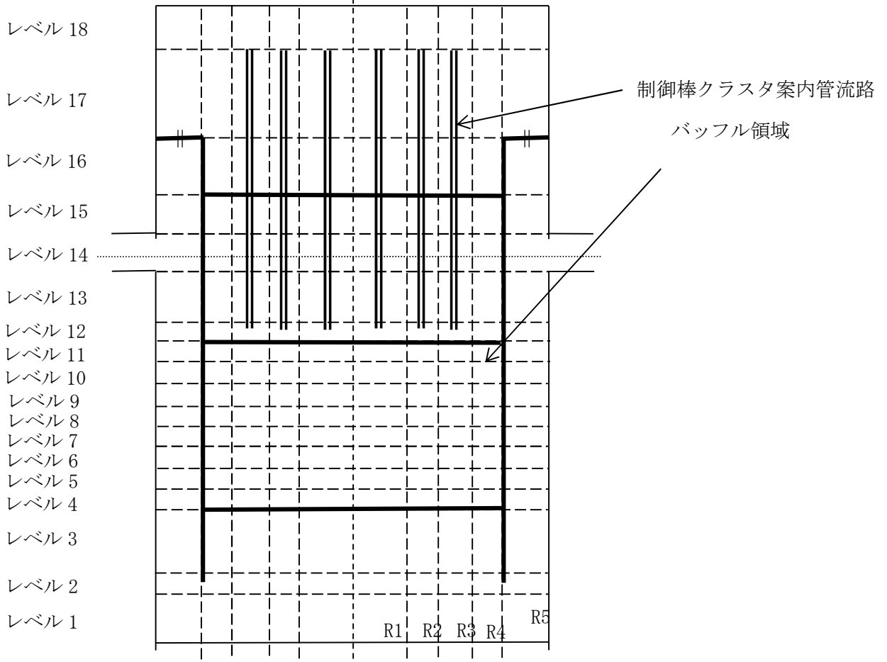
図5 PWR 3 ループプラントの原子炉容器内の炉心領域を除くセル分割
