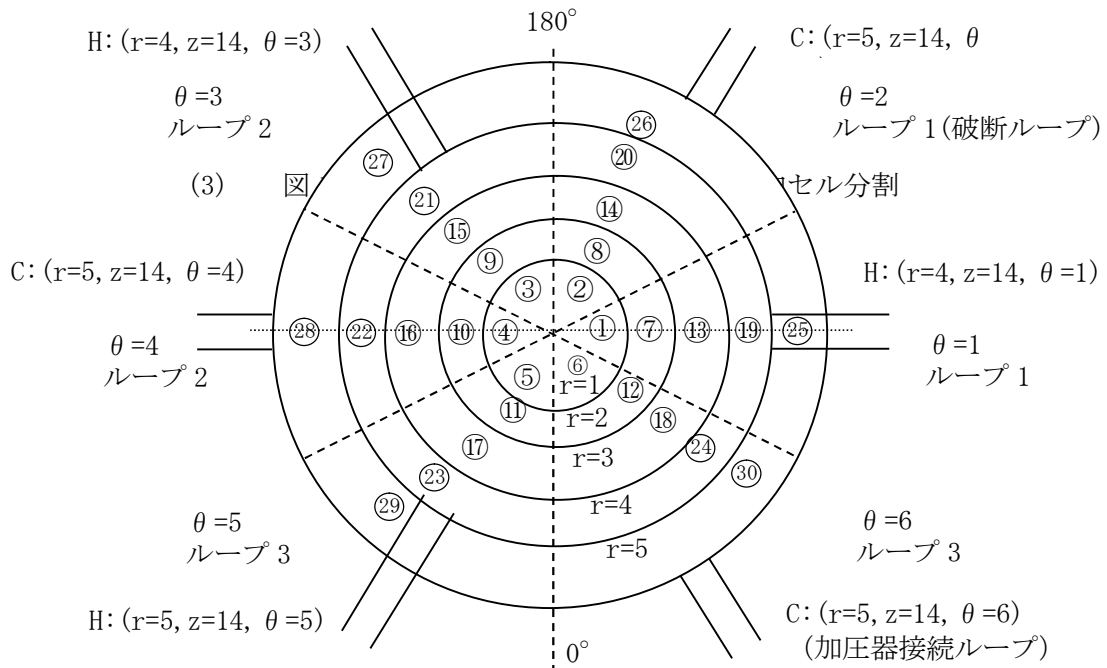
(j) 水平断面相対セル番号
