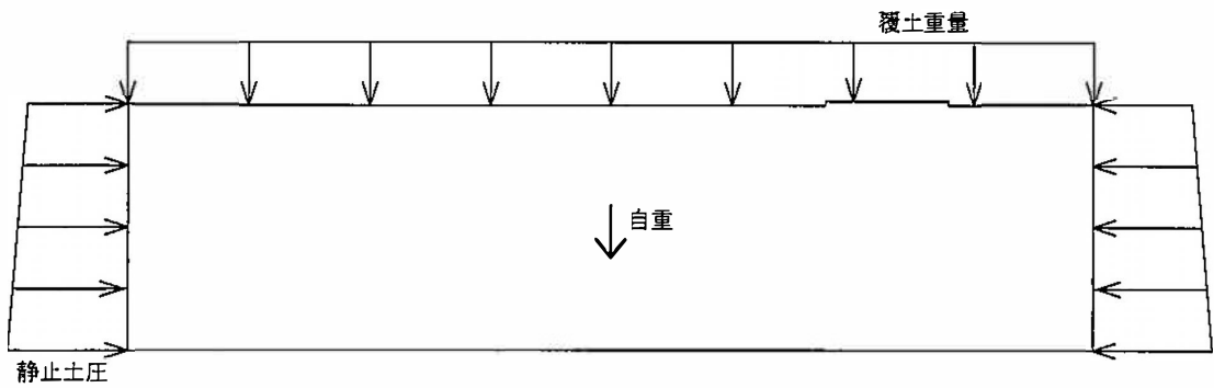
(a) 常時
