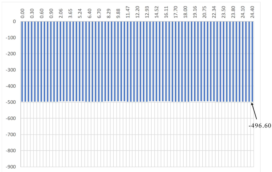
図 1-イ (ハ)-25 地盤反力(覆土後 常時、単位 : \text{kN/m}^2 )
