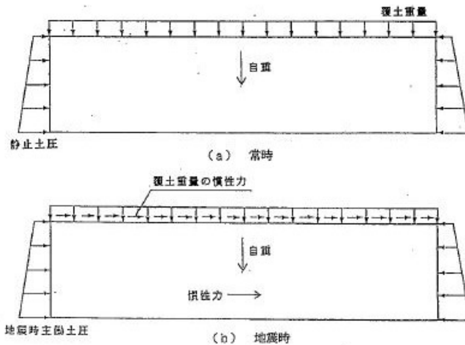
図 1-イ(ハ)-6 荷重の組合せ
