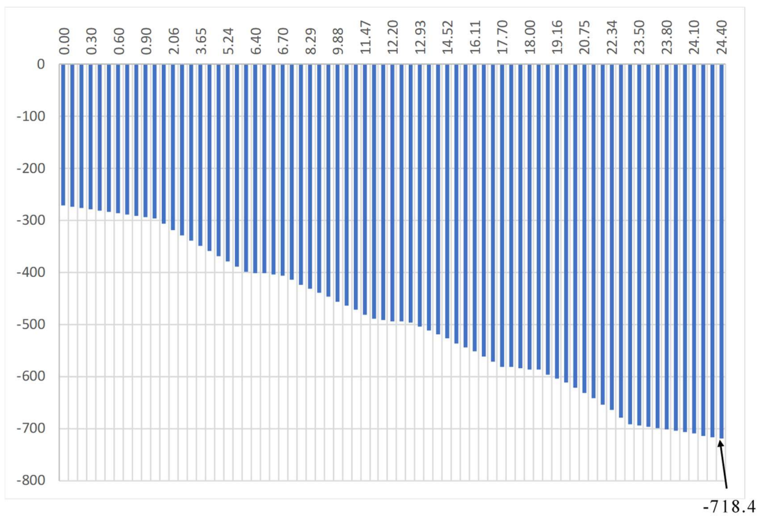
図 1-イ (ハ)-26 地盤反力(覆土後 地震時、単位 : \text{kN/m}^2 )
