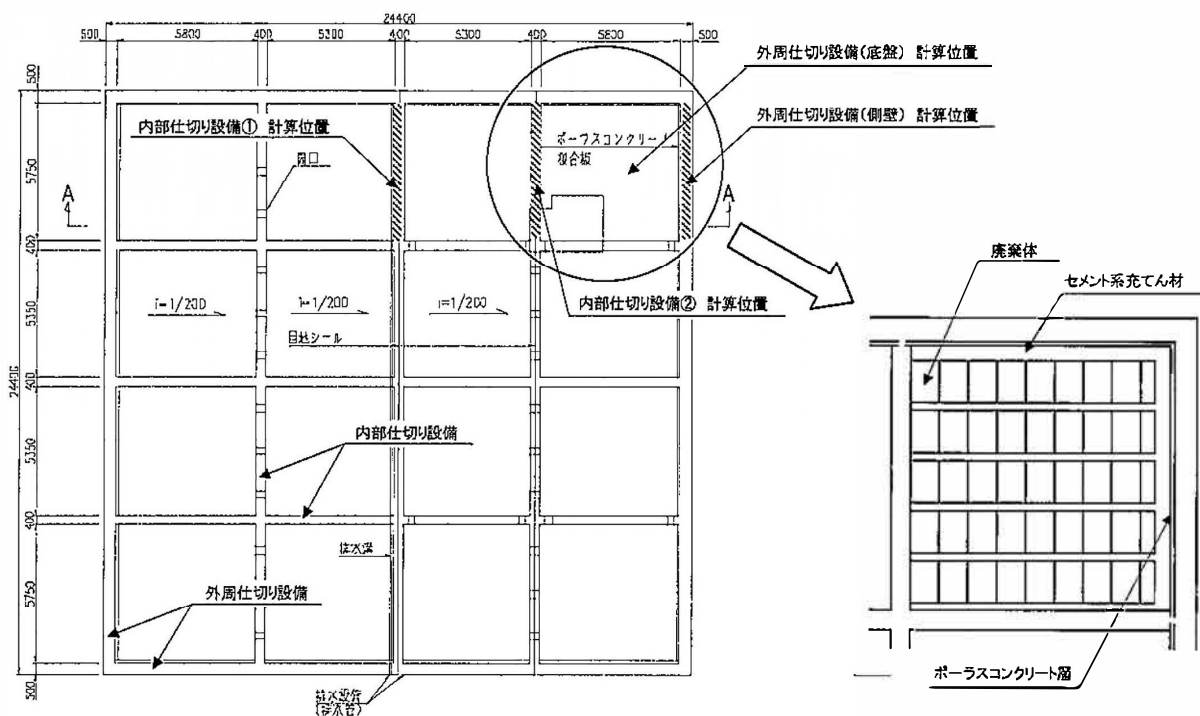
平面図
