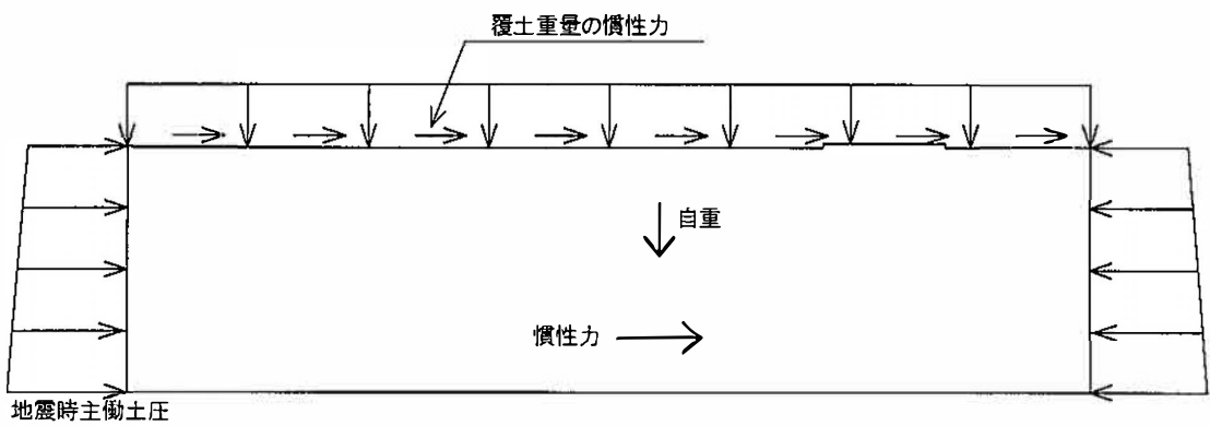
(b) 地震時
