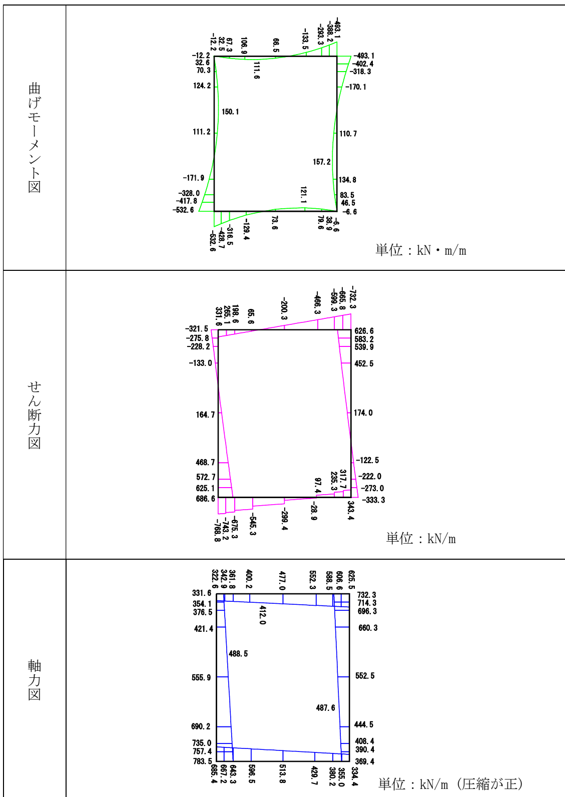
図 1-イ(ニ)-5 断面力図(地震時)
