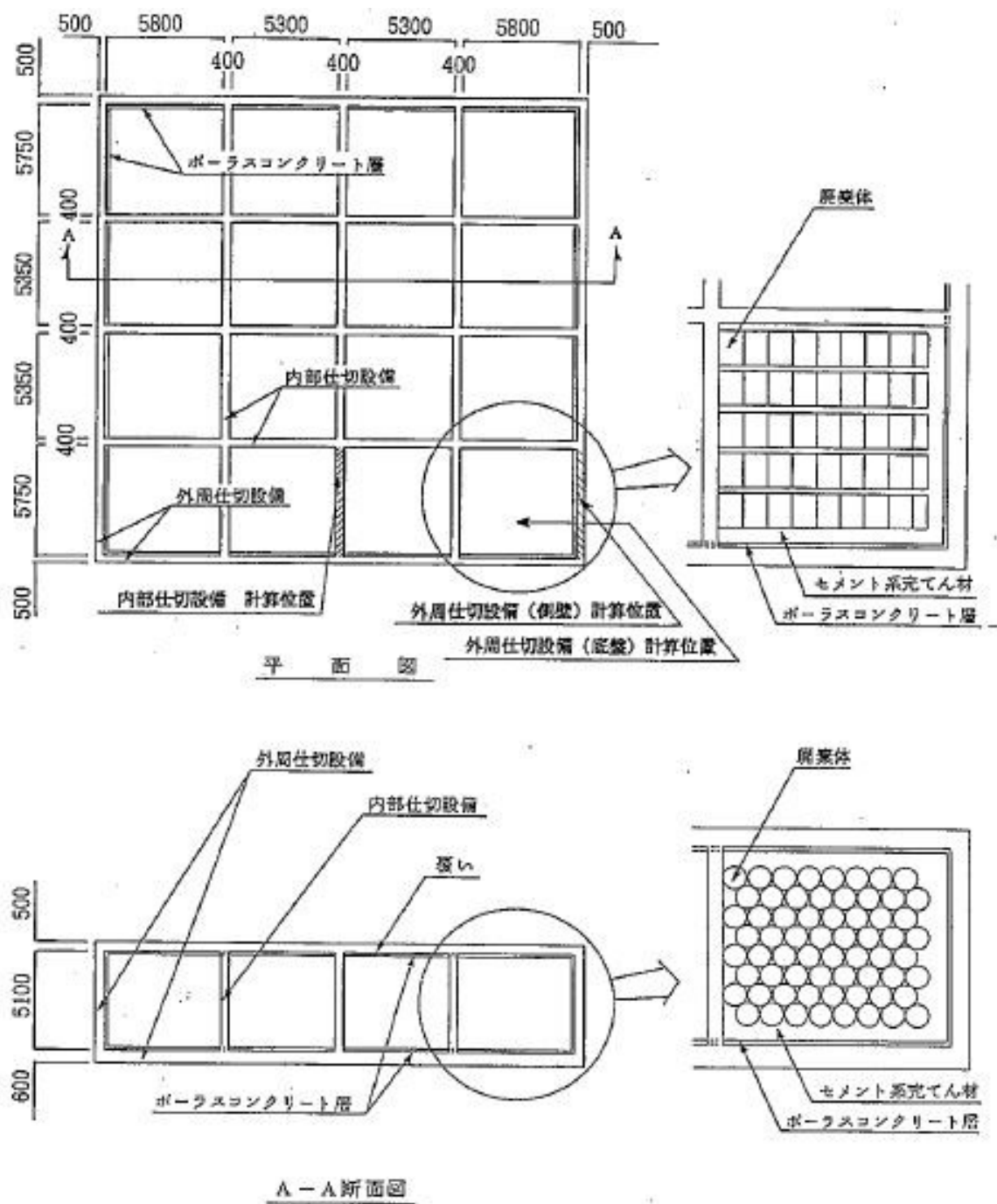
図 1-イ(ハ)-3 埋設設備の平面図、断面図 (1号廃棄物埋設地第6群C埋設設備及び7,8群埋設設備を除く)
