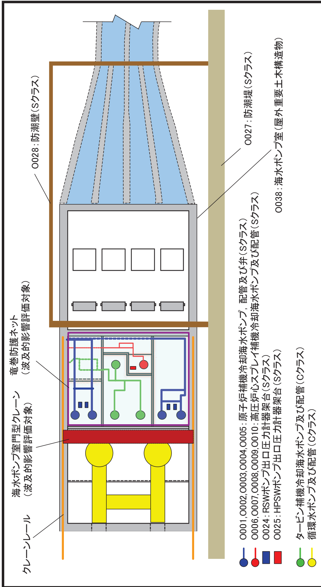
第 6.4-3 図 女川 2 号機 損傷, 転倒, 落下等に係る建屋外上位クラス施設配置図 (海水ポンプ室)
