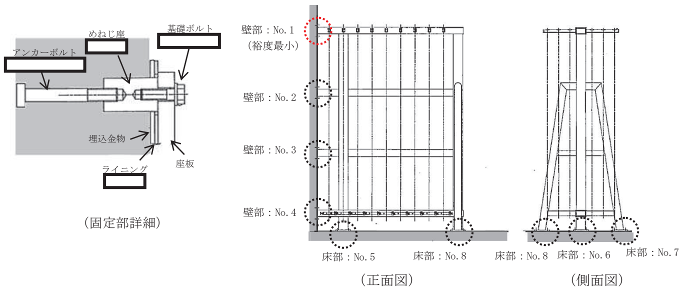
添付9-2図 制御棒貯蔵ハンガ（その2）構造図
