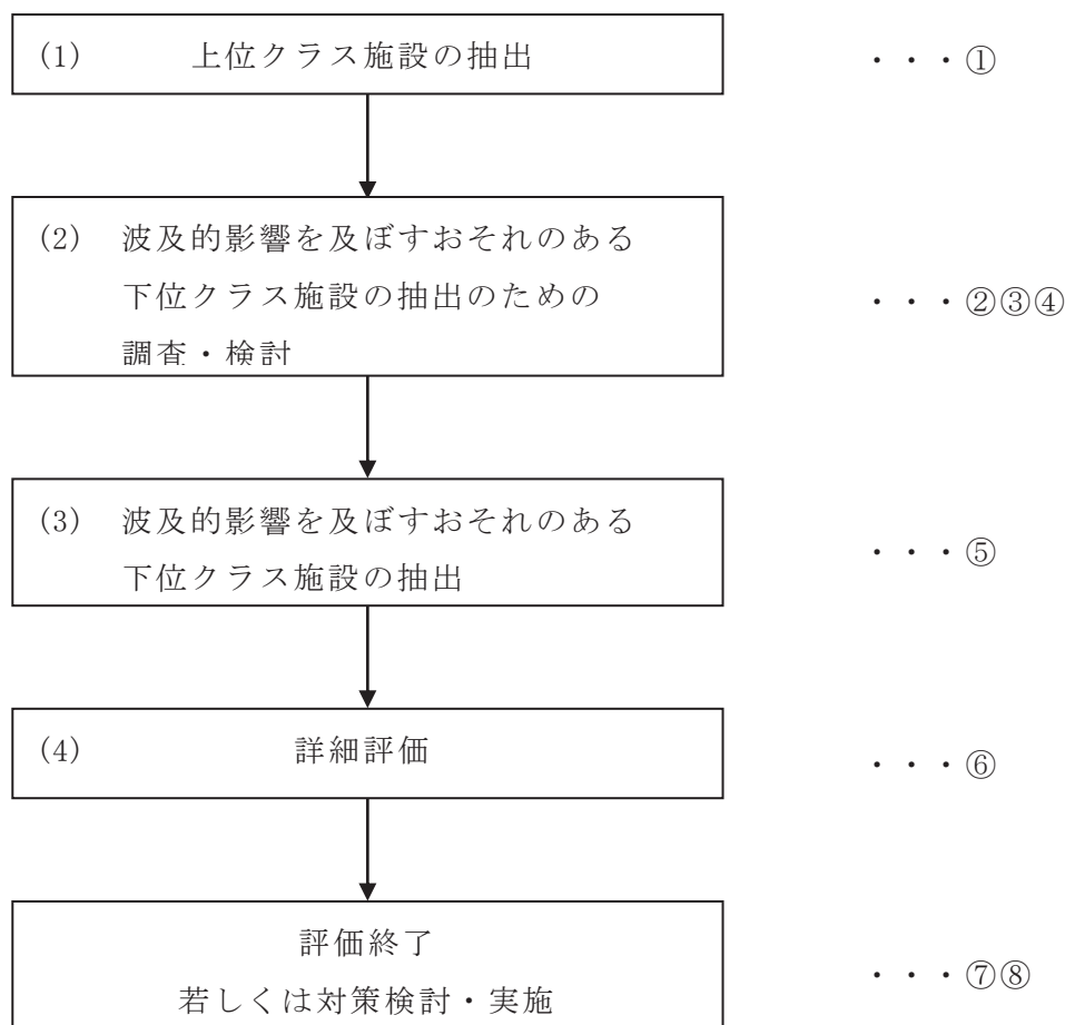
図1 波及的影響に係る概略検討フロー
