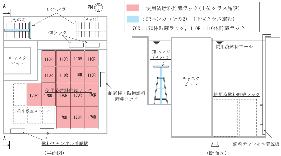
添付 9-1 図 使用済燃料プール内配置状況
