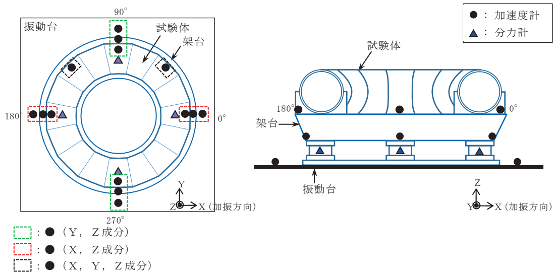
図6 計測機器設置位置
