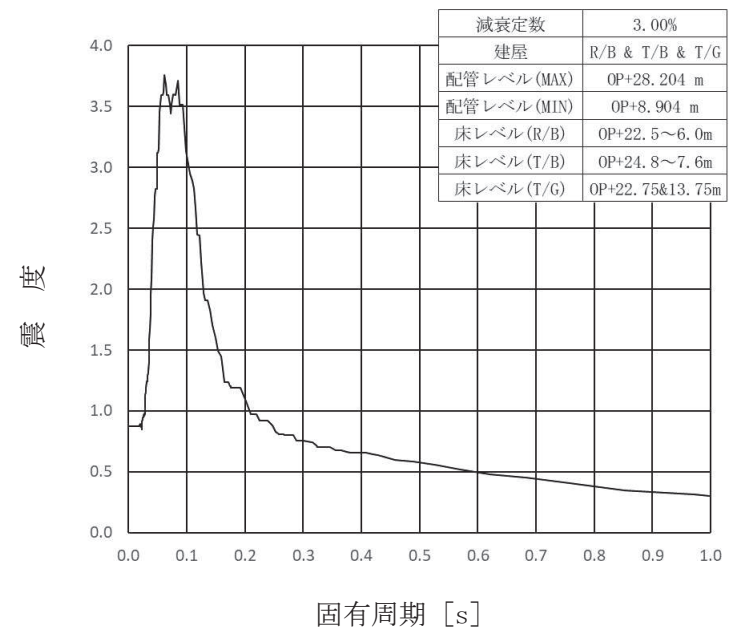
図 3-2 床応答スペクトル (鉛直方向)
