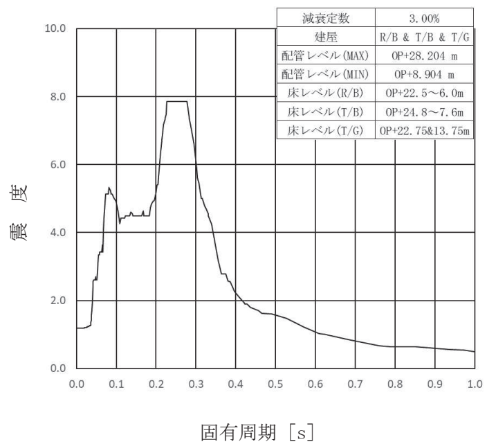
図 3-1 床応答スペクトル (水平方向)
