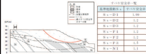
図 3.3.2-8 斜面 B のすべり安定性評価結果
