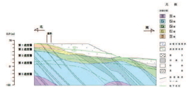
図 3.3.2-14 斜面Bの地質断面図
