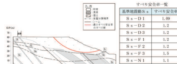
図 3.3.2-15 斜面Bのすべり安定性評価結果
