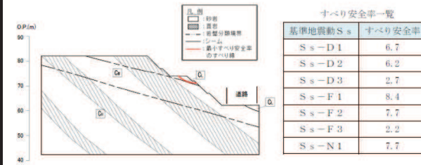
図 3.3.2-7 斜面 A のすべり安定性評価結果
