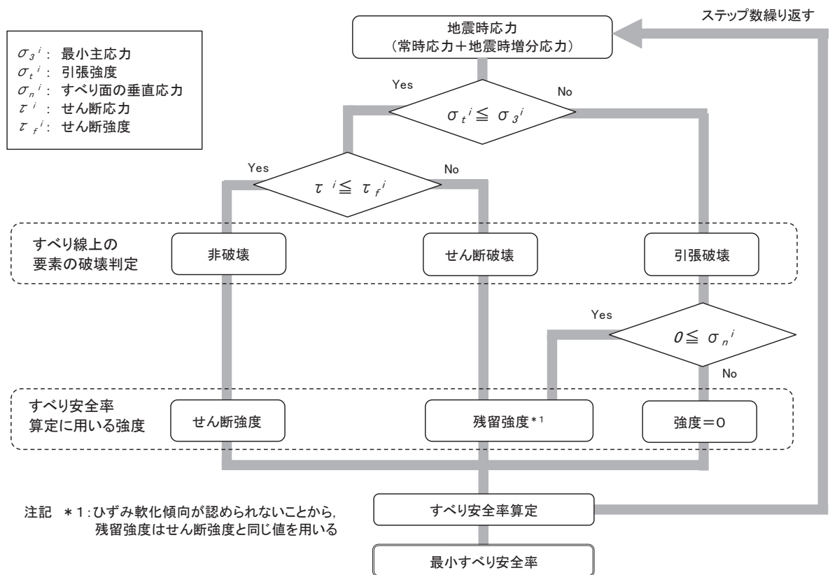
図 3.4-20 すべり安全率の算定フロー
