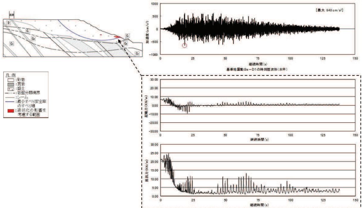
図3.4-26 液状化の影響を考慮する範囲における起動力及び抵抗力
