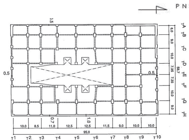
図 6.3.5-1 平面図 (1階)
