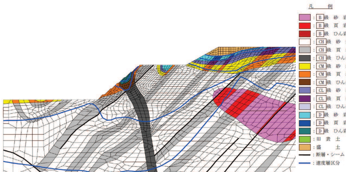
図 3.4-30 解析モデル図
