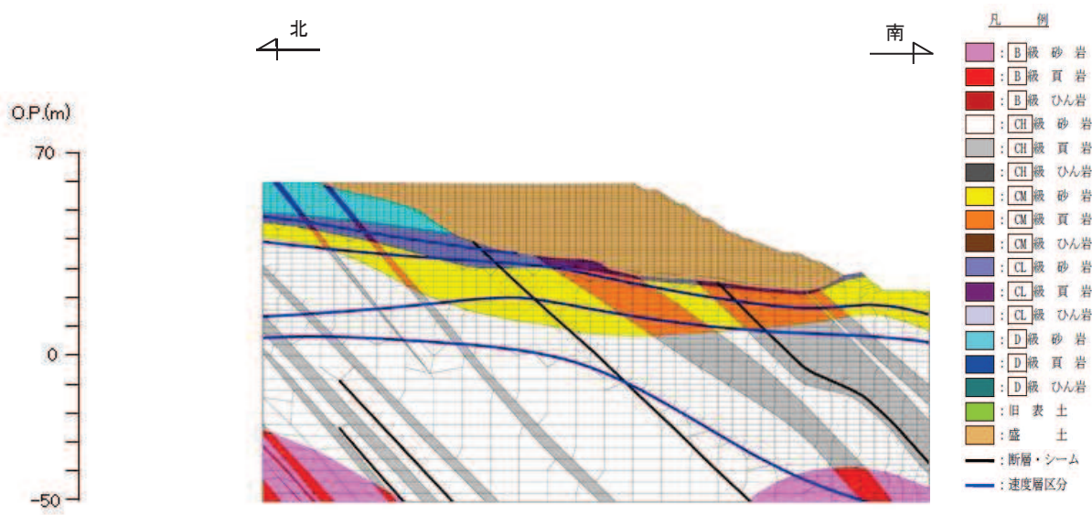
図 3.4-22 解析モデル図
