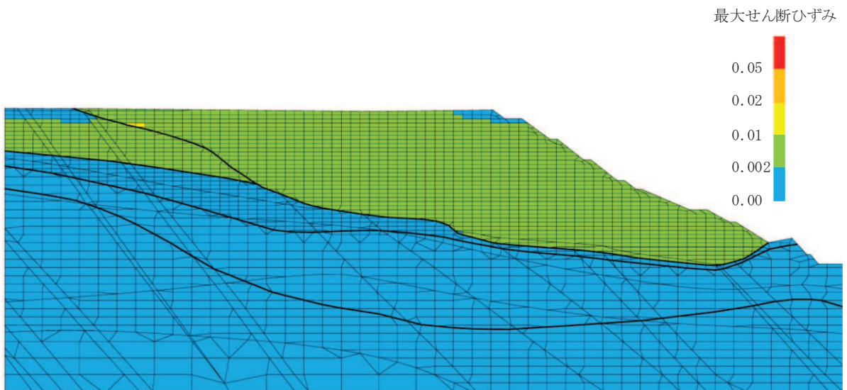
図 3.4-12 斜面 B における最大せん断ひずみ分布図 ( S_s - D1 )
