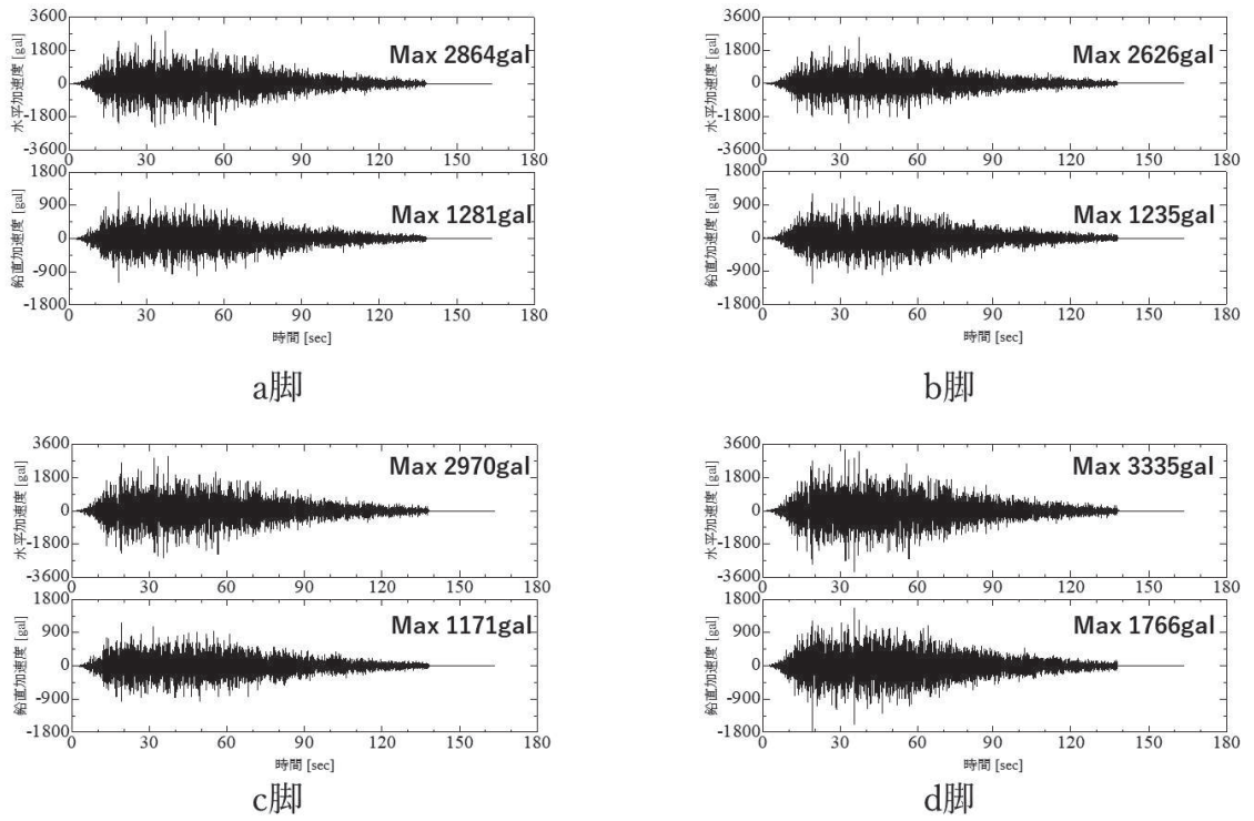
図 6. 2. 2-15 加速度時刻歴波形 (Ss-D1 位相反転ケース)
