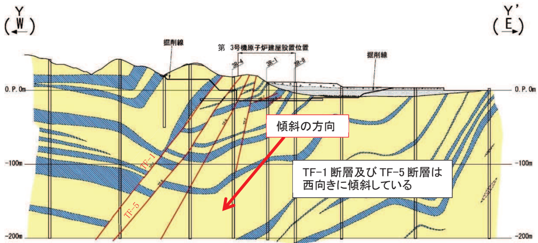
図 3.4-28 事務建屋の周辺斜面の評価断面選定根拠
