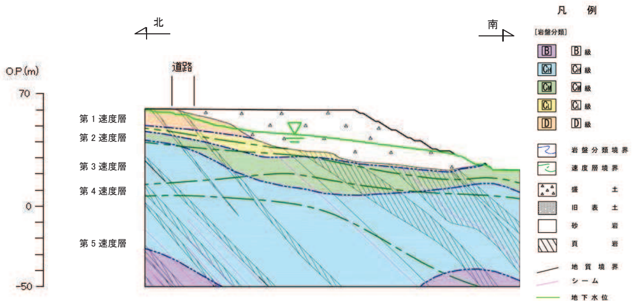
図 3.4-18 斜面 B の地質断面図
