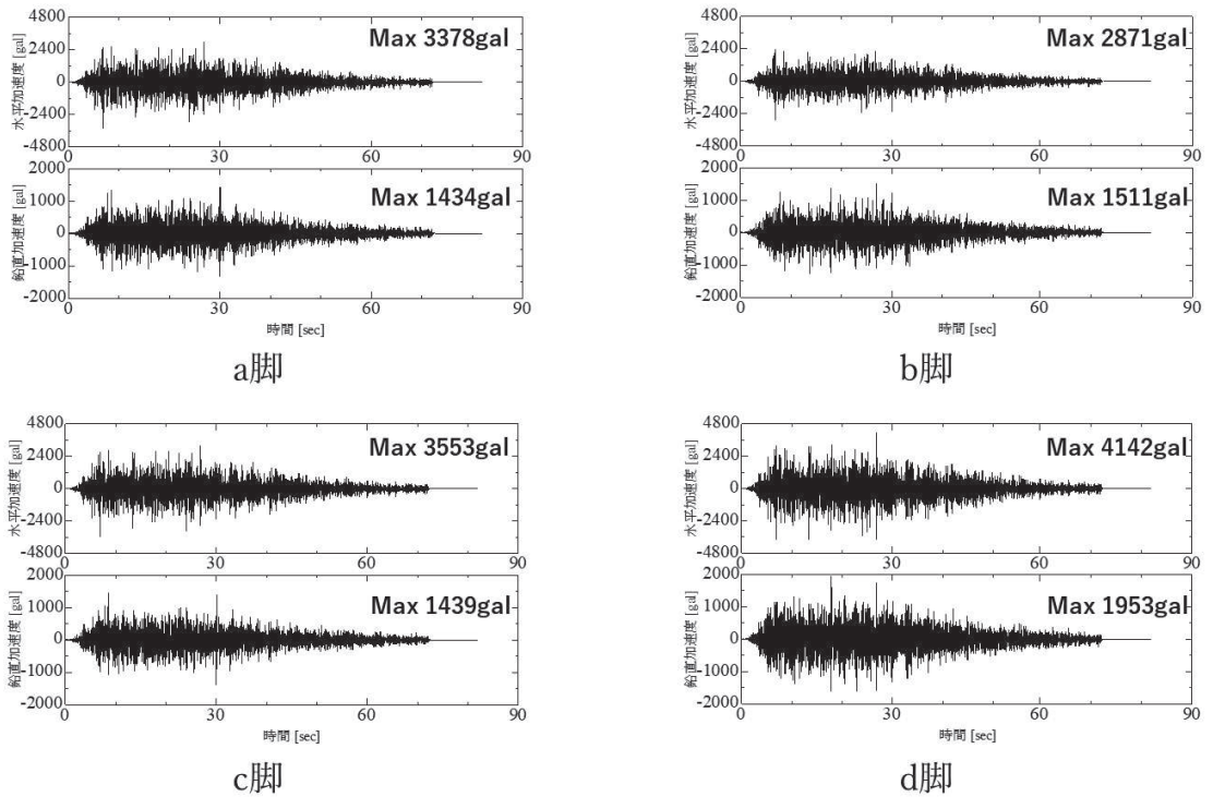
図 6. 2. 2-18 加速度時刻歴波形 (Ss-D2 位相反転ケース)
