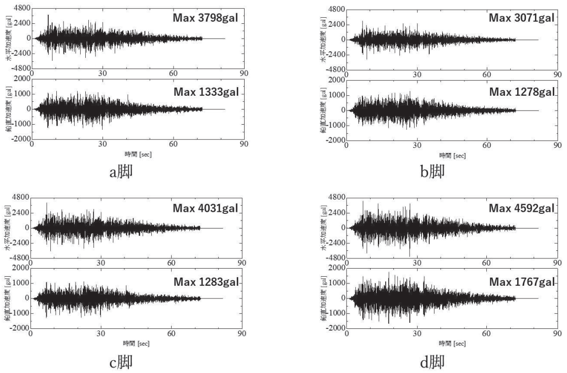
図 6. 2. 2-17 加速度時刻歴波形 (Ss-D2)
