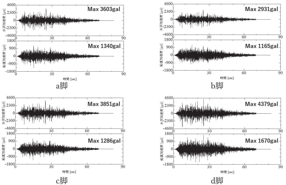
図 6. 2. 2-21 加速度時刻歴波形 (Ss-D3 位相反転ケース)
