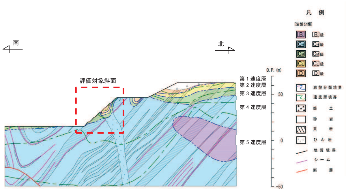
図 3.4-29 地質断面図
