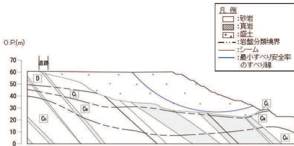
図 3.4-21 すべり安全率が最小となったすべり面
