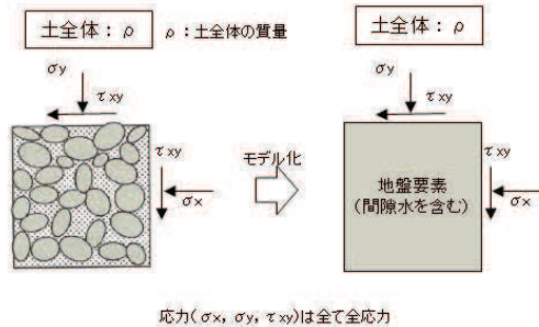
図 3.4-15 全応力解析及び有効応力解析の概念図
