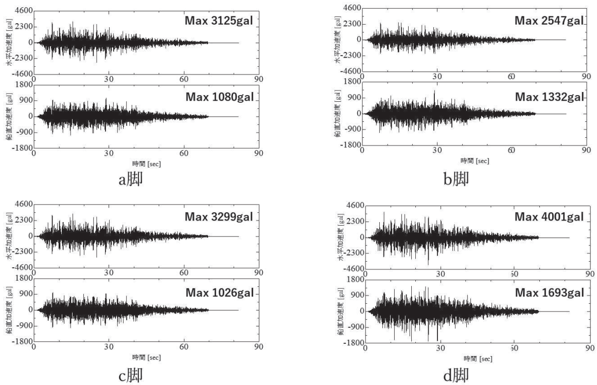
図 6. 2. 2-20 加速度時刻歴波形 (Ss-D3)
