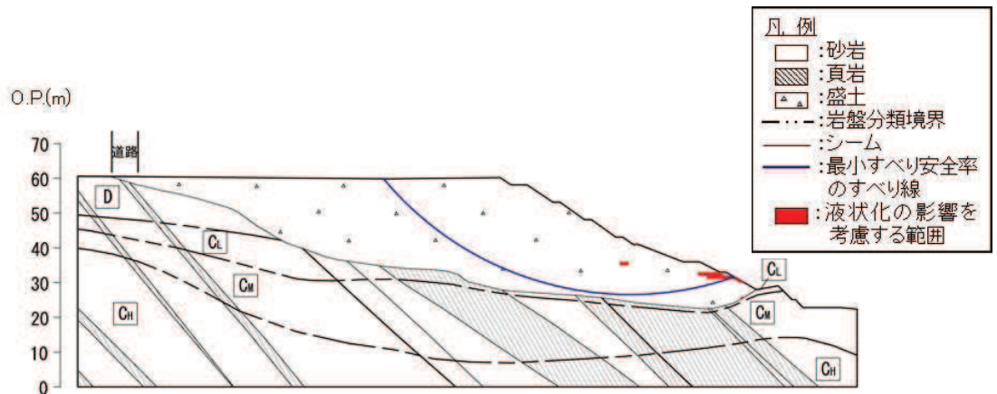
図 3.4-25 すべり線
