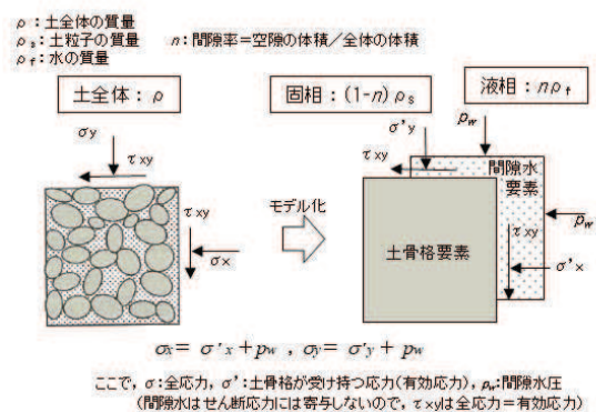
図 3.4-15 全応力解析及び有効応力解析の概念図
