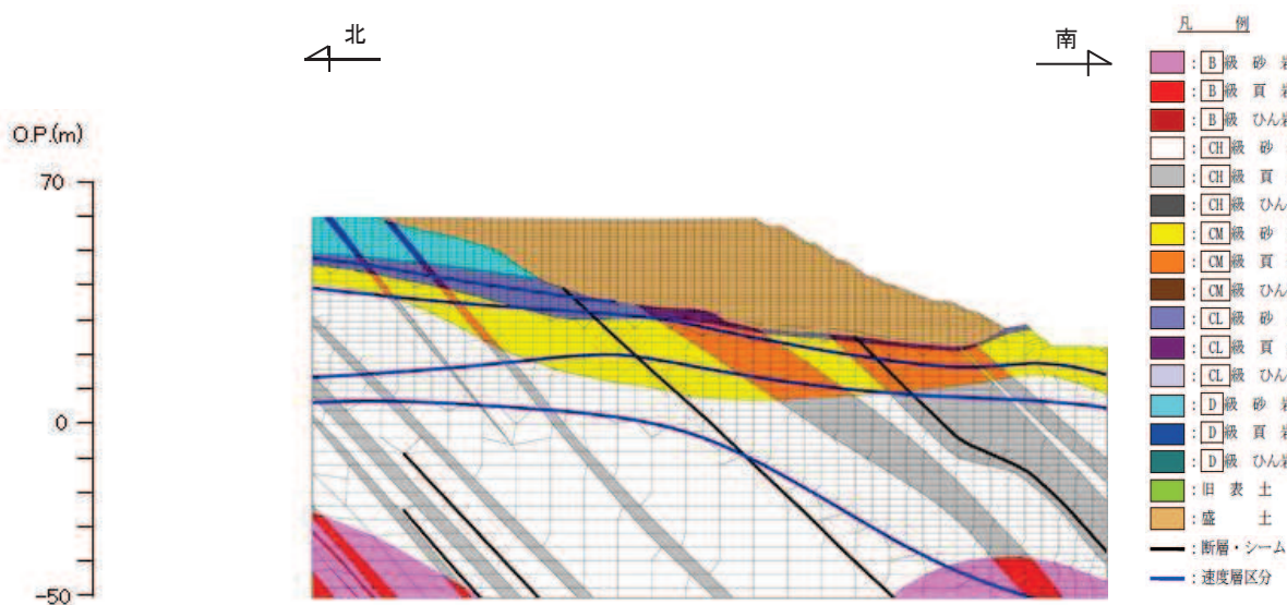
図 3.4-19 解析モデル図
