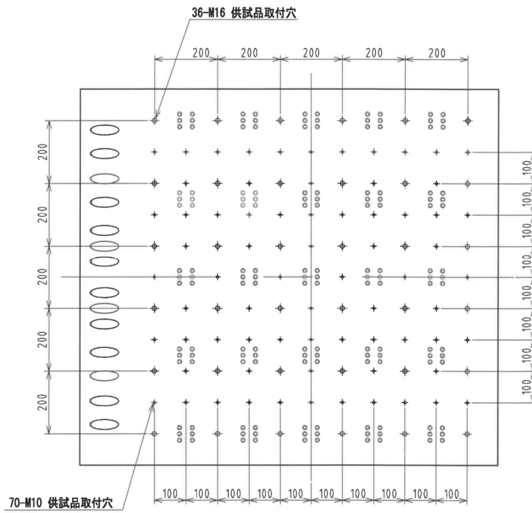
図 5 水平補助テーブル ネジパターン
