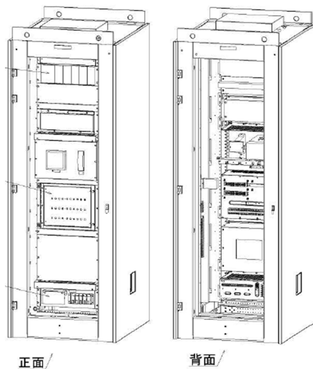
図 3 制御盤の概要
