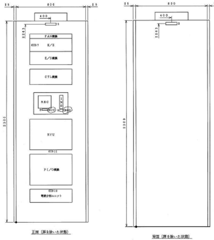
図 2 制御盤内部の機器配置概要
