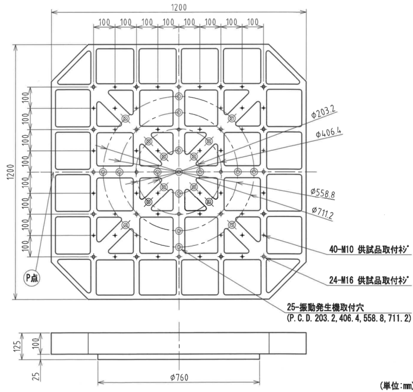
図 4 垂直補助テーブル ネジパターン
