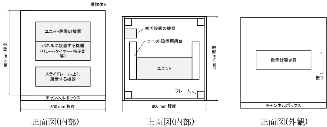
図 1 供試体 A の概要
