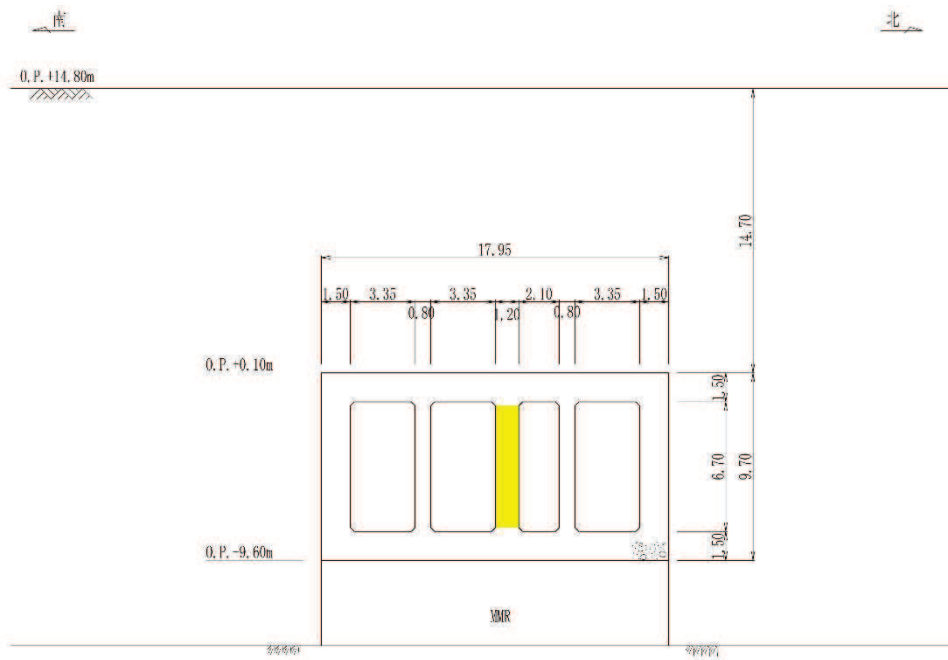
図 2-6(2) Ccb 工法を適用する部材
