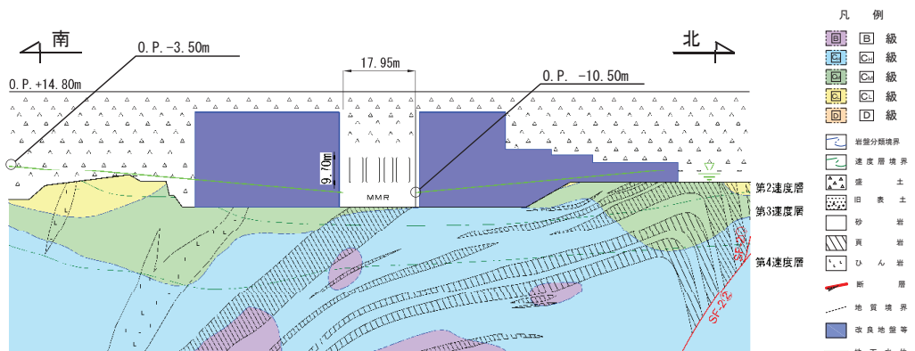
図 2-30 原子炉機器冷却海水配管ダクト(鉛直部) 地震時荷重算出地質断面図(C-C 断面:南北)
