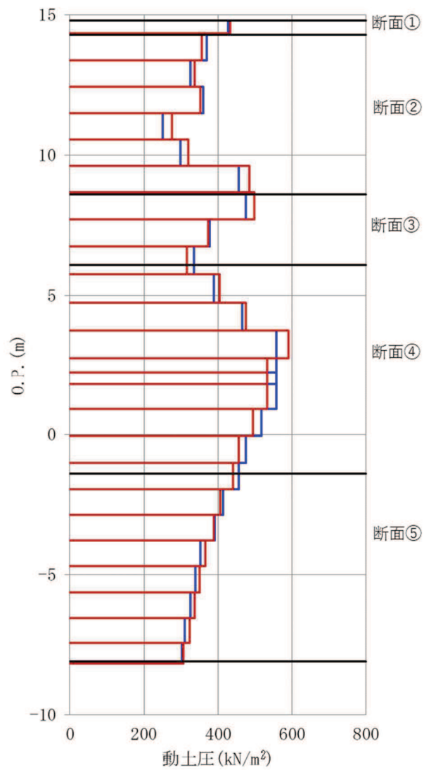
図 3.3-1 設計用モデルの土圧と剛性低下モデルの土圧の比較
