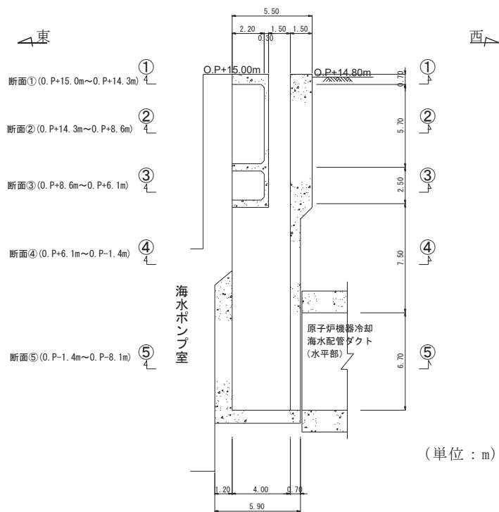
図 3-3 原子炉機器冷却海水配管ダクト（鉛直部）縦断図（B-B 断面）
