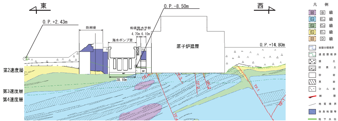
図 2-24 地盤改良範囲 (鉛直部横断図, ④ - ④断面)
