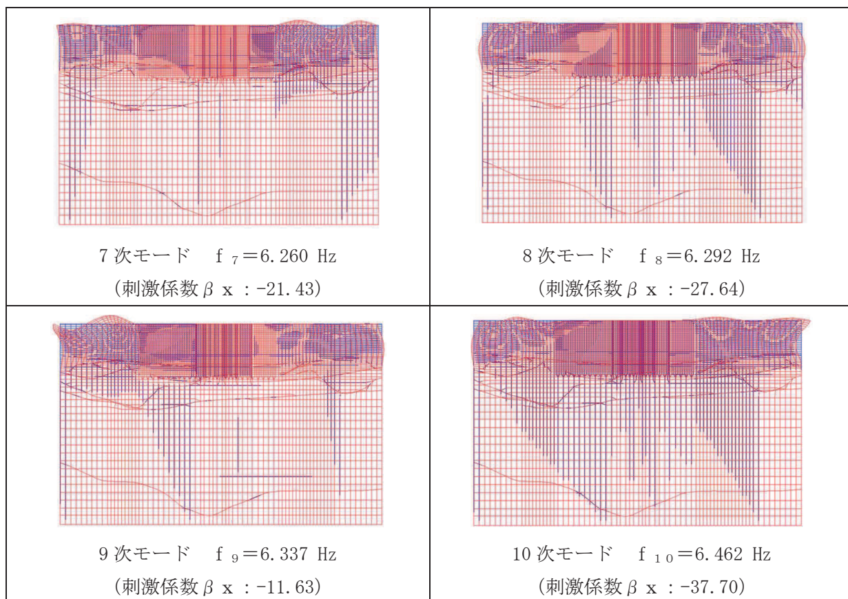
図 3-16(2) 固有値解析結果 (モード図) (A-A 断面 : 南北) (2/2)
