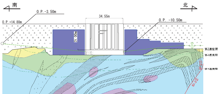
図 2-28 原子炉機器冷却海水配管ダクト(鉛直部) 地震時荷重算出地質断面図(A-A 断面:南北)
