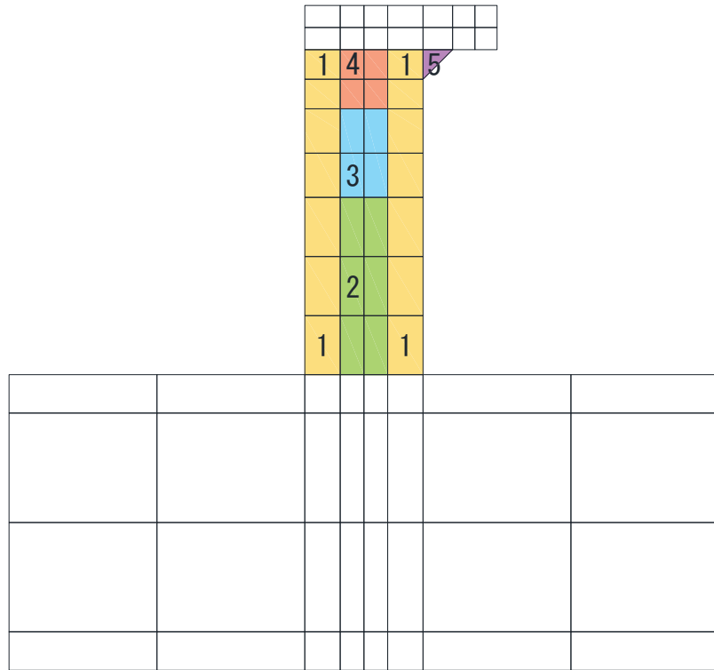
図 6-30(1) 要素プロパティ番号図 (隔壁)
