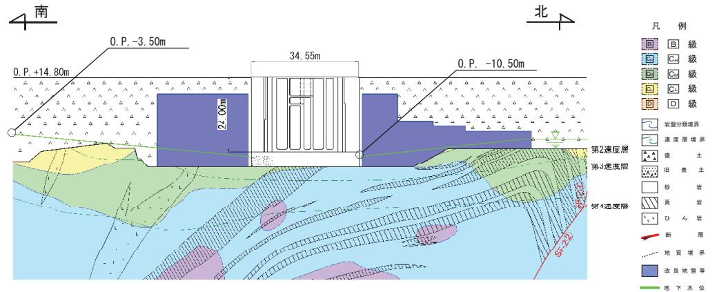
図 2-35 設計用地下水位 (A-A 断面)
