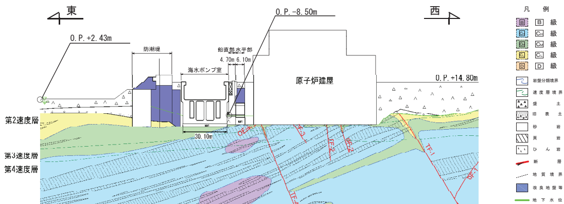
図 2-29 原子炉機器冷却海水配管ダクト(鉛直部) 地震時荷重算出地質断面図(B-B 断面:東西)
