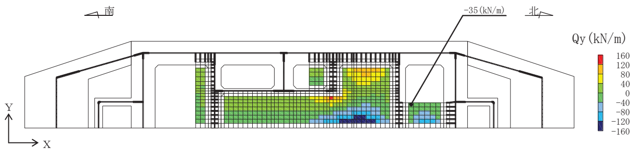
図 7-7 せん断破壊に対する照査における照査値最大時の断面力分布図 (せん断力 (kN/m) : Q_y ) (頂版, 解析ケース③, S d - D 2 (++) )
