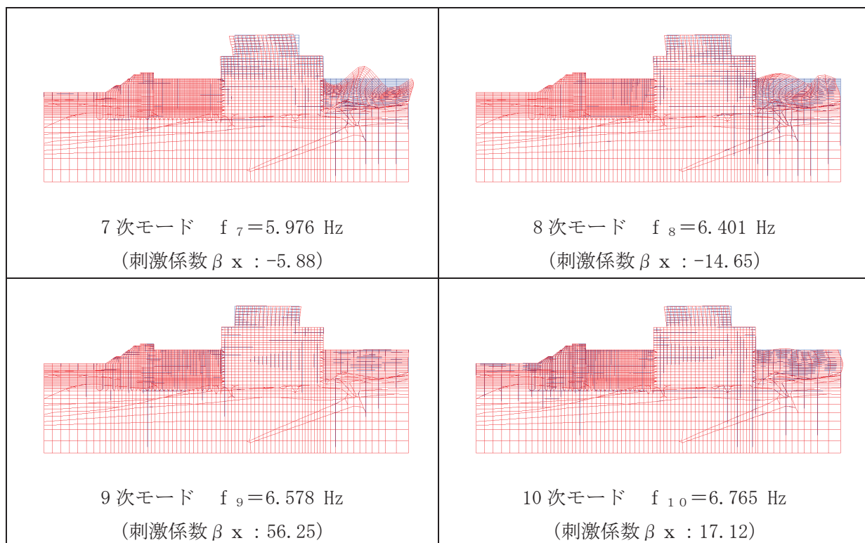
図 3-17(2) 固有値解析結果 (モード図) (B-B 断面 : 東西) (2/2)
