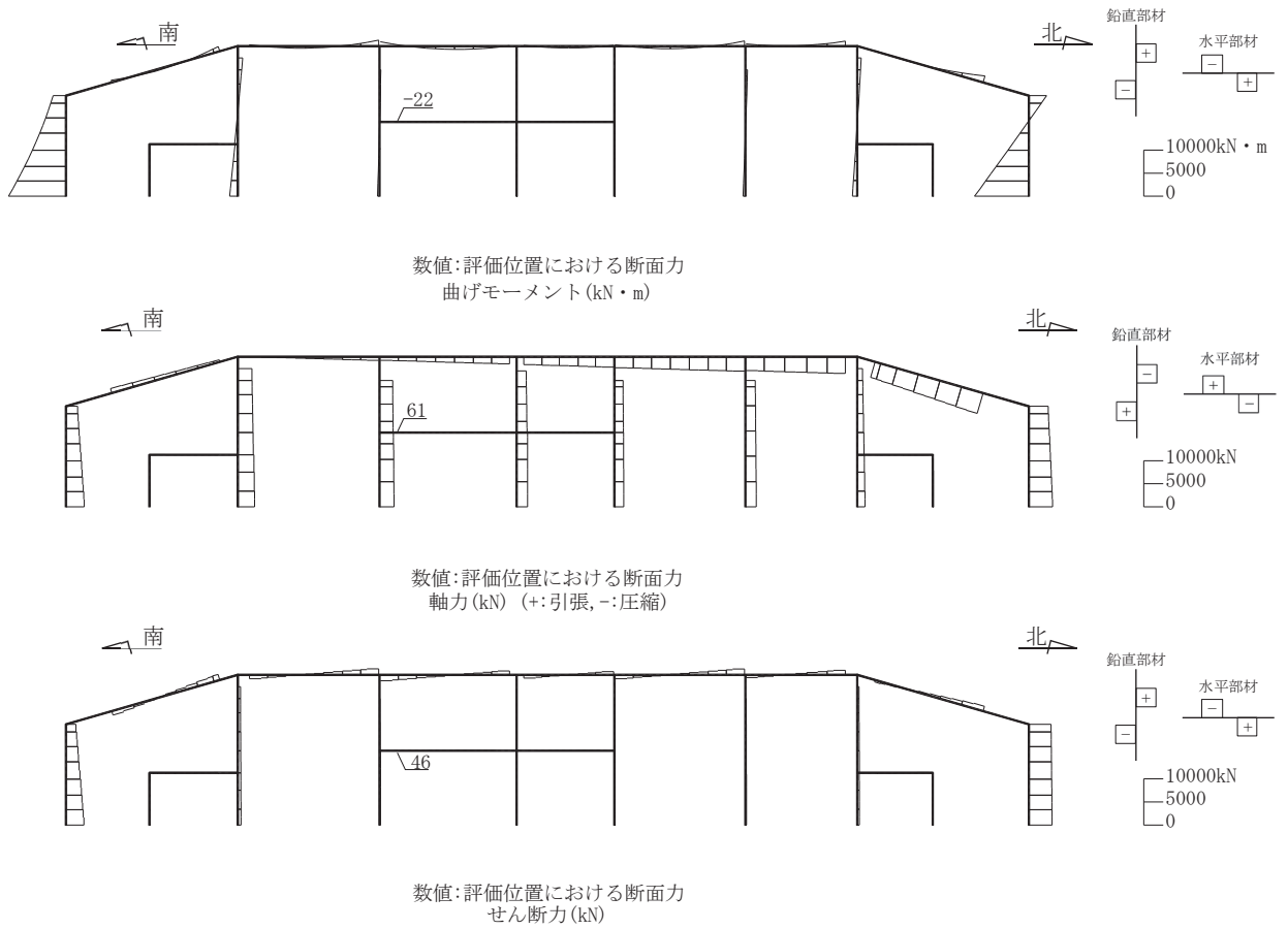
図 6-9 曲げ・軸力系の破壊に対する照査値最大時の断面力図 (断面②, 隔壁 (南北), 解析ケース①, S s - D 1 (-+))
