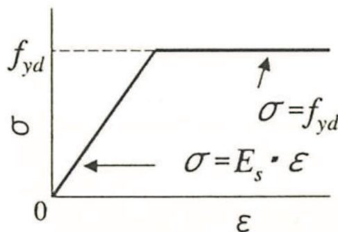
図 4-10 鉄筋の応力-ひずみ関係 (コンクリート標準示方書より引用)
