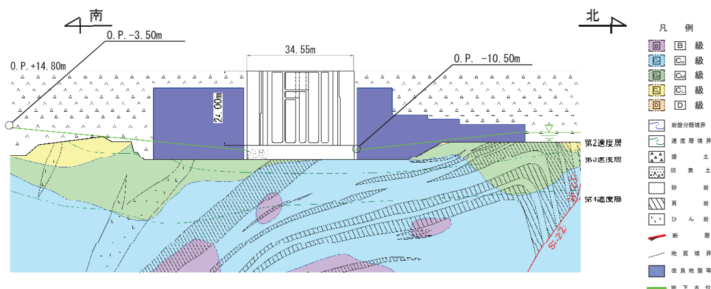
図 2-23 地盤改良範囲 (鉛直部縦断面図, ③ - ③断面)
