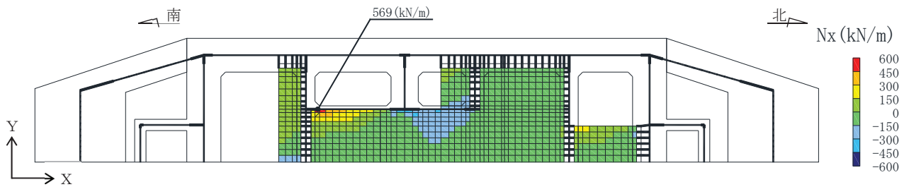
図 6-5 曲げ・軸力系の破壊に対する照査値最大時の断面力分布図 (軸力 (kN/m) : N_x ) (頂版, 解析ケース④, S s - D 2 (++) )
