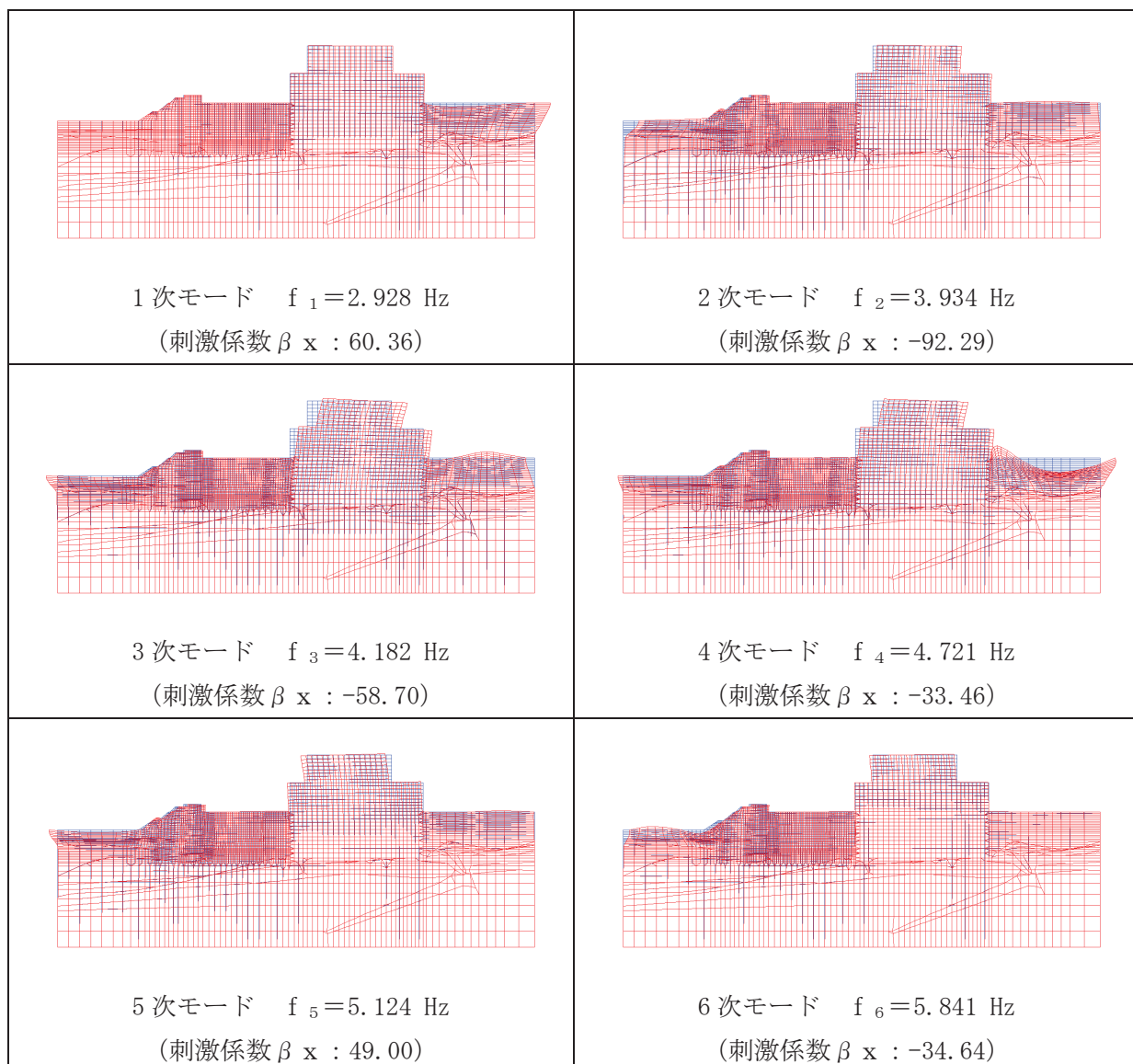
図 3-17(1) 固有値解析結果 (モード図) (B-B 断面 : 東西) (1/2)
