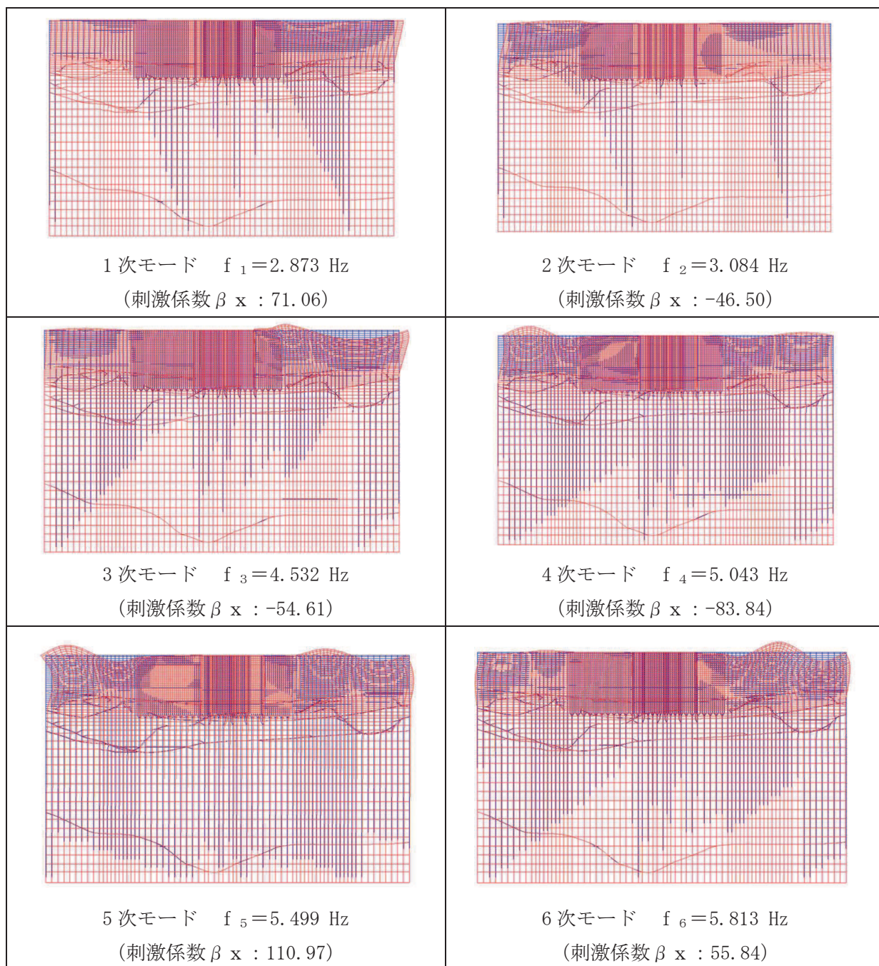
図 3-16(1) 固有値解析結果 (モード図) (A-A 断面 : 南北) (1/2)
