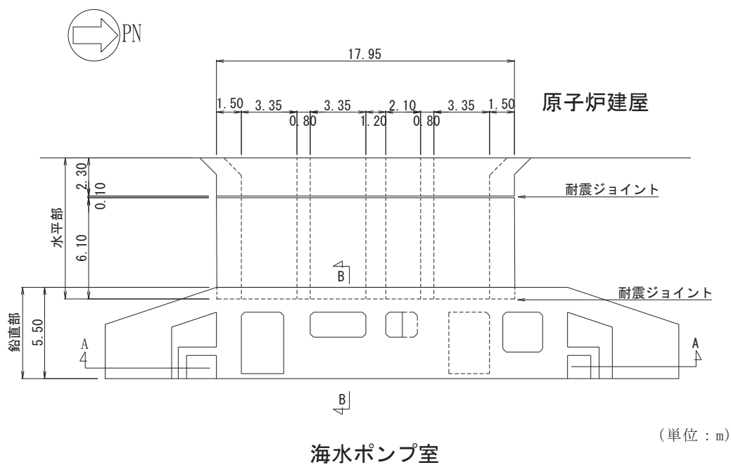
図 3-1 原子炉機器冷却海水配管ダクト（鉛直部）平面図
