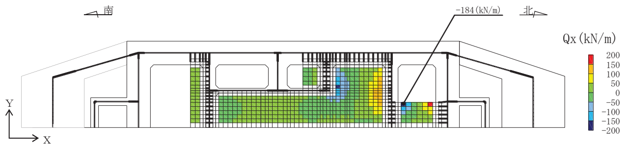
図 7-6 せん断破壊に対する照査における照査値最大時の断面力分布図 (せん断力 (kN/m) : Q_x ) (頂版, 解析ケース③, S d - D 2 (++) )
