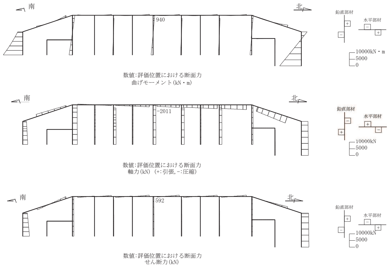
図 6-21 せん断破壊に対する照査値最大時の断面力図
