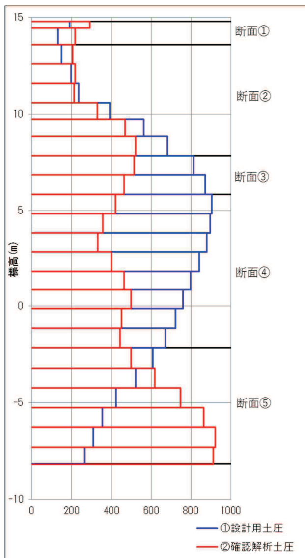
図 2.3-3 等価剛性モデルと単独モデルの地震時土圧の比較 (S s - D 1 (++) )
