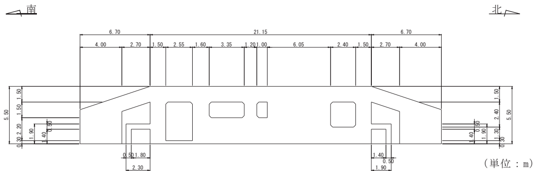
図 3-4 評価対象部材（頂版：断面①）
