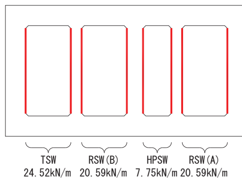
図3-18 機器・配管系の荷重図
