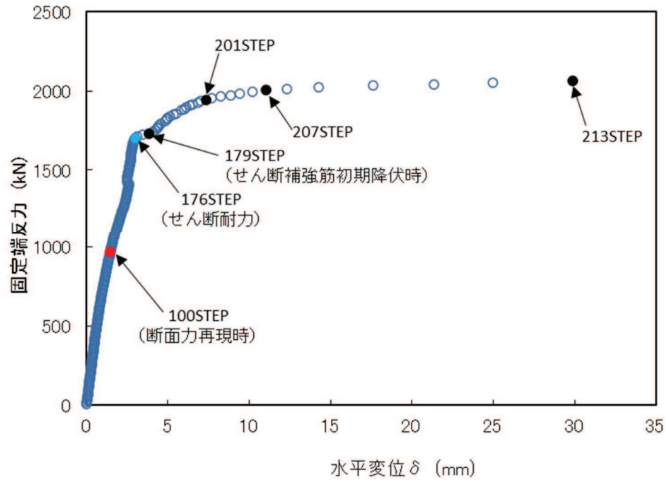
図 6-36 荷重-変位曲線
