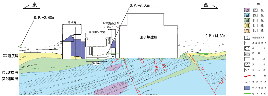
(a) 地震時荷重算出用地質断面図
