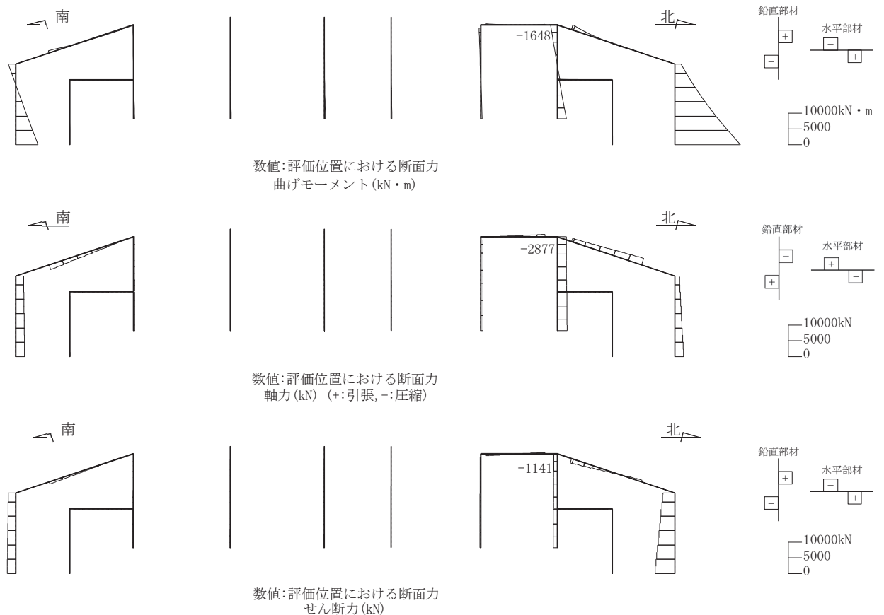
図 6-22 せん断破壊に対する照査値最大時の断面力図
