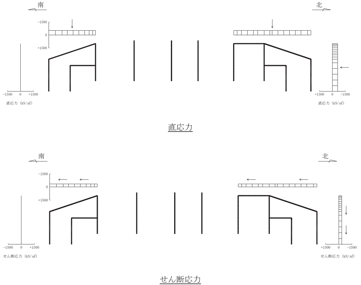
図6-1 (1) 作用荷重分布図 (直応力及びせん断応力) (断面⑤, 解析ケース③, S s -N1 (-+))
