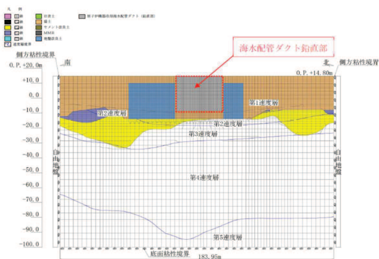
図 2.2-1 地震時土圧検証用の海水配管ダクト（鉛直部）単独モデル
