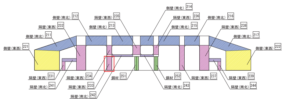
図 6-9 曲げ・軸力系の破壊に対する照査値最大時の断面力図 (断面②, 隔壁 (南北), 解析ケース①, S s - D 1 (-+))
