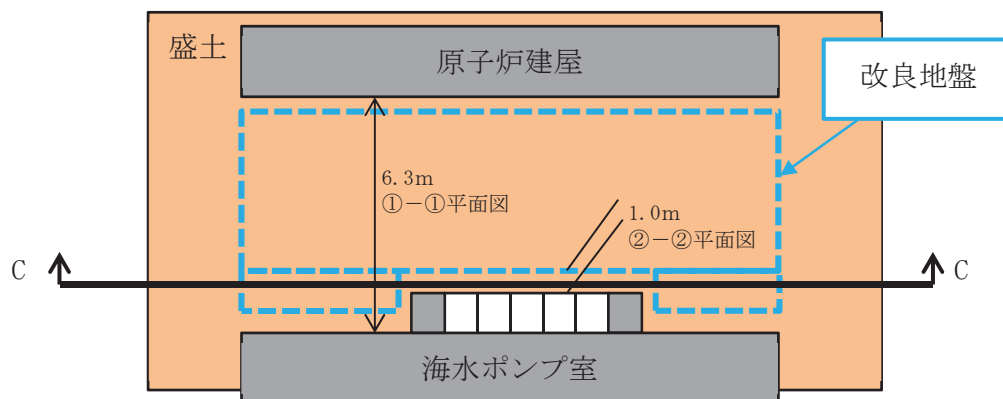
図 3-32 海水ポンプ室～原子炉建屋間の模式平面図
