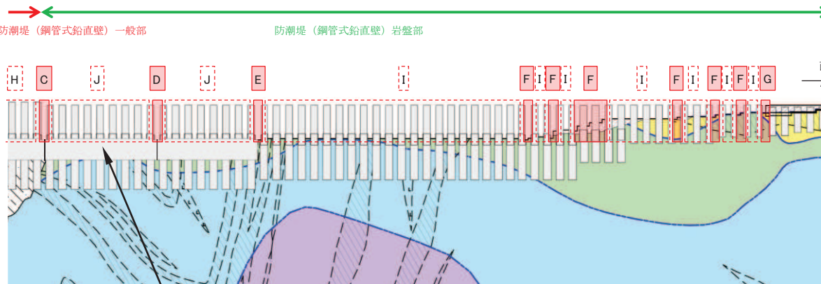
背面補強工 (縦線は構造目地)
