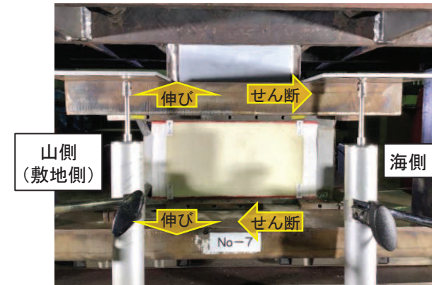
変形試験概要
