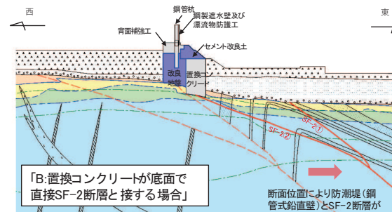
(断面B)
