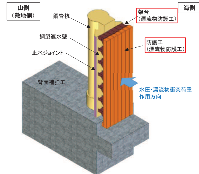
漂流物防護工の構造概要図
