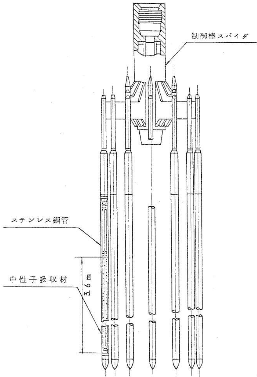
第1.4-23図 制御棒クラスター構造説明図
