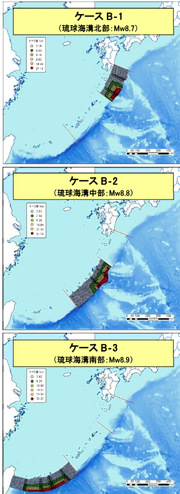
第1.2-7図(2) 琉球海溝の津波波源
