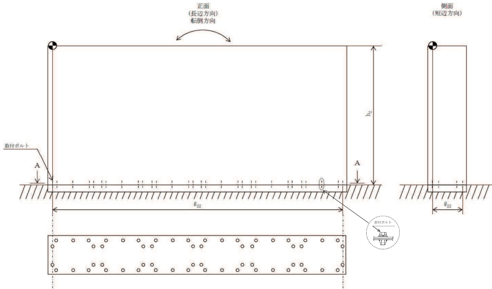
A~A 矢視図
