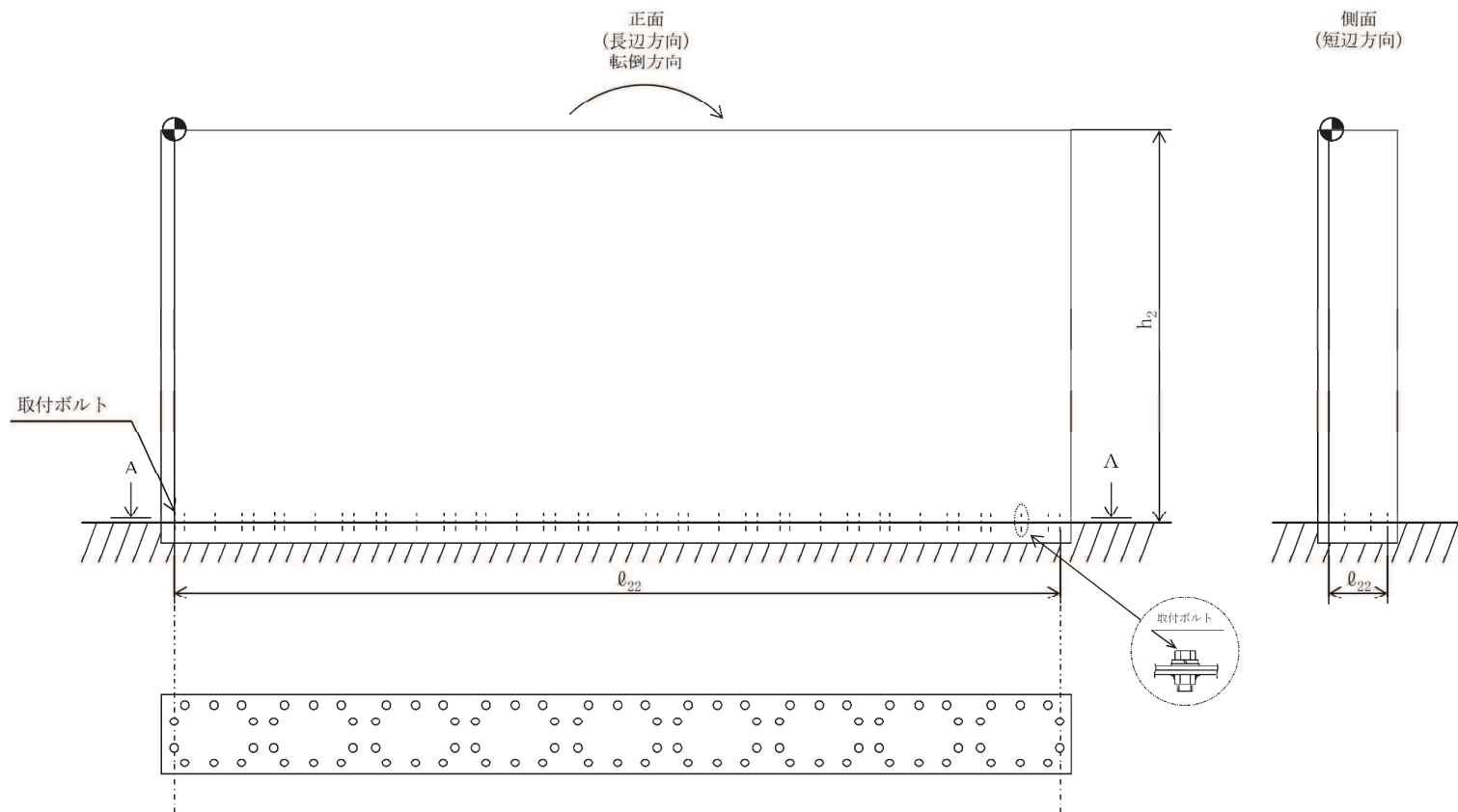
A~A矢视图
