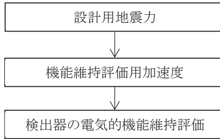
図 2-1 フィルタ装置水温度の耐震評価フロー
