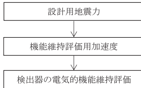
図 2-1 圧力抑制室内空気温度の耐震評価フロー
