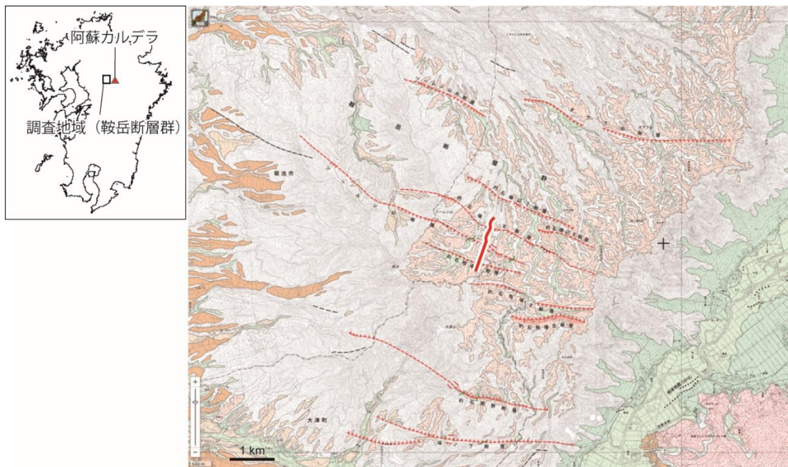
図1 調査地域（鞍岳断層群及びその周辺）及び調査測線（赤線）を示す位置図。 原図は地理院地図に都市圏活断層図を重ねたものを使用。
