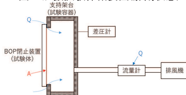
図6 気密性能試験概要図
