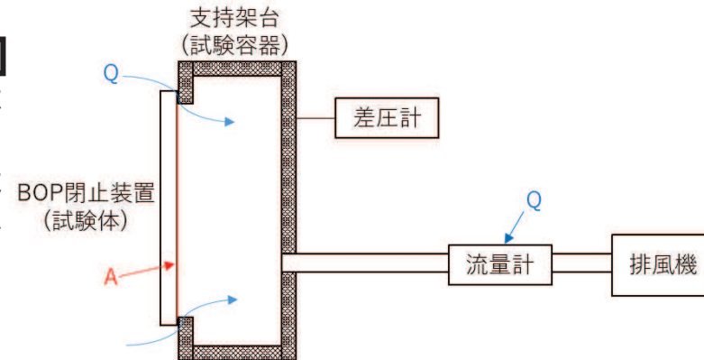
参考図2-18 気密性能試験概要図
