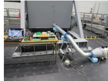
参考図2-19 BOP閉止装置気密性能試験状況
