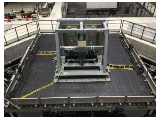
図7 BOP閉止装置加振試験状況
