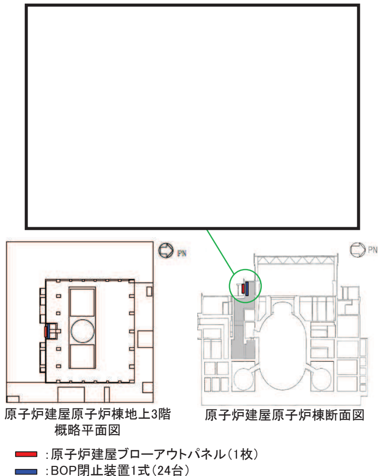
図1 BOP閉止装置配置図
