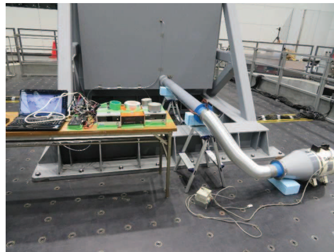
図8 BOP閉止装置気密性能試験状況
