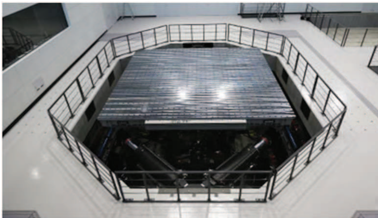
参考図2-3 三次元振動台の概要図
