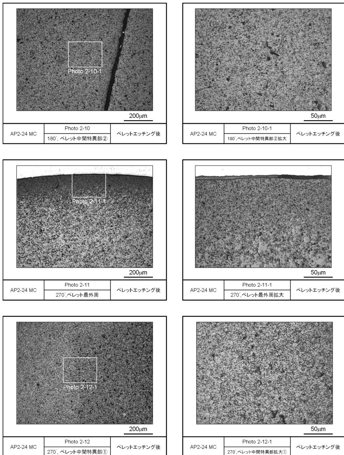
図 4.2.4-2(5) レファレンス試料の金相写真 (ペレットエッチング後, AP2-24 MC)
