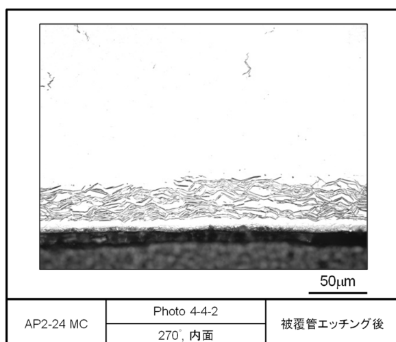
図 4.2.4-4(3) レファレンス試料の金相写真 (被覆管エッチング後, AP2-24 MC)
