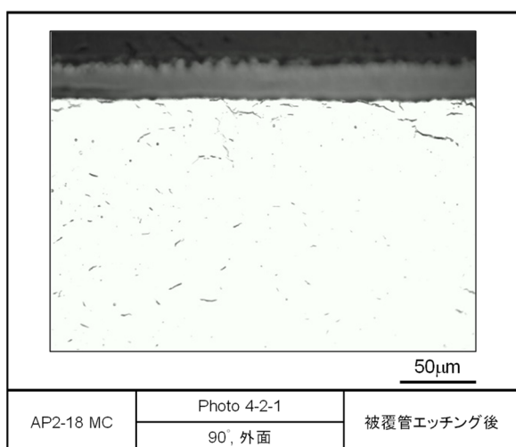
図 4.2.3-4(2) レファレンス試料の金相写真 (被覆管エッチング後, AP2-18 MC)
