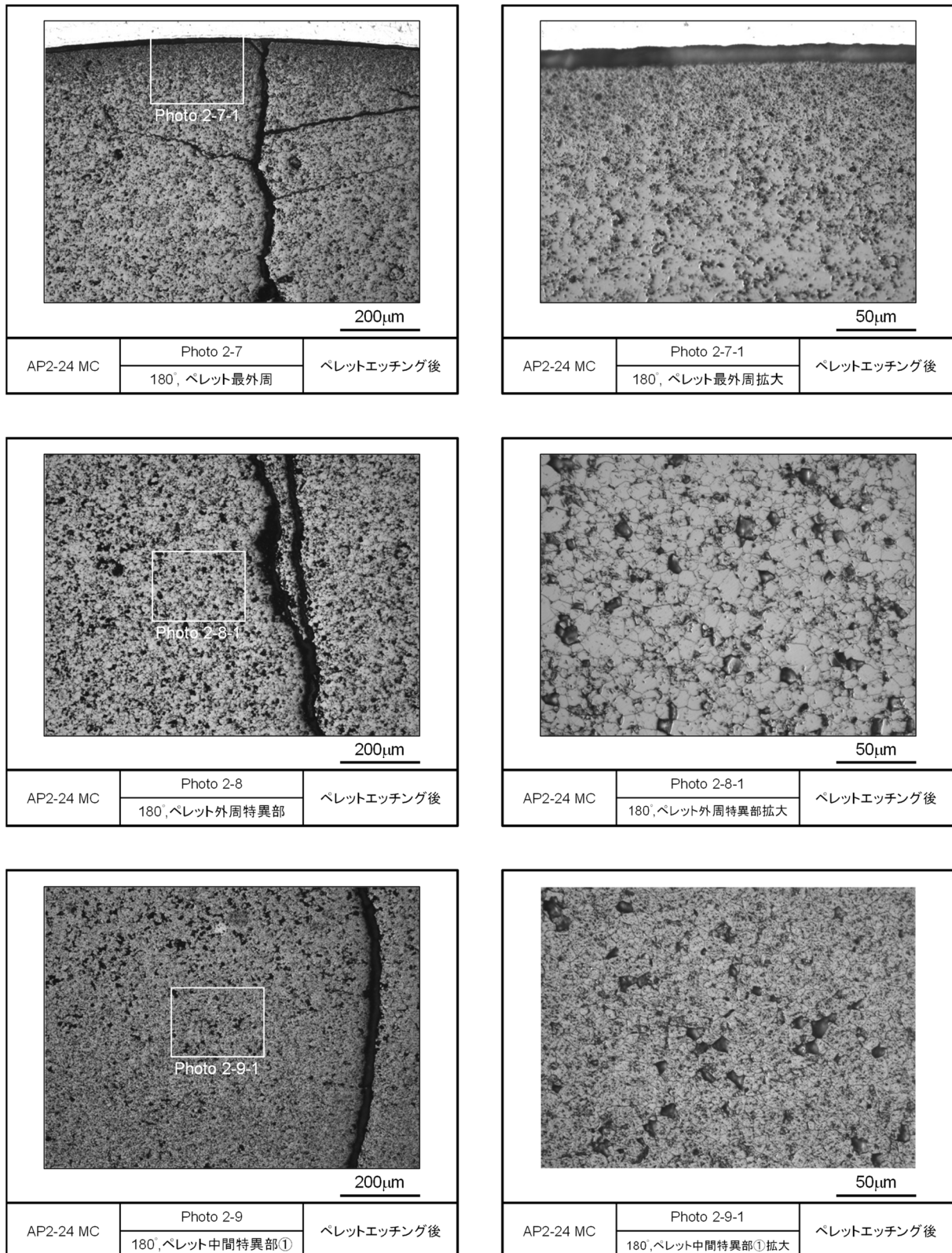
図 4.2.4-2(4) レファレンス試料の金相写真 (ペレットエッチング後, AP2-24 MC)
