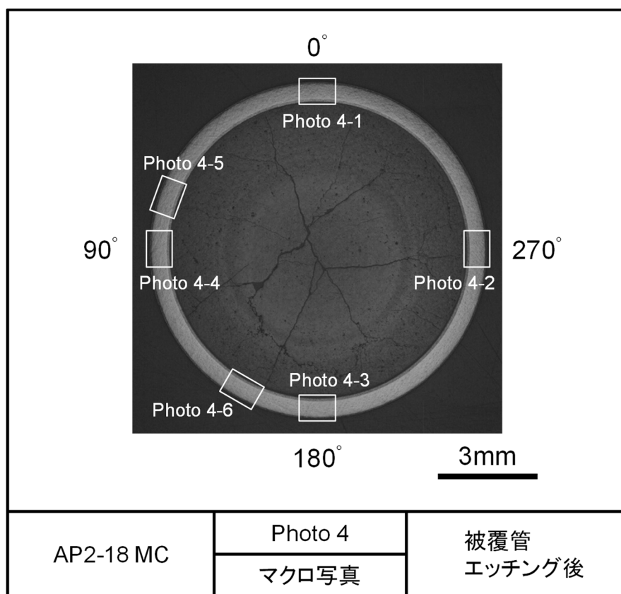
図 4.2.3-4(1) レファレンス試料の金相写真（被覆管エッチング後，AP2-18 MC）
