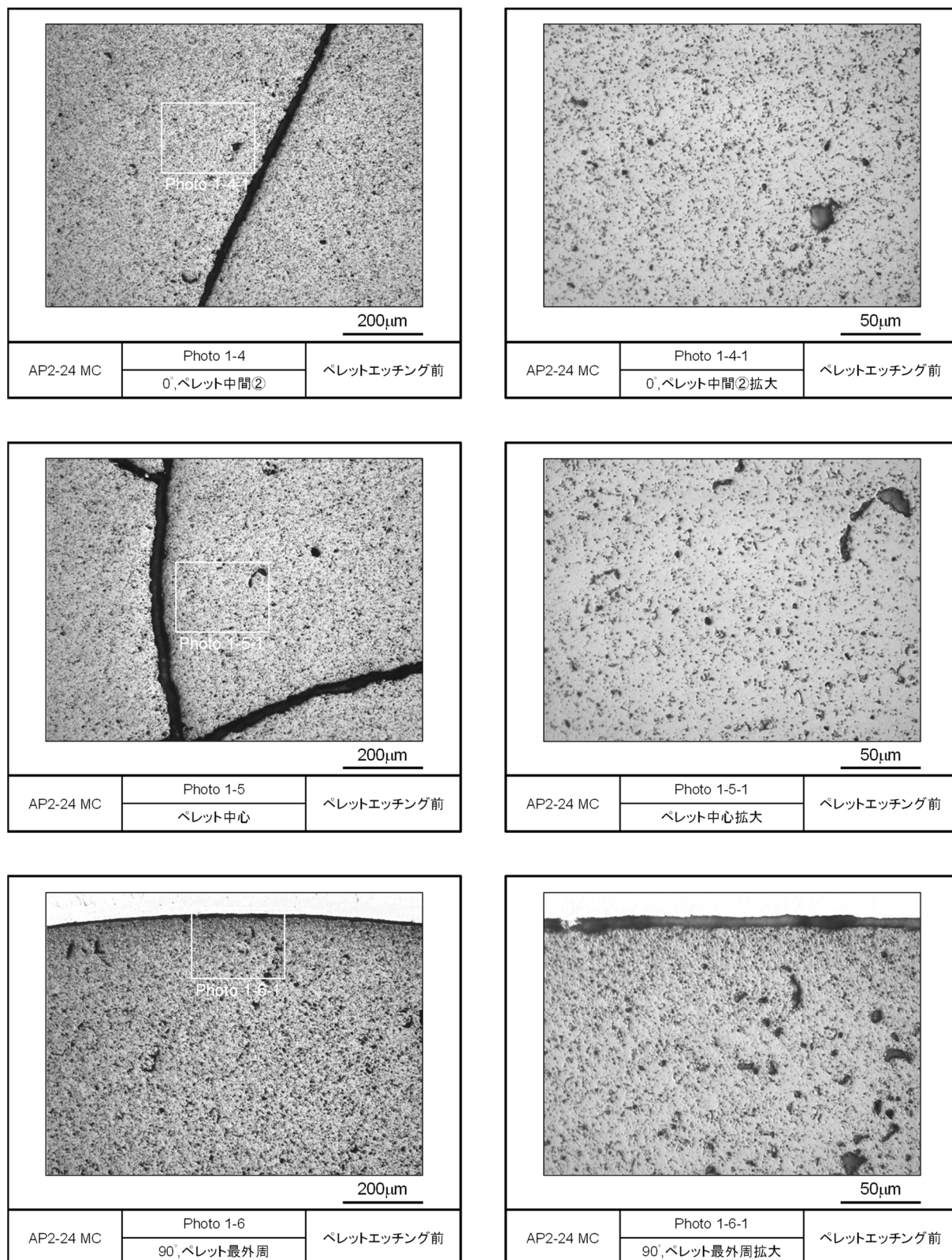
図 4.2.4-1(3) レファレンス試料の金相写真 (ペレットエッチング前, AP2-24 MC)
