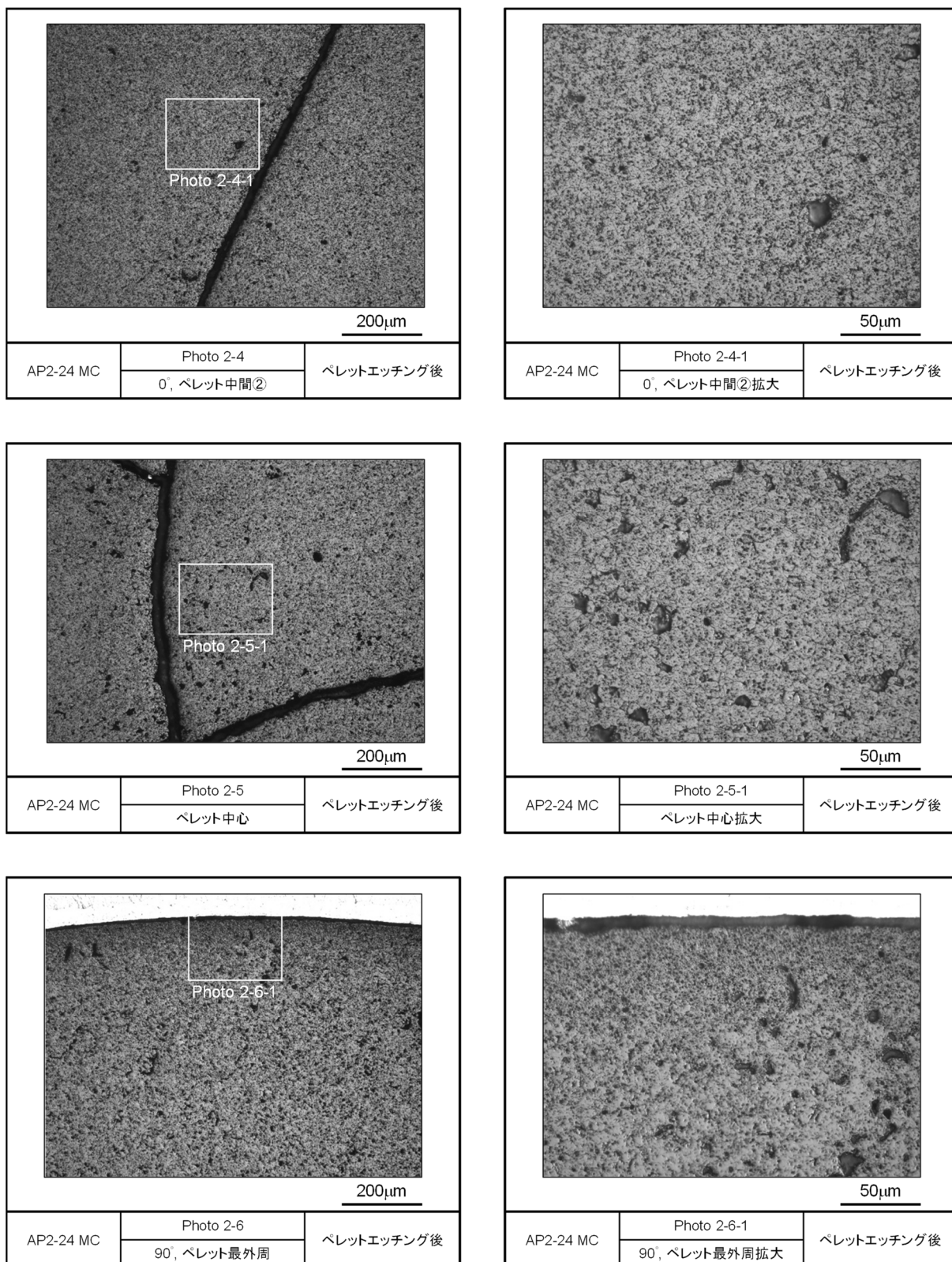
図 4.2.4-2(3) レファレンス試料の金相写真 (ペレットエッチング後, AP2-24 MC)
