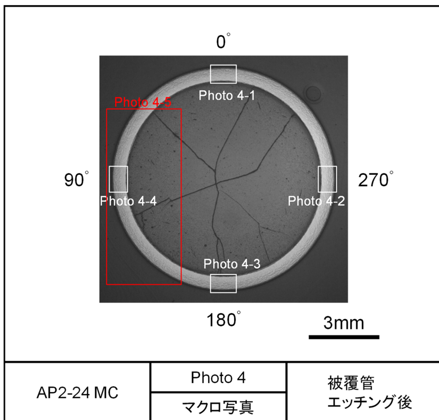
図 4.2.4-4(1) レファレンス試料の金相写真（被覆管エッチング後，AP2-24 MC）
