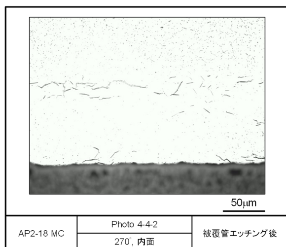
図 4.2.3-4(3) レファレンス試料の金相写真 (被覆管エッチング後, AP2-18 MC)
