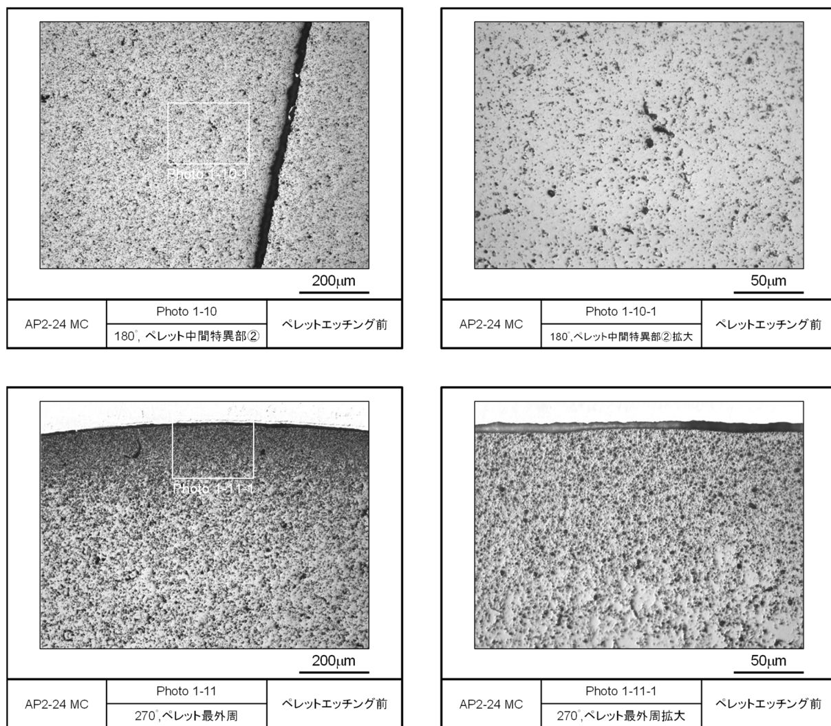
図 4.2.4-1(5) レファレンス試料の金相写真 (ペレットエッチング前, AP2-24 MC)
