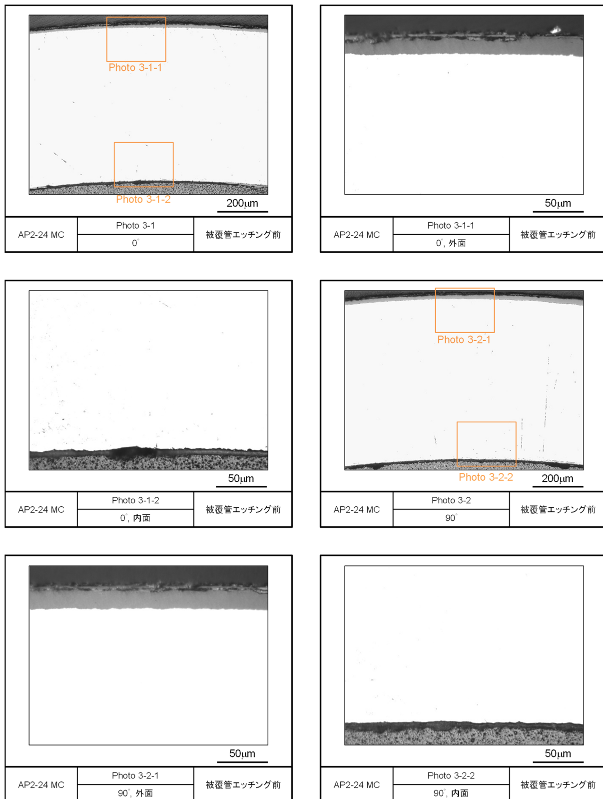
図 4.2.4-3(2) レファレンス試料の金相写真 (被覆管エッチング前, AP2-24 MC)
