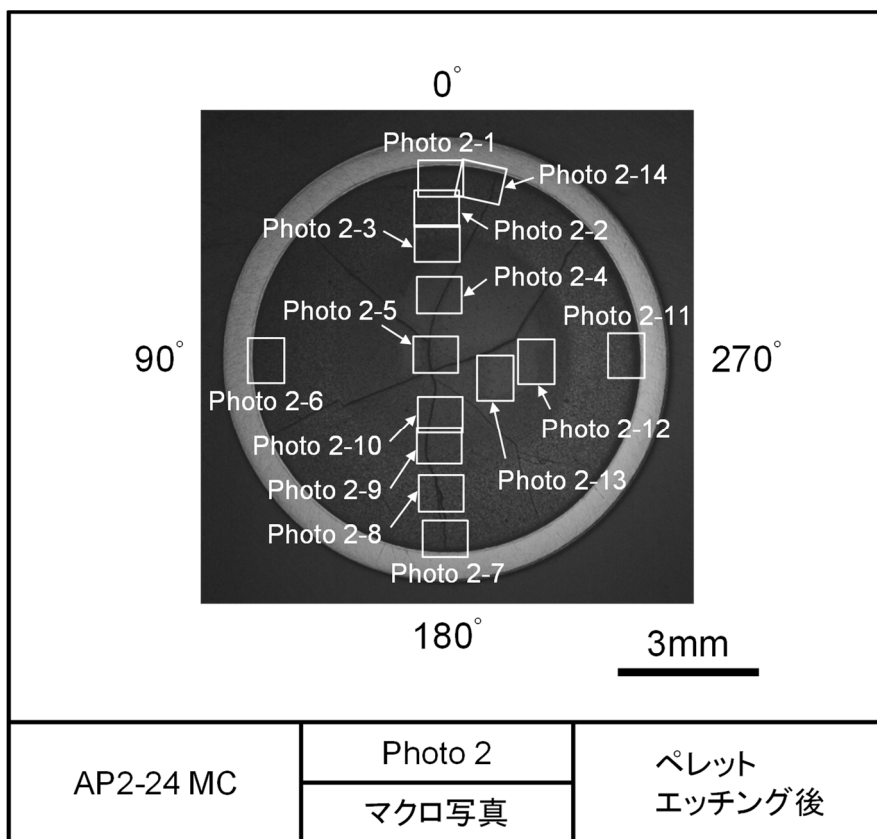
図 4.2.4-2(1) レファレンス試料の金相写真 (ペレットエッチング後, AP2-24 MC)
