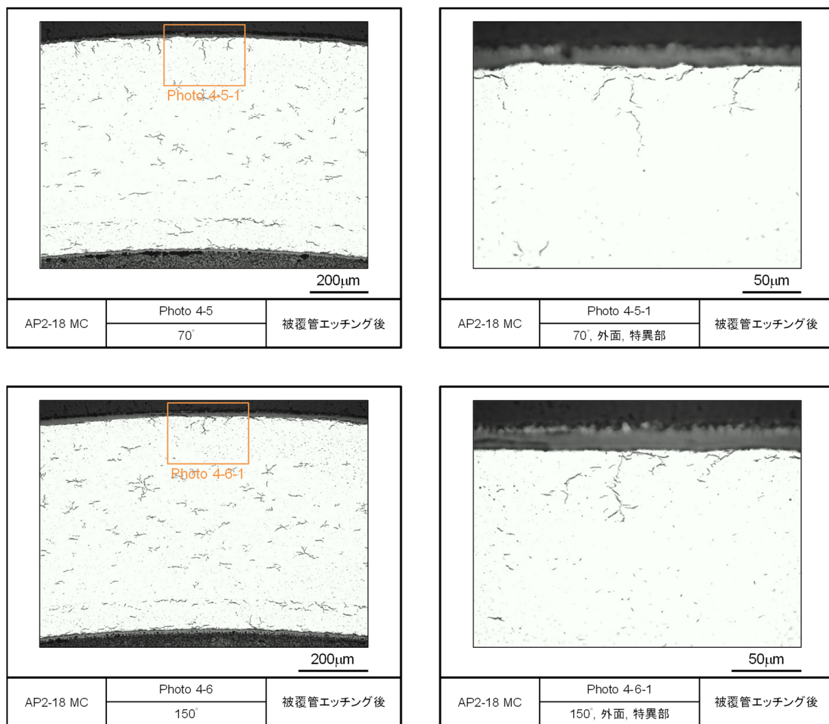
図 4.2.3-4(4) レファレンス試料の金相写真 (被覆管エッチング後, AP2-18 MC)
