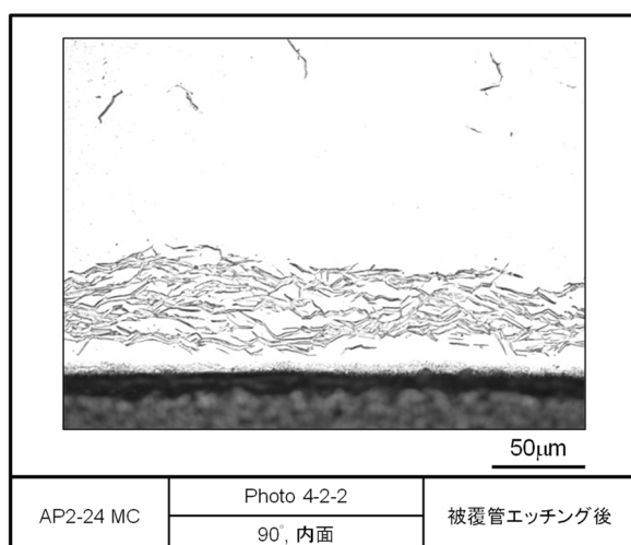
図 4.2.4-4(2) レファレンス試料の金相写真 (被覆管エッチング後, AP2-24 MC)
