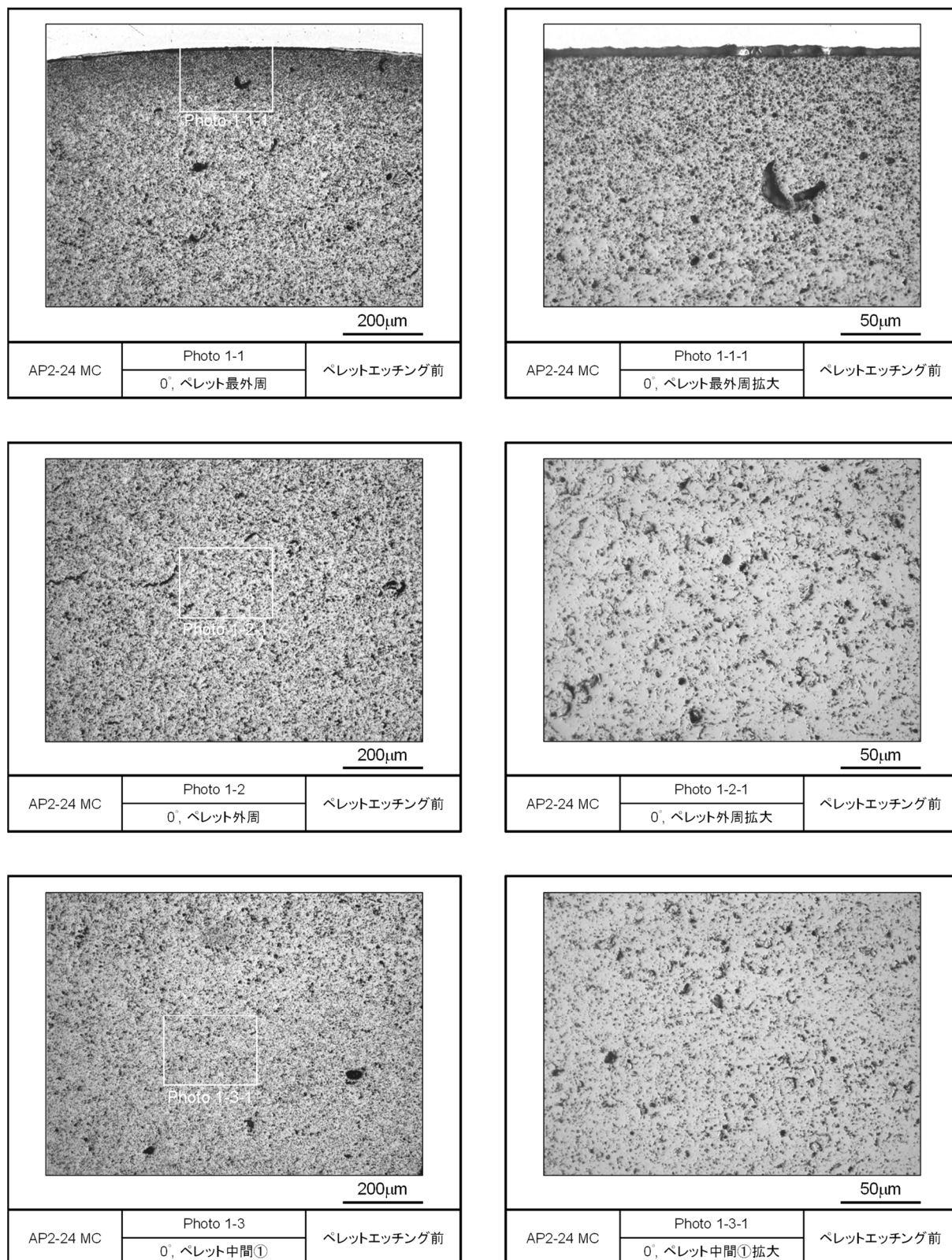
図 4.2.4-1(2) レファレンス試料の金相写真 (ペレットエッチング前, AP2-24 MC)
