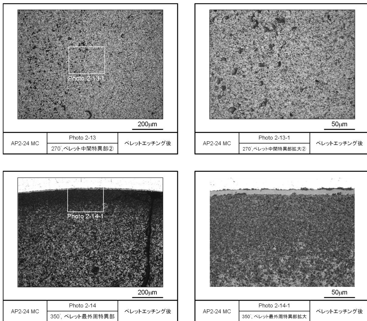
図 4.2.4-2(6) レファレンス試料の金相写真 (ペレットエッチング後, AP2-24 MC)
