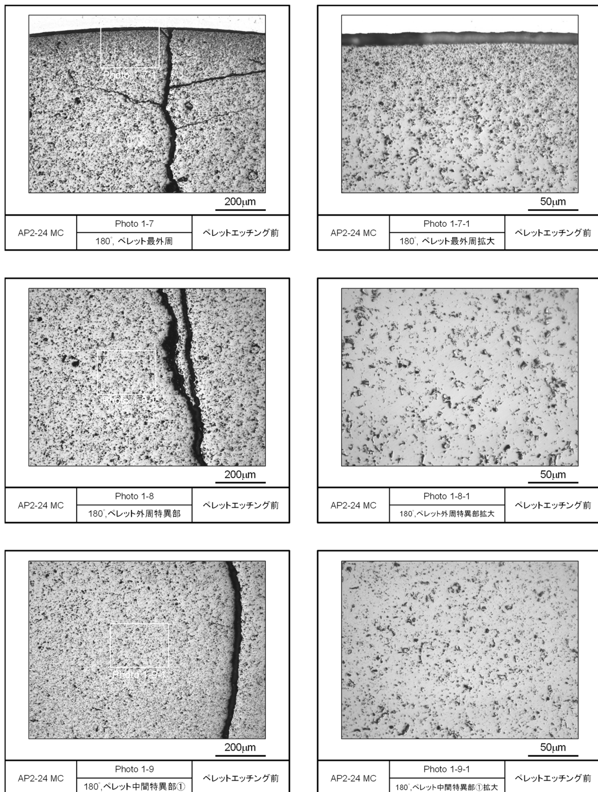
図 4.2.4-1(4) レファレンス試料の金相写真 (ペレットエッチング前, AP2-24 MC)
