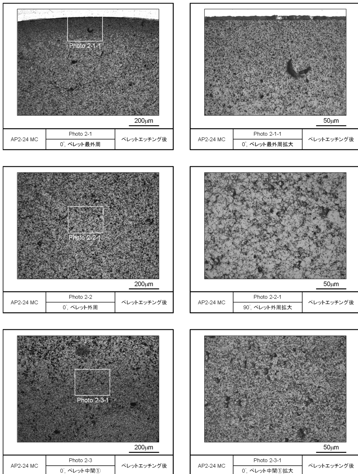
図 4.2.4-2(2) レファレンス試料の金相写真 (ペレットエッチング後, AP2-24 MC)
