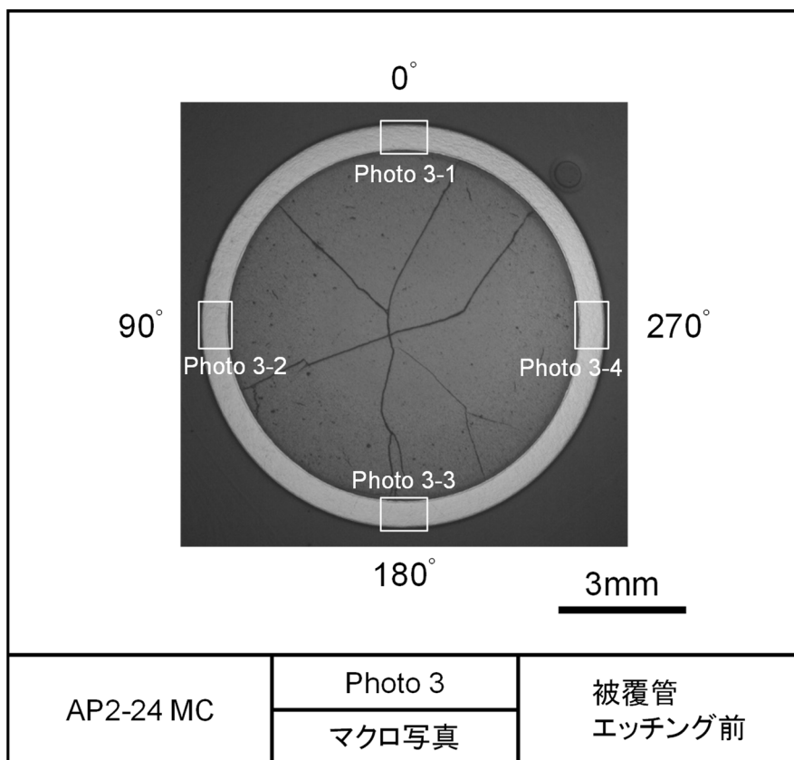
図 4.2.4-3(1) レファレンス試料の金相写真（被覆管エッチング前, AP2-24 MC)
