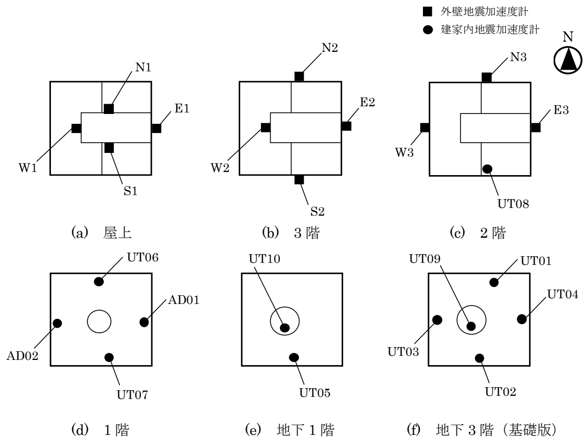
図7 地震計設置位置(平面図)
