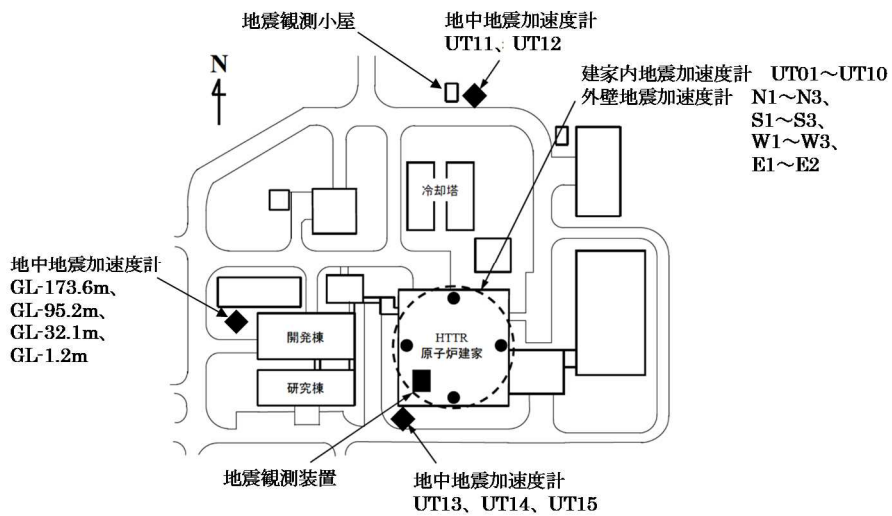
図 6 地震計設置位置 (建家及び地盤)
