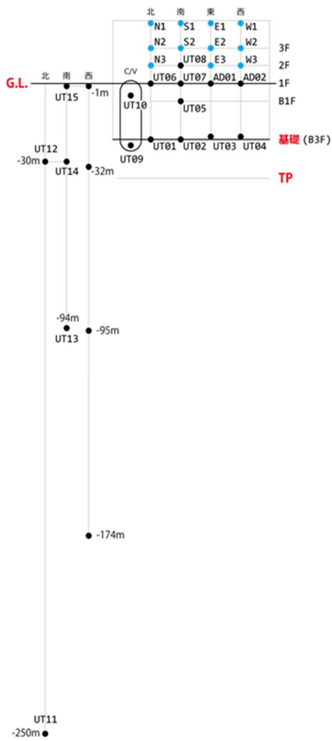
図 5 地震計設置位置 (概略図)
