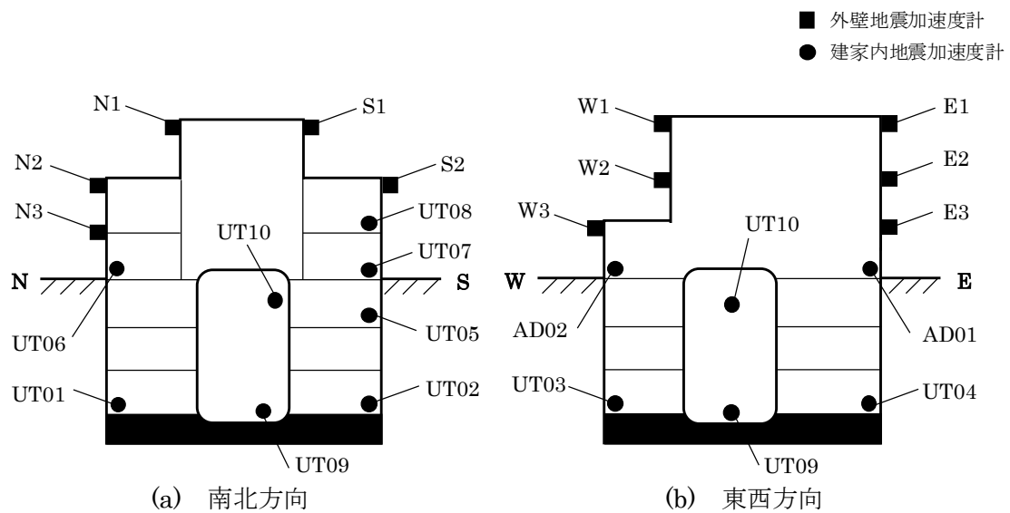
図8 地震計設置位置(立面図)
