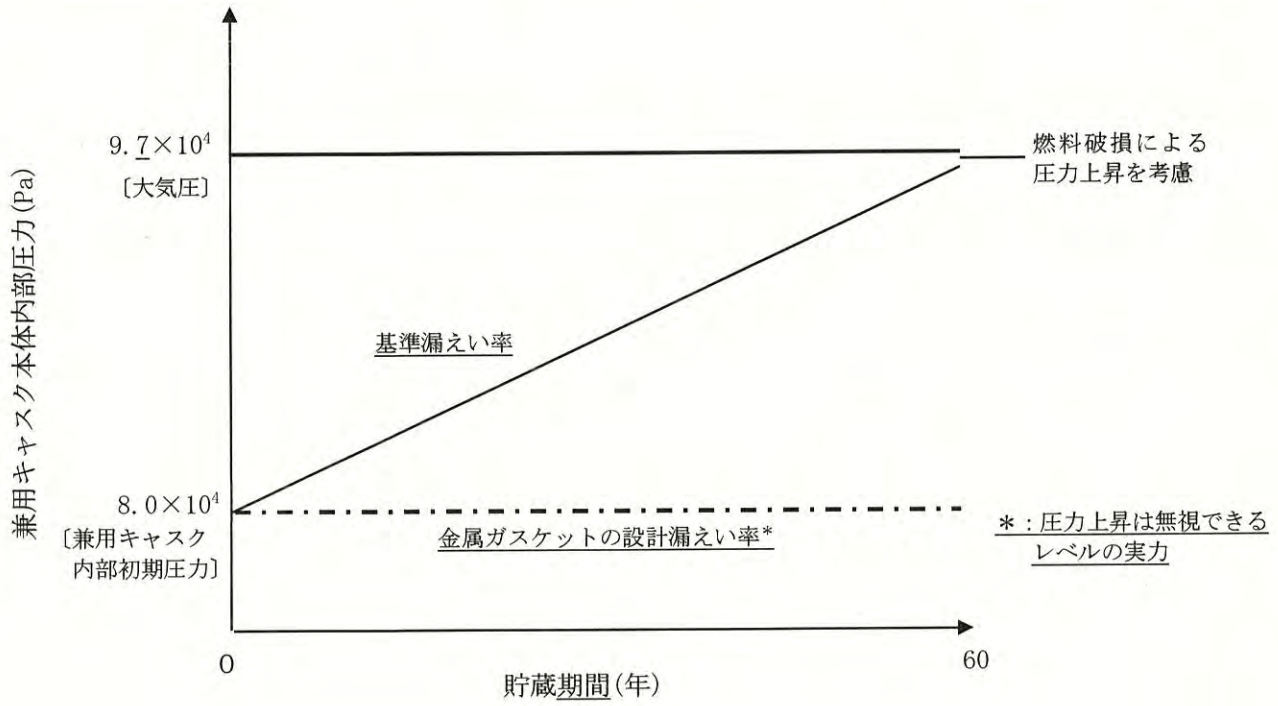
図 2.4.4-5 兼用キヤスクの漏えい率の考え方
