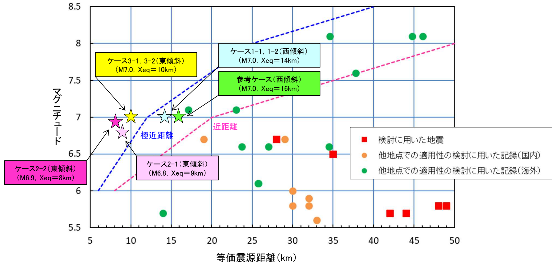
Noda et al.(2002)のデータ範囲と「横浜断層による地震」との関係
