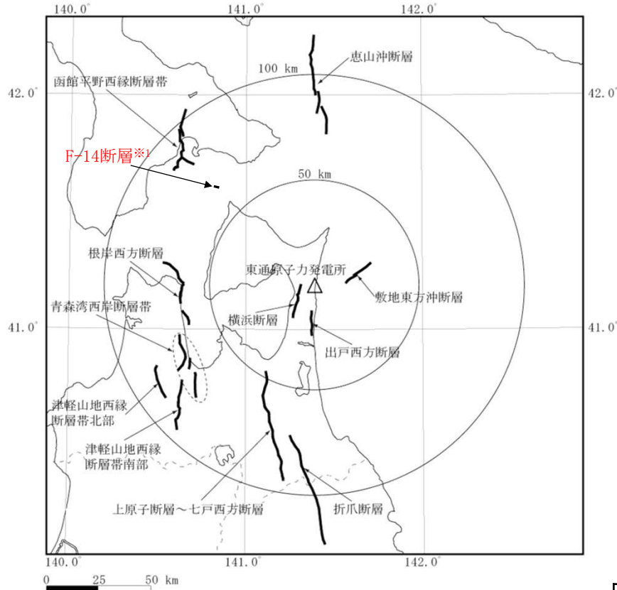
震源として考慮する活断層 配置図
