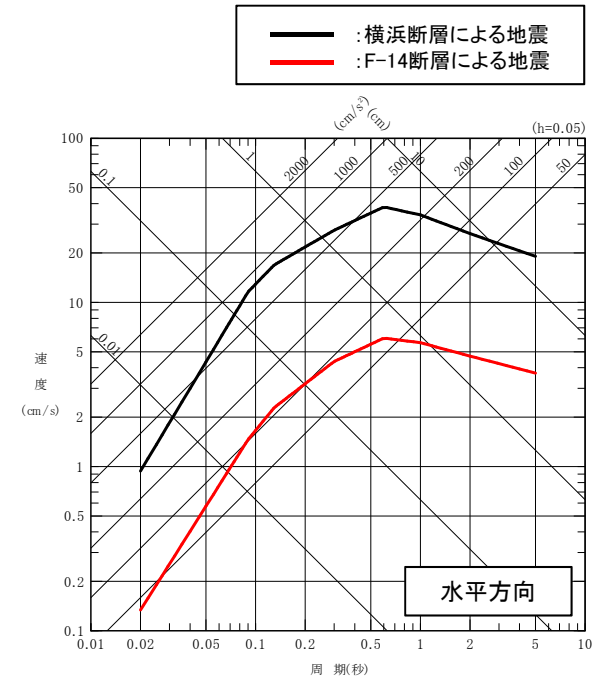
横浜断層による地震とF-14断層による地震の応答スペクトル [Noda et al.(2002)]
